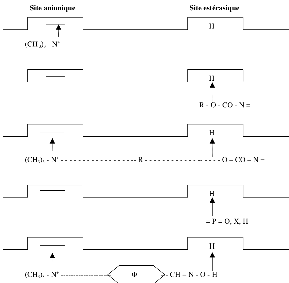
figure 4.8.-1: cholinestérases et anticholinestérasiques - de haut en bas : ammoniums quaternaires, carbamates d'amines tertiaires, carbamates d'ammonium quaternaires, réactivation par le pralidoxime.
