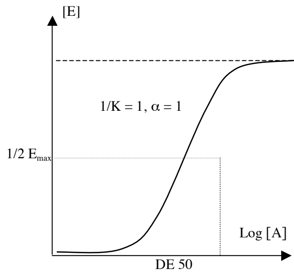
figure 2.1.-5 : courbe doses/effets, coordonnées semi-logarithmiques - Log [A] doses, [E] intensité de l'effet, [E_{max}] intensité maximale de l'effet, DE 50 dose efficace 50 ou puissance = CE 50 concentration efficace 50, 1/K affinité, \alpha efficacité.
