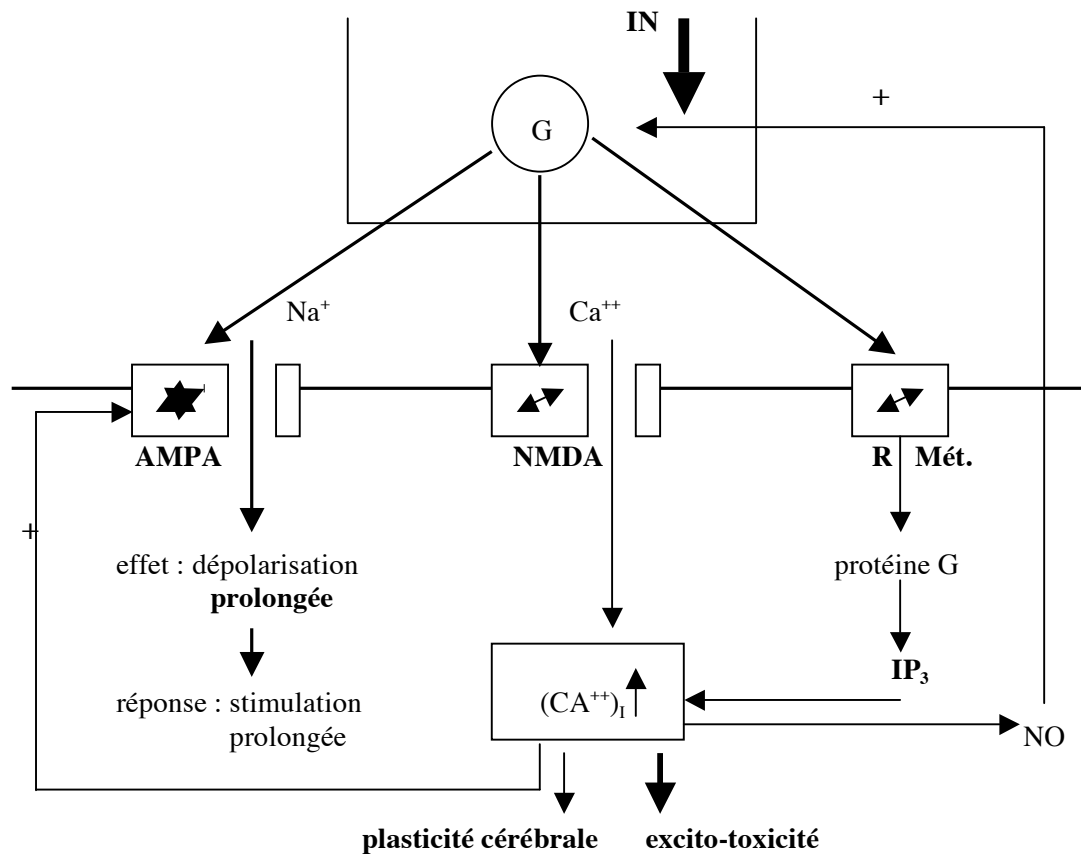
figure 3.7.-9 : synapse glutaminergique (fonctionnement prolongé, excito-toxicité) - G acide glutamique, Na + ions sodium, Ca ++ ions calcium, NO oxyde nitrique, IP 3 inositol triphosphate (second messenger), AMPA, NMDA, R Mét. récepteurs glutaminergiques, (Ca ++ ) i ions calcium libres intracellulaires.
