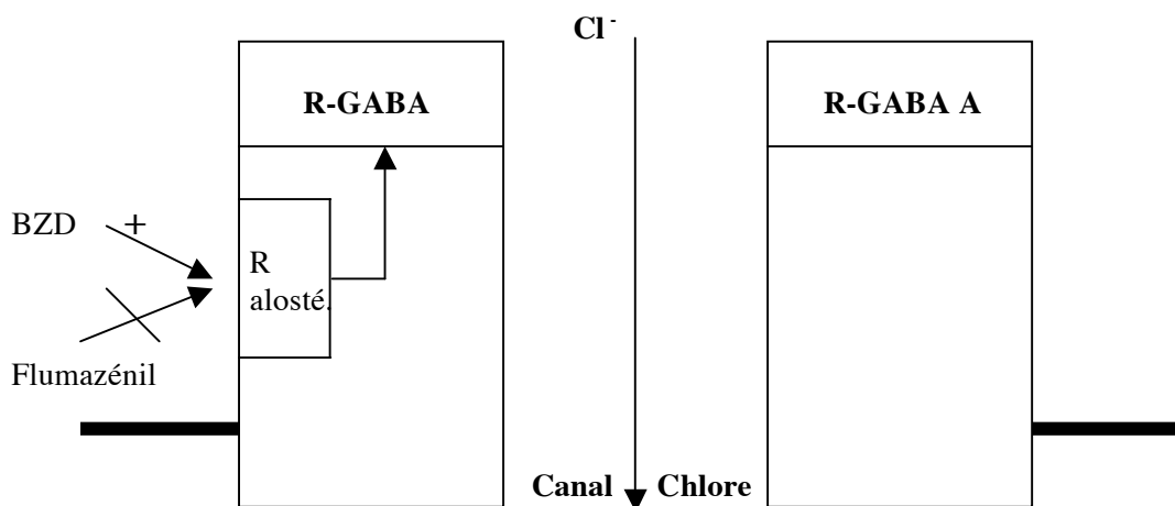
figure 4.16.-1: le récepteur GABA-A et son site allostérique - BZD benzodiazépines, R alosté. récepteur allostérique, R-GABA A récepteur gaba-ergique A.
