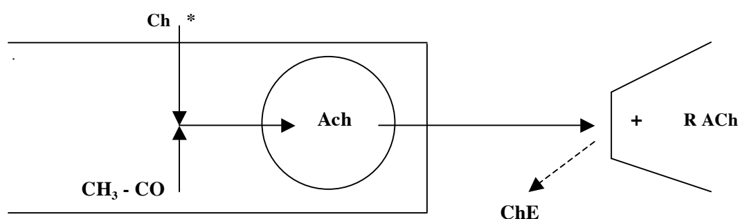
figure 3.3-1 : synapse cholinergique - Ch choline, CH 3 -CO radical acétyl, Ach acétylcholine, ChE cholinestérases, R ACh récepteur de l'acétylcholine, * transport actif.
