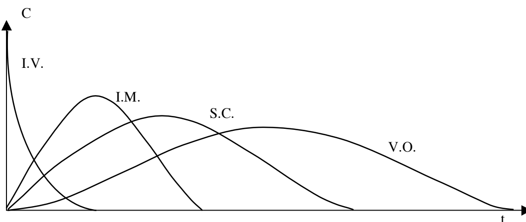
figure 1.6-4 : administration unique, diverses voies, concentrations plasmatiques.
