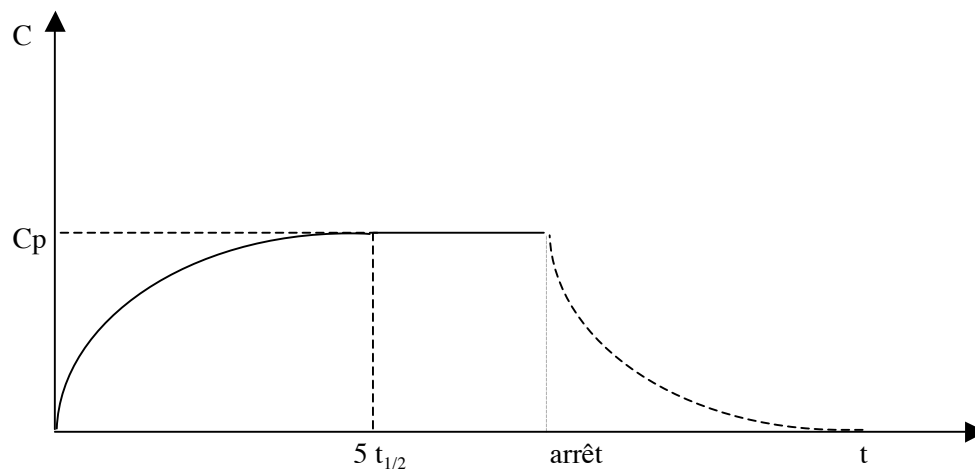
figure 1.6-5 : administration continue (perfusion) - C_p concentration à l'équilibre (plateau), t_{1/2} demi-vie plasmatique d'élimination. I vitesse de perfusion. Cl_T clairance corporelle totale.
