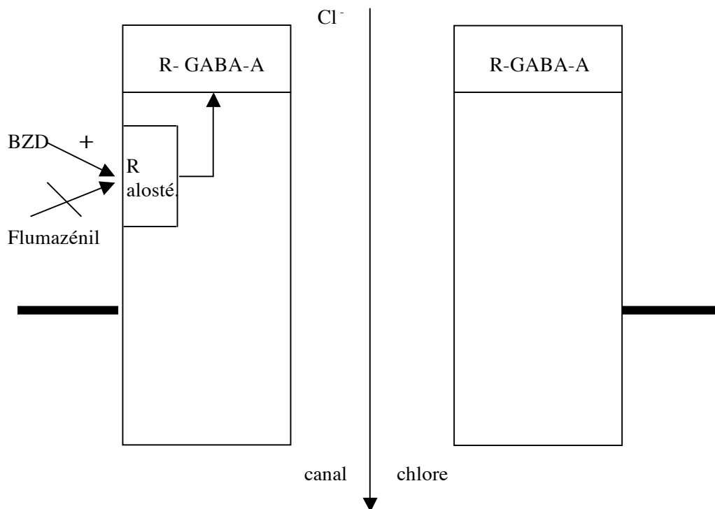
Figure 3.7.-4 : récepteur GABA-A - BZD benzodiazépines, R alosté. Récepteur alostérique, R-GABA A récepteur gaba-ergique A.
