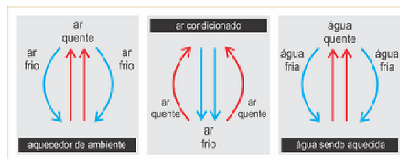
Convecção térmica
