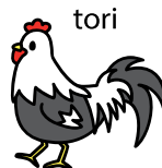
tori
