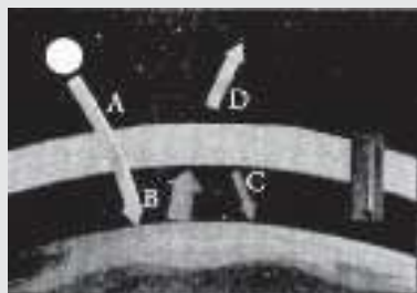
Efecto invernadero
