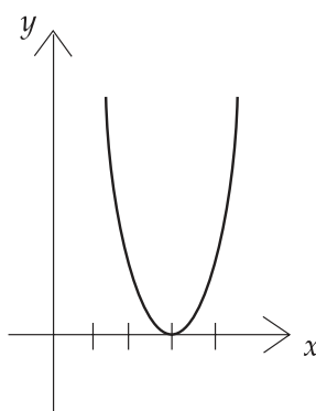
Solución única y = x^2 - 6x + 9
