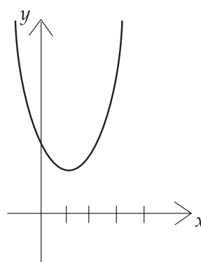
Soluciones imaginarias y = x^2 + 2x + 3
