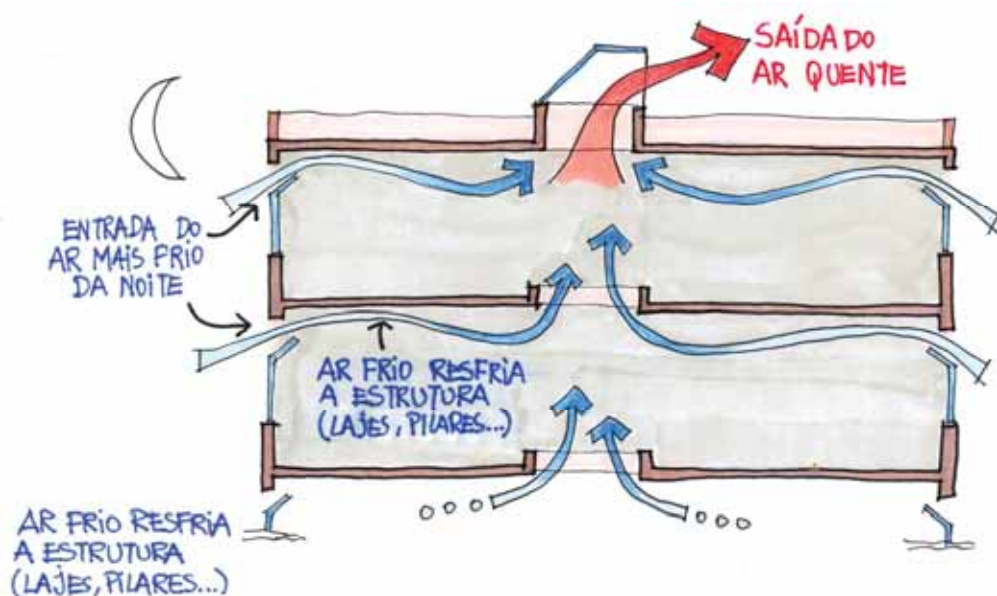
Figura 6-20: Ventilação noturna
