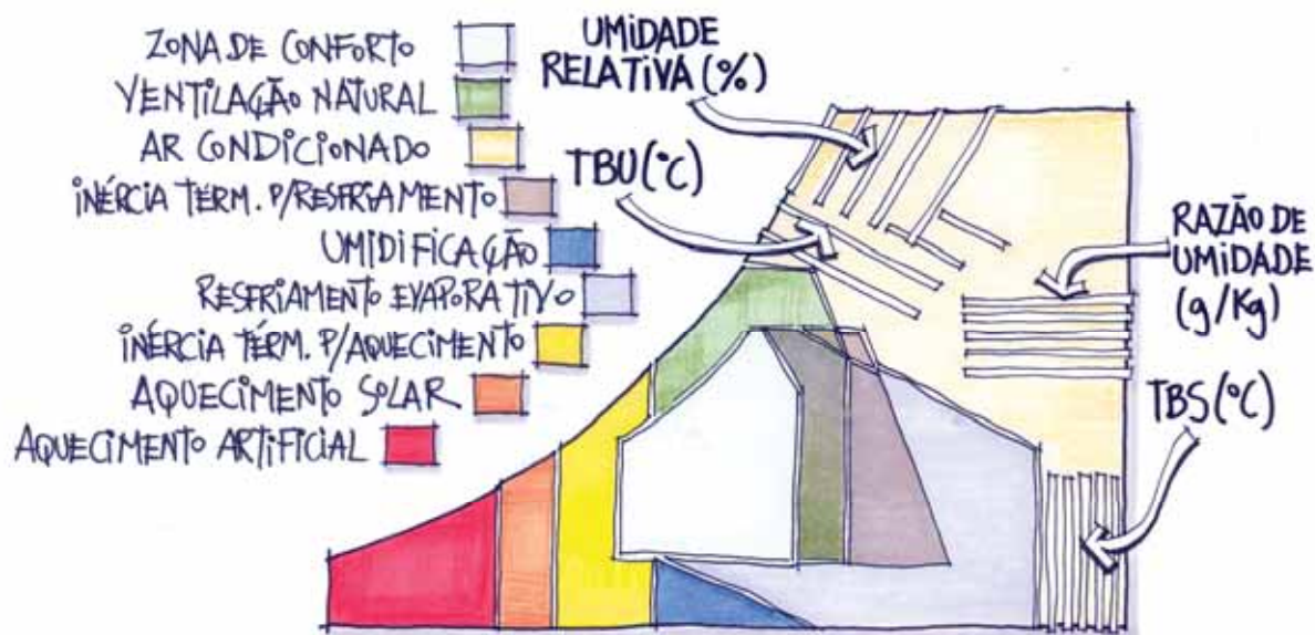
Figura 3-18: Carta Bioclimática adotada para o Brasil
