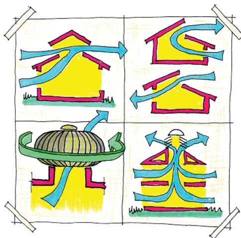
Figura 9-11: Ventilação vertical
