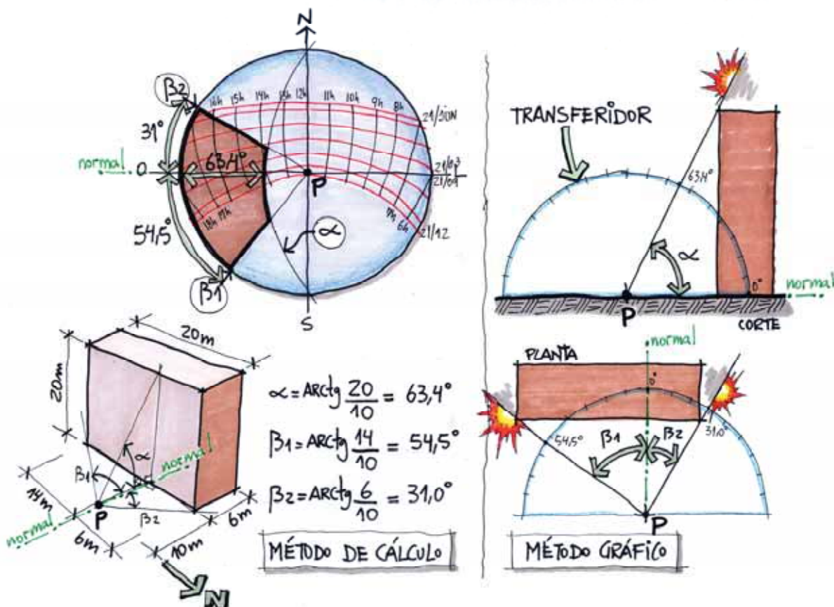
Figura 4-23: Máscara de sombreamento de um edifício para um ponto "P" sobreposta à carta solar
