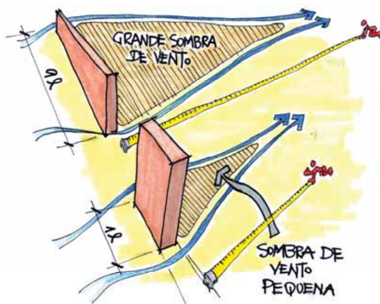
Figura 6-8: Sombra de vento em função da largura da barreira
