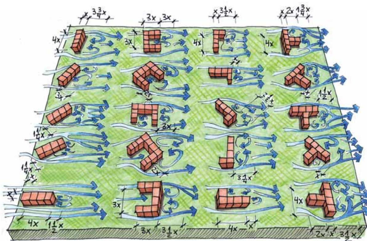
Figura 6-10: Fluxo de ventos ao redor das edificações
