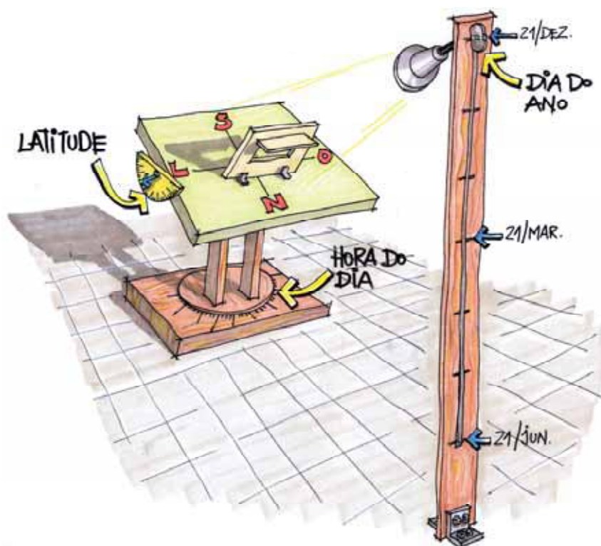
Figura 4-38: Heliodon
