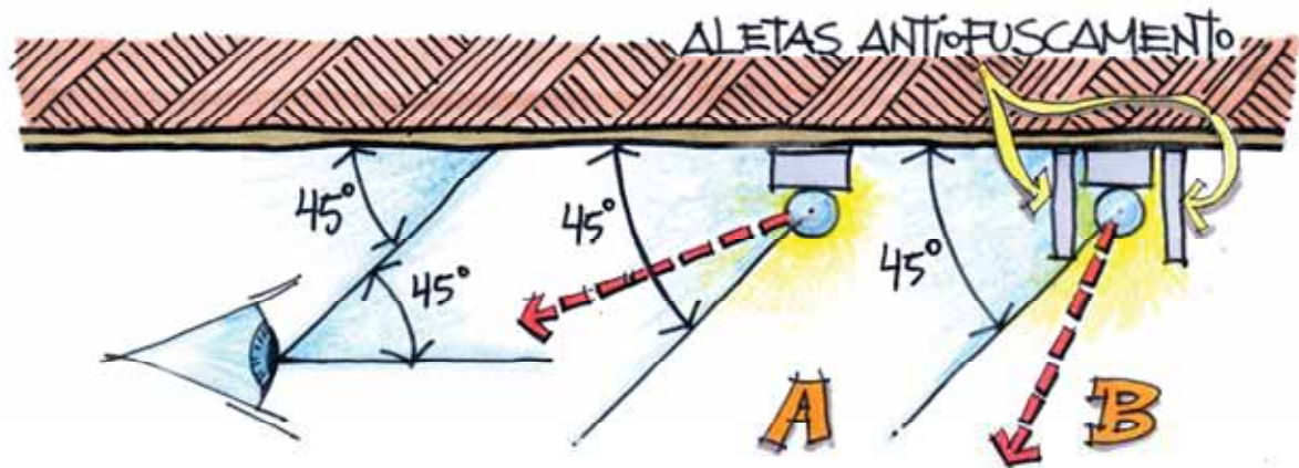
Figura 2-23: Zona de ofuscamento direto
