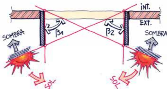
Figura 4-28: Proteção solar vertical - ângulo \beta e sombreamento
