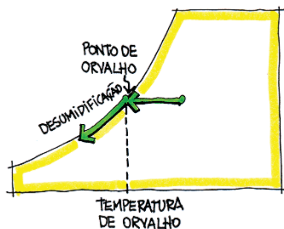
Figura 11-11: Desumidificação
