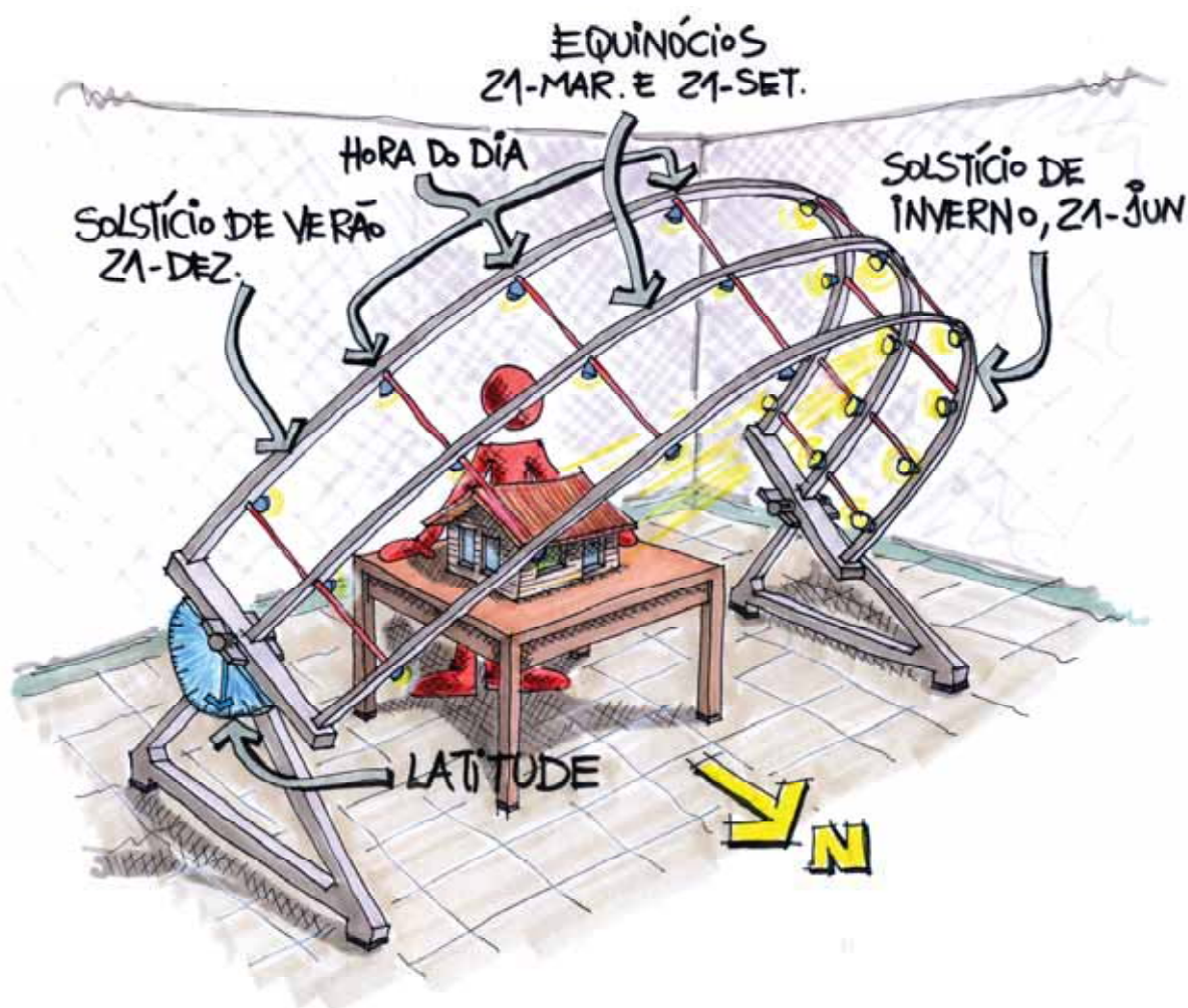
Figura 4-39: Solarscópio
