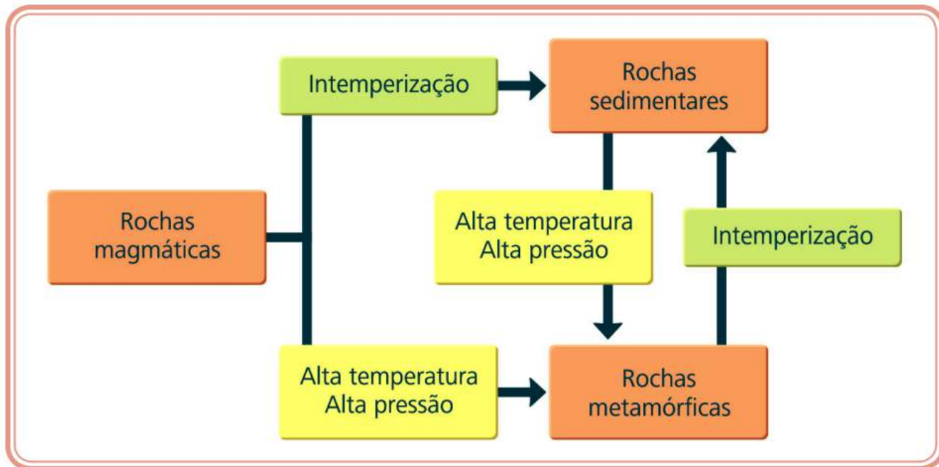
Figura 2.5: Dinâmica das rochas
