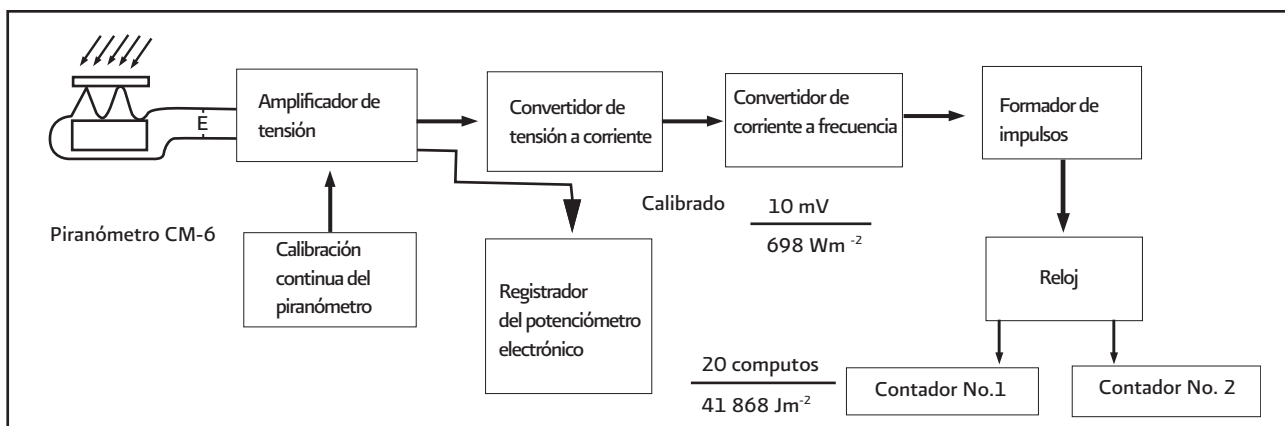
Figura 6.7 Diagrama de bloques de un integrador electrónico (CC-1)
