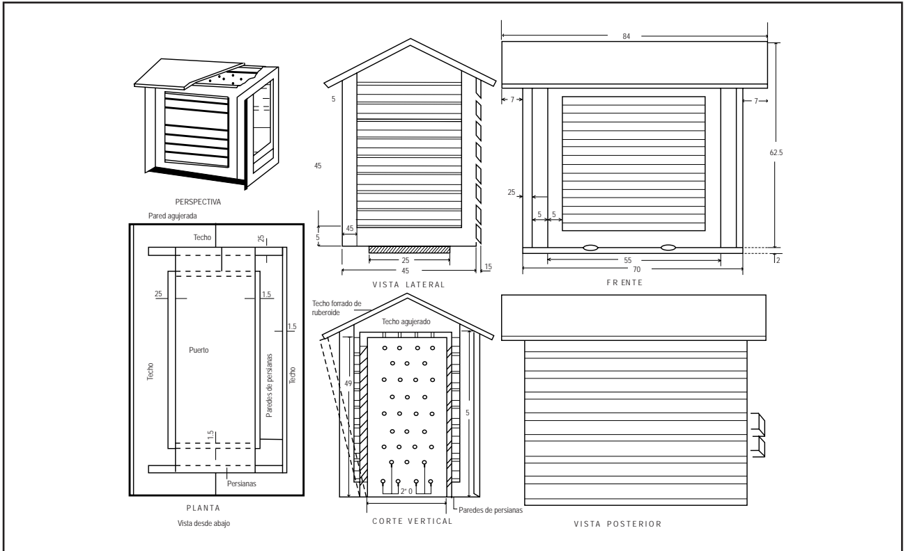
Figura 13.2 Detalles de la caseta o abrigo meteorológico
