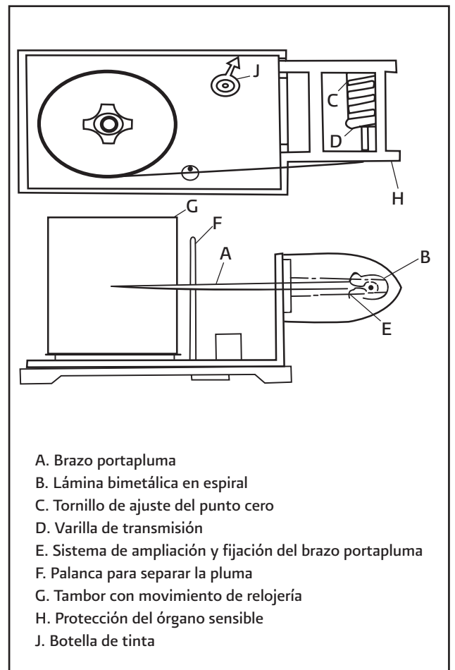
Figura 1.4 Elementos del termógrafo de lámina bimetálica
