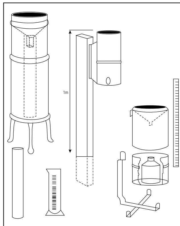
Figura 5.4 Pluviómetro de Hellman (a) y de Reglilla (B)
