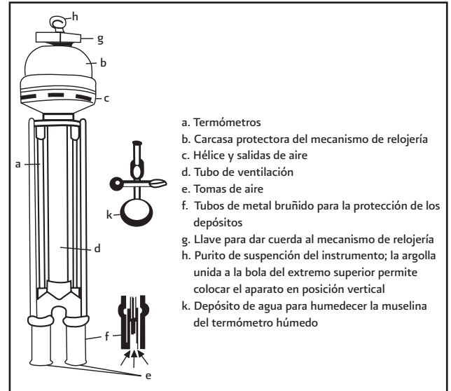
Figura 3.2 Psicrómetro tipo Assman
