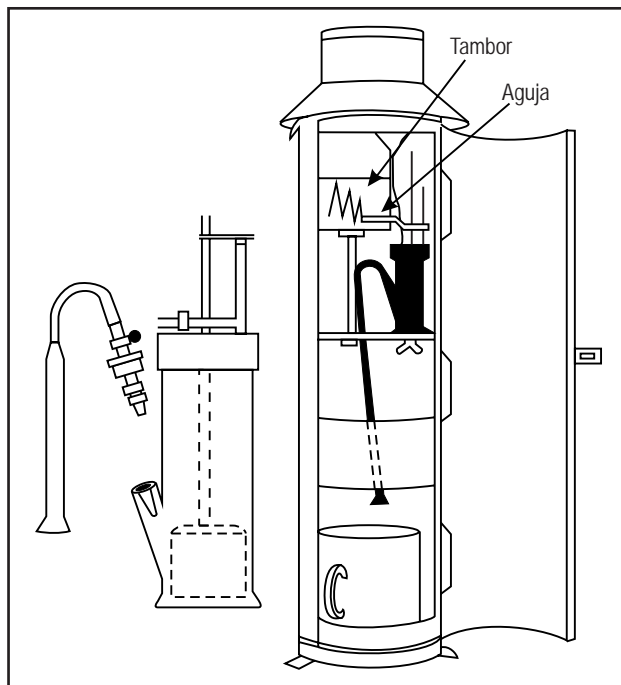
Figura 5.5 Pluviógrafo
