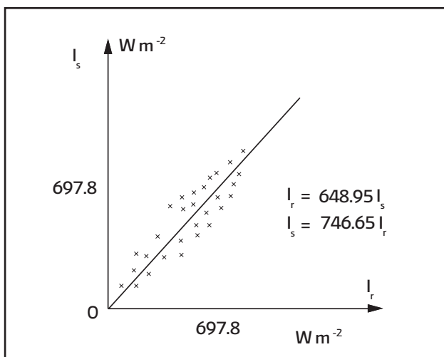
Figura 6.9 Gráfico de I_s en función de I_r para propósitos de calibración.
