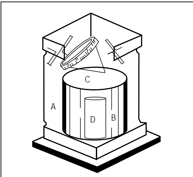
Figura 5.2 Pluviómetro con sus diferentes componentes
