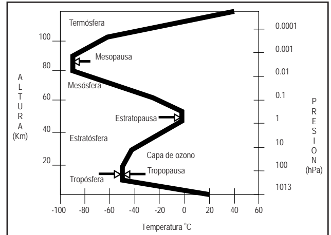
Figura 12.1 Capas de la atmósfera
