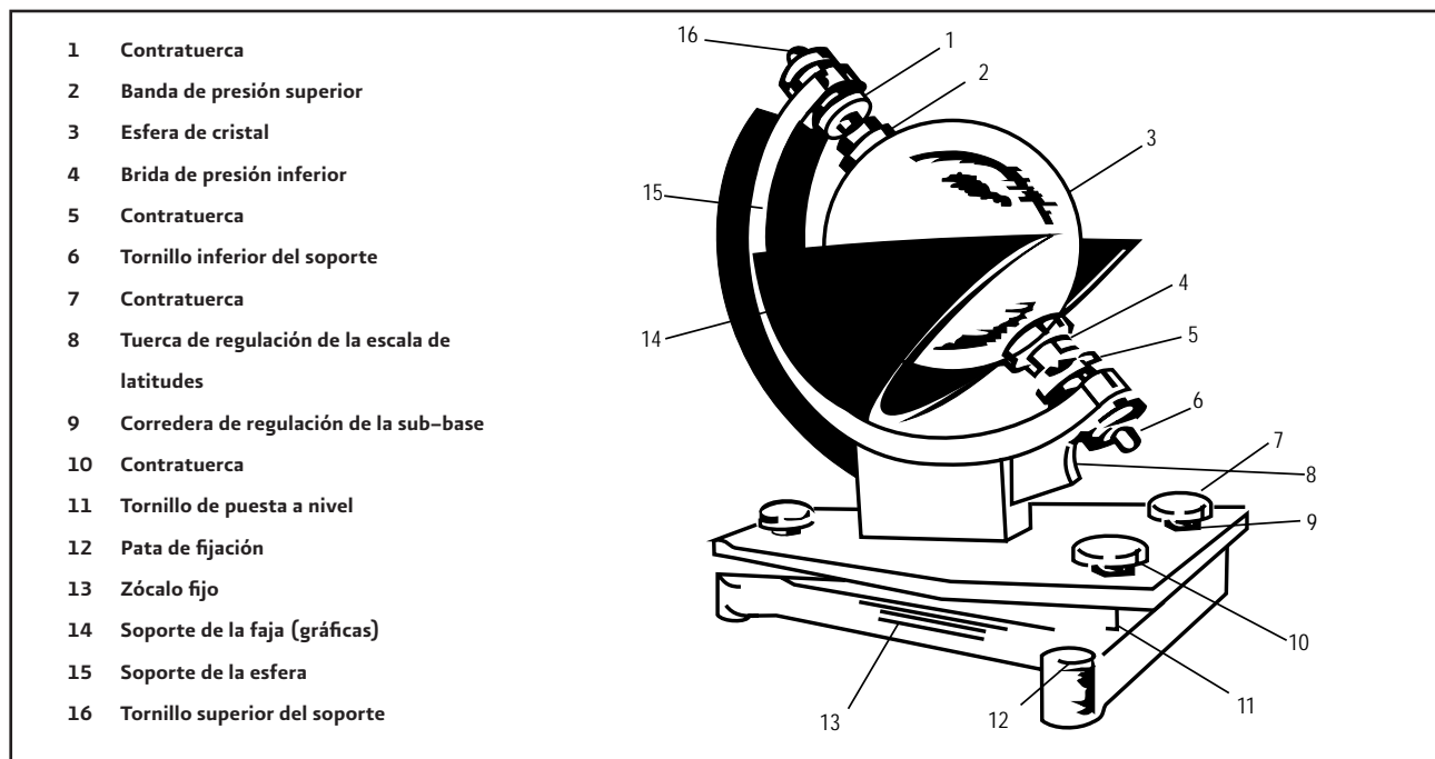
Figura 7.1 Heliofanógrafo de Campbell-Stokes
