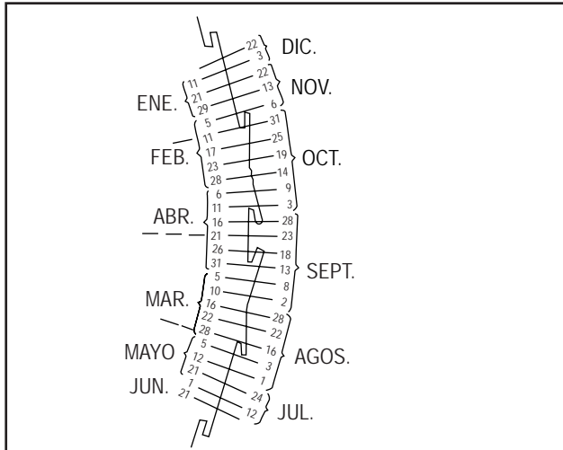
Figura 7.3 Sección del soporte del heliofanógrafo y calendario de utilización de esos diagramas.
