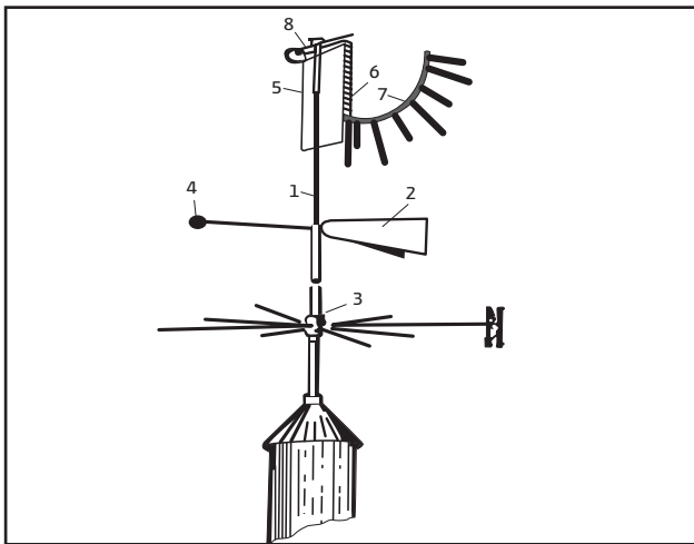
Figura 4.3 Anemómetro de placa.
