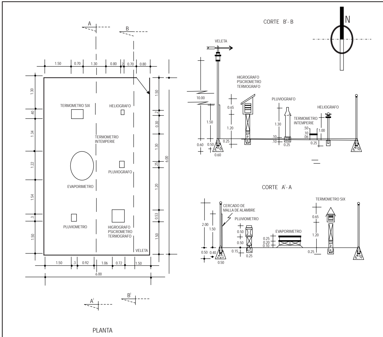
Figura 13.3 Orientación y ubicación de los instrumentos y equipo de medición
