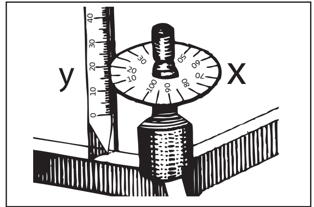
Figura 9.4 Lectura de la escala del tornillo micrométrico
