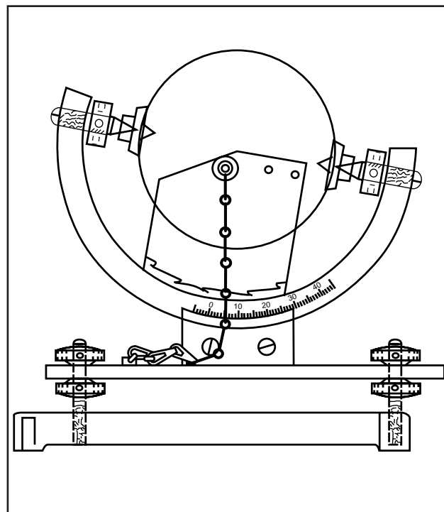
Figura 7.2 Modelo tropical de heliofanógrafo.
