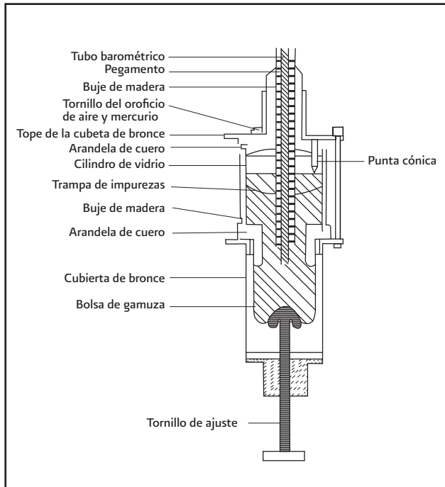
Figura 2.2 Cubeta del barómetro de Fortín
