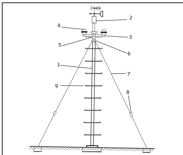
Figura 4.2 Mástil anemométrico.
