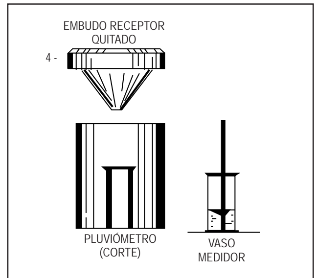
Figura 5.3 Pluviómetro con sus partes más indispensables
