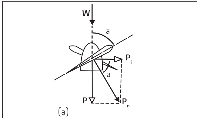
Figura 4.8 Los parámetros del sensor de hélice.
