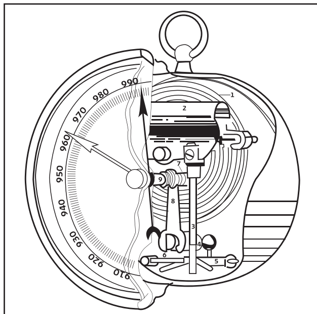
Figura 2.6 Mecanismo típico de un barómetro aneroide
