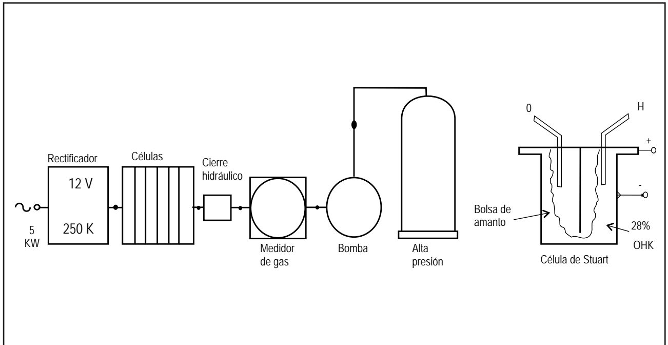
Figura 12.5 Esquema funcional del generador de hidrógeno electrolítico
