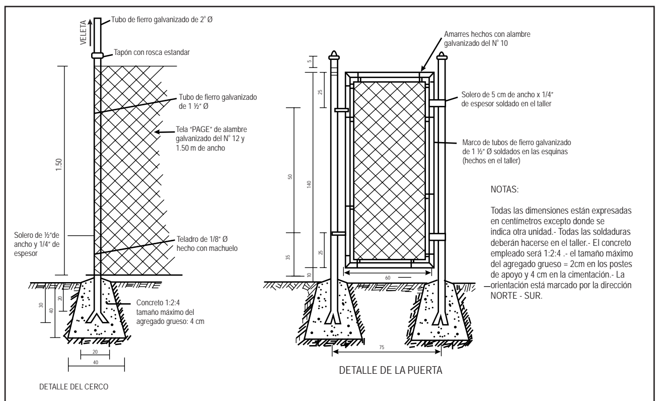
Figura 13.1 Detalle constructivo del cerco
