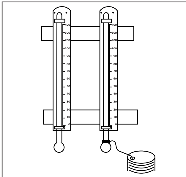
Figura 3.1 Psicrómetro simple sin ventilación artificial
