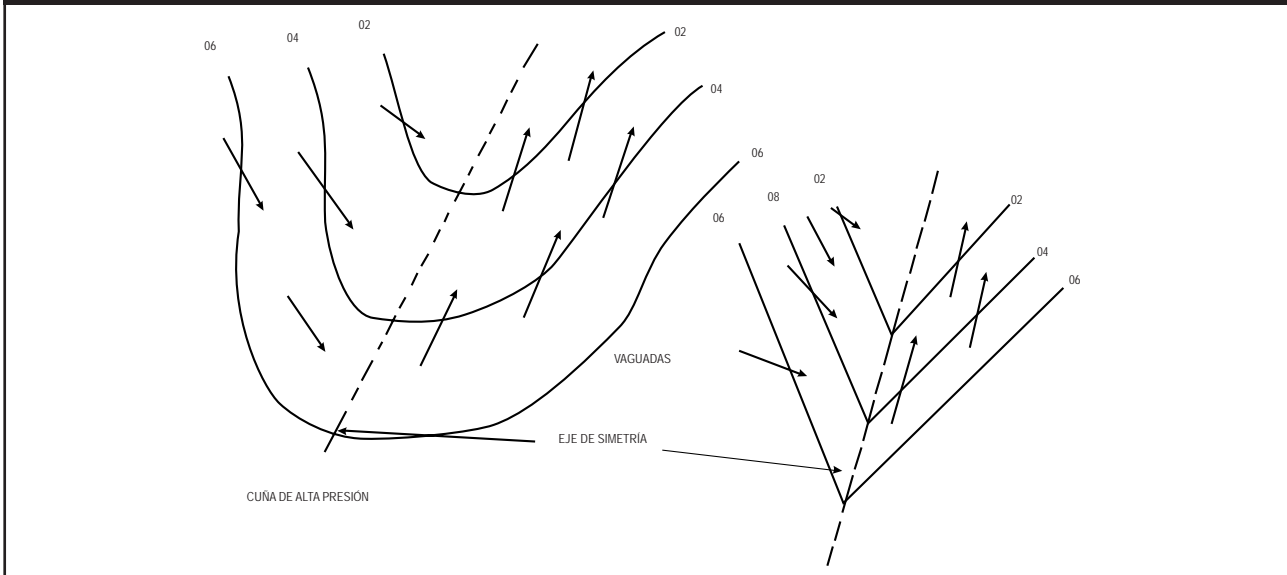
Fig. 6 Vaguada
