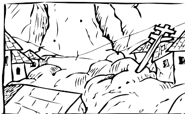
Deslizamientos.
