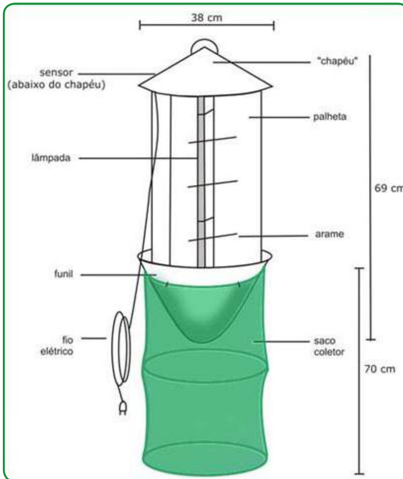
Figura E4 - Modelo de armadilha luminosa comercializada pela empresa BIOCONTROLE.
