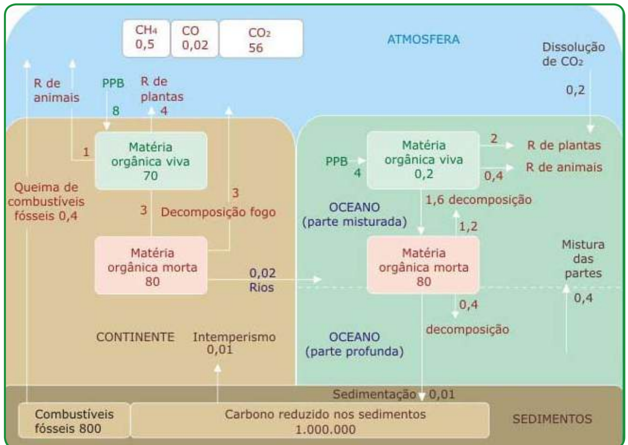
Figura D3 - Ciclo do carbono com seus depósitos e fluxos - Depósitos: 10^5 mol; fluxos: 10^5 mol . ano -1 (Fonte: adaptado de www.ib.usp.br/.../ciclo_bio-geoquimicos_print.htm )
