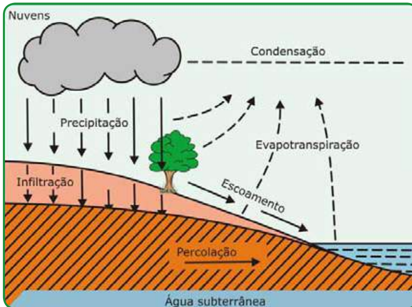
Figura D2 - Ciclo da água. (Fonte: adaptado de http://www.geofisica.com.br/cicloa.gif )
