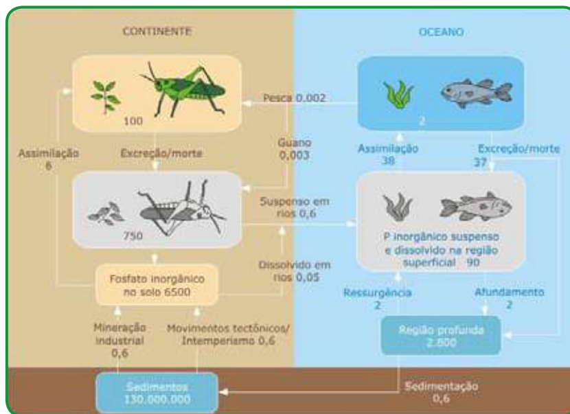
Figura D5 - Ciclo do fósforo com seus depósitos e fluxos - Depósitos: 10^{12} mol; fluxos: 10^{12} mol . ano -1 (Fonte: adaptado de www.ib.usp.br/.../ciclo_biogeoquimicos_print.htm )
