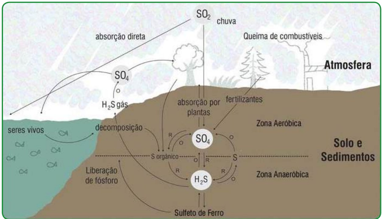
Figura D7 - Ciclo do enxofre. (Fonte: adaptado de Odum, 2004)
