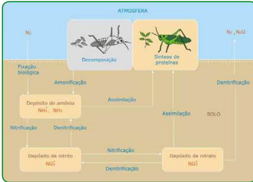
Figura D4 - Ciclo do nitrogênio. (Fonte: adaptado de www.ib.usp.br/.../ciclo_biogequimicos_print.htm )
