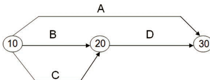
Figura 10.1 Exemplo de uma rede PERT/CPM
