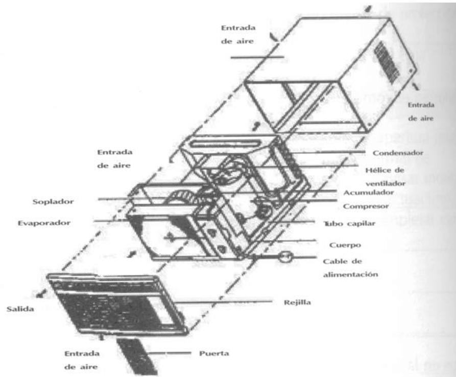
Fig 20: Despiece, componentes mayores de un AA de ventana
