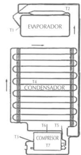
Fig 2: Temperaturas del Circuito de una nevera doméstica
