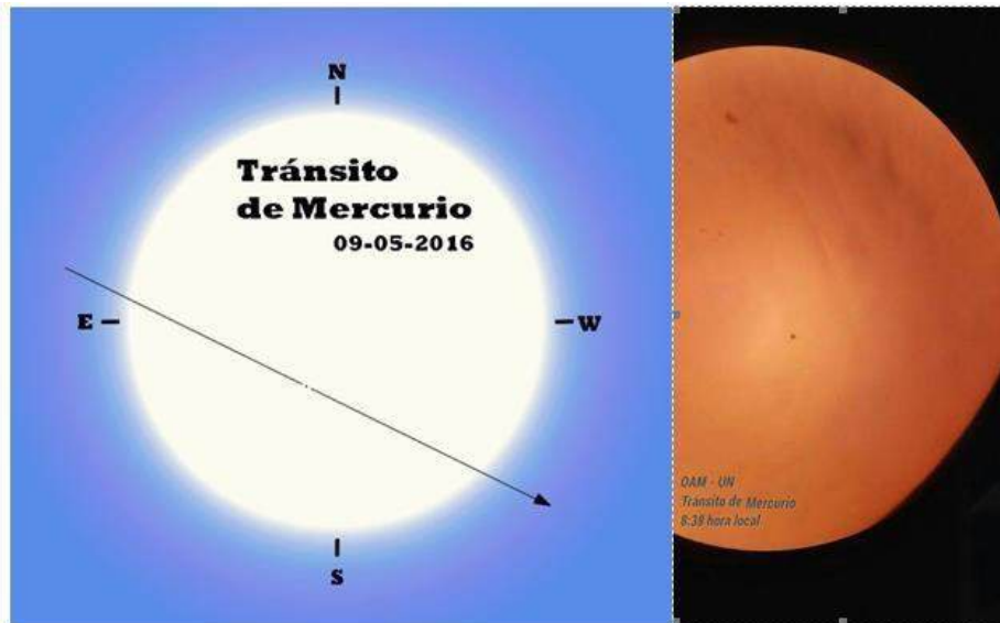
Figura 3.13. Tránsito de Mercurio desde el OAM
