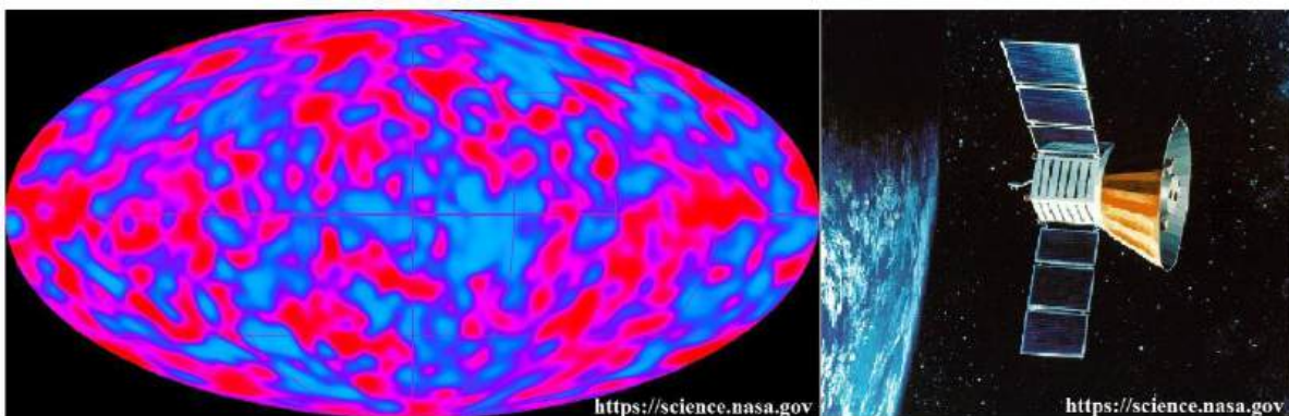
Figura 1.10. Proyecto COBE: mapa de las anisotropías de la radiación de fondo de microondas CMB, formado con los datos tomados por la nave COBE, y Explorador del Fondo Cósmico COBE Fuente, en
