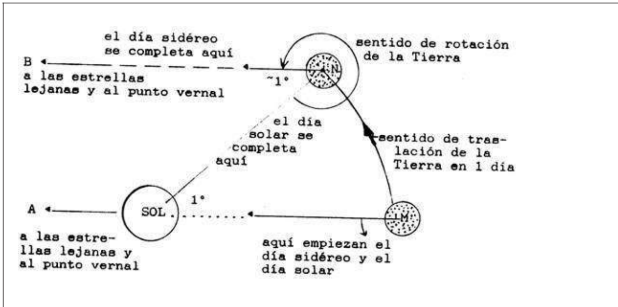
Figura 4.1 Día sidéreo y día solar: el día sideral es más corto que el día solar en casi un grado, puesto que, por la traslación, el Sol parece haberse quedado atrás respecto de las estrellas del fondo (A y B se encuentran en el infinito).
