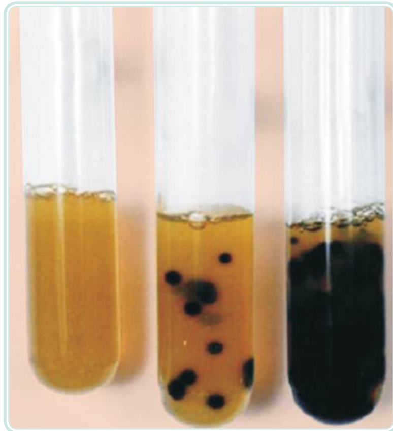
Figura 7.10: Termófilos anaeróbios produtores de H 2 S
