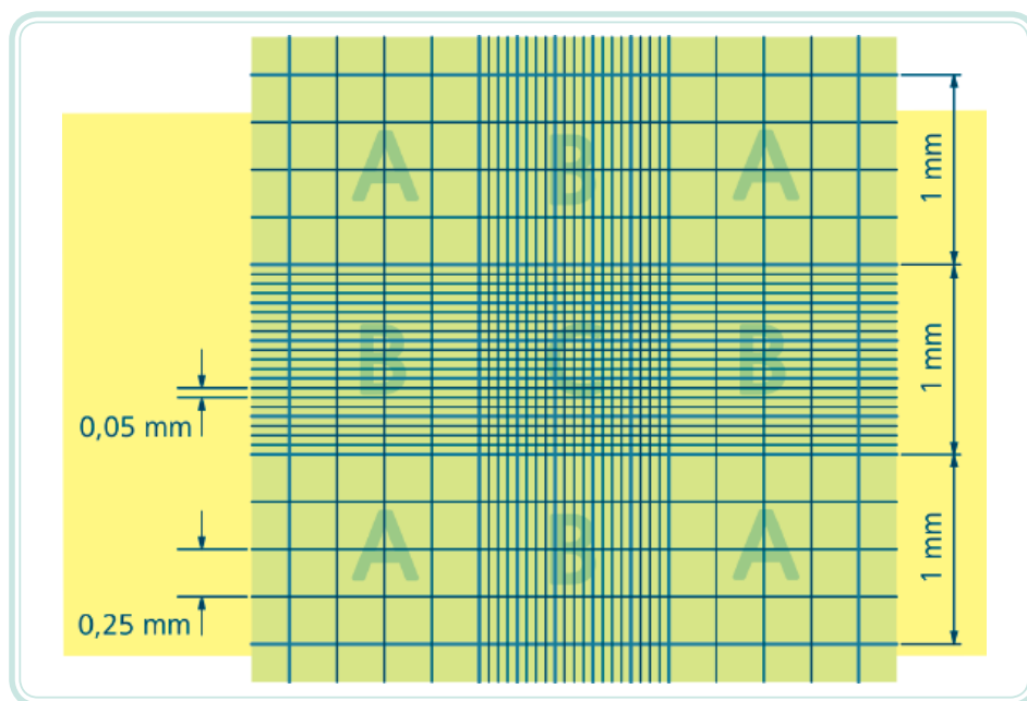
Figura 1.2: Lâmina hematimétrica ou câmara de Neubauer Fonte: CTISM
