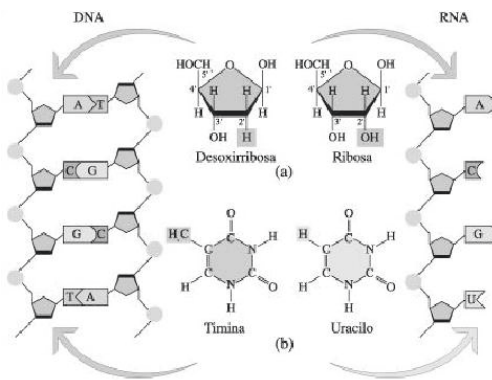
Figura 22. Diferencias entre el ADN y el ARN (Fuente: Curtis y Barnes, 2000).
