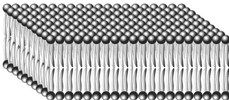
Figura 11. Disposición de los fosfolípidos en las membranas biológicas.
