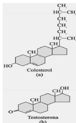
Figura 13. En (a) Estructura química del colesterol; en (b) la testosterona, hormona producida en el testículo y sintetizada a partir del colesterol (Fuente: Curtis y Barnes, 2000)
