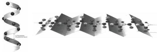
Figura 17. Estructura secundaria: a la izquierda, la hélice \alpha . A la derecha, la hoja plegada \beta (Fuente: Lodish, 2002).
