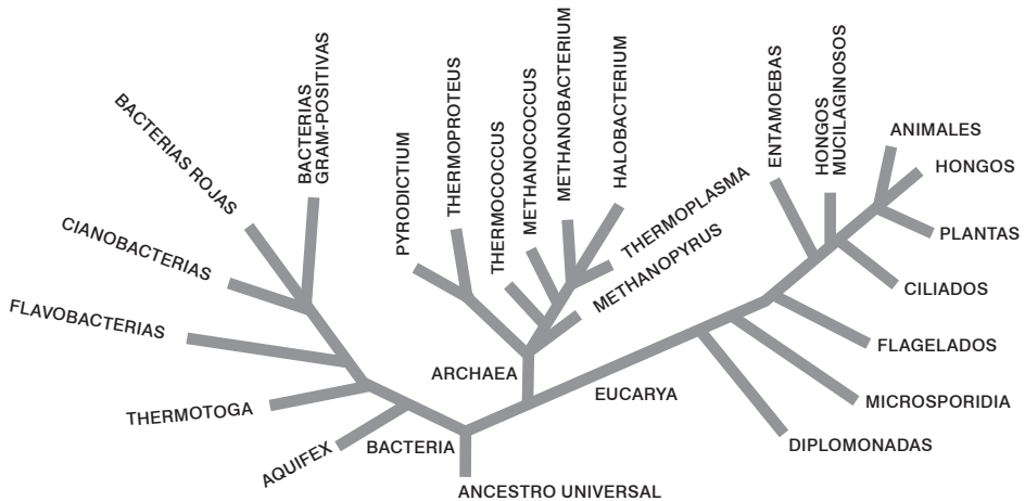
Figura 2. Árbol filogenético basado en tres grandes dominios: Bacterias, Archaea y Eucarya. Modificado de Woese (2000) Interpreting the universal phylogenetic tree. Evolution 97(15): 8392-8396.
