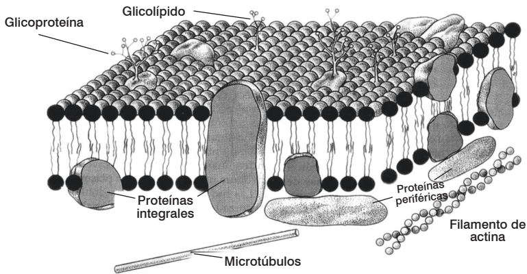
Figura 8. Esquema del mosaico fluido de la membrana celular (Junqueira y Carneiro, 1998). La membrana plasmática está constituida por una bicapa lipídica con proteínas intercaladas. Los azúcares en la membrana sólo se encuentran en la monocapa externa.
