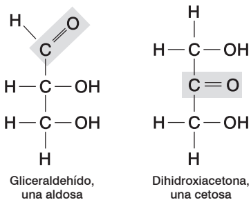
Figura 6. Dos monosacáridos constituidos por tres átomos de carbono, llamados triosas (Fuente: Stryer et al. , 2003).
