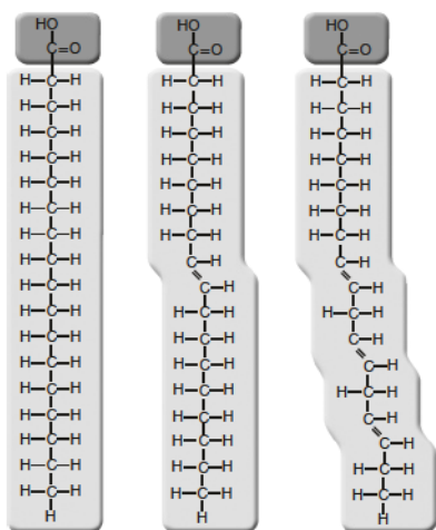
Figura 9. Tres fórmulas estructurales de ácidos grasos. A la izquierda, el ácido esteárico, constituido por una cadena principal de carbono completamente saturada con átomos de hidrógeno. En el medio se observa el ácido oleico, que tiene un doble enlace en su cadena principal, y por lo tanto es un ácido graso no saturado. A la derecha, el ácido linolénico, que tiene tres dobles enlaces, por lo que es poliinsaturado (Fuente: Starr-Taggart, 2004).
