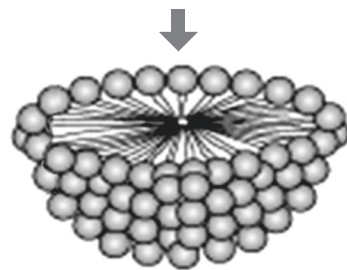
Figura 10. Esquema de una micela.
