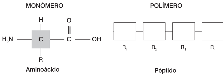
Figura 15. Formación de un polímero por enlaces peptídicos (Fuente: Stryer et. al. , 2003).
