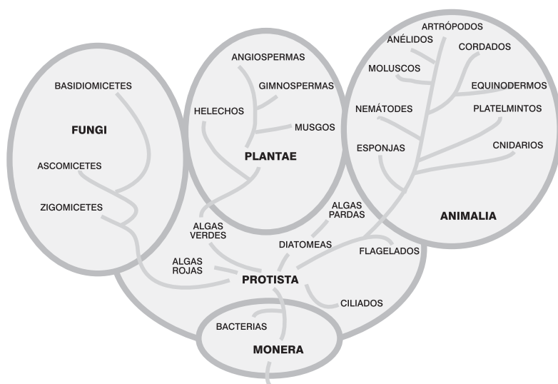
Figura 1. Árbol filogenético tradicional, basado en el sistema de cinco reinos (modificado de Spivak, 2006).
