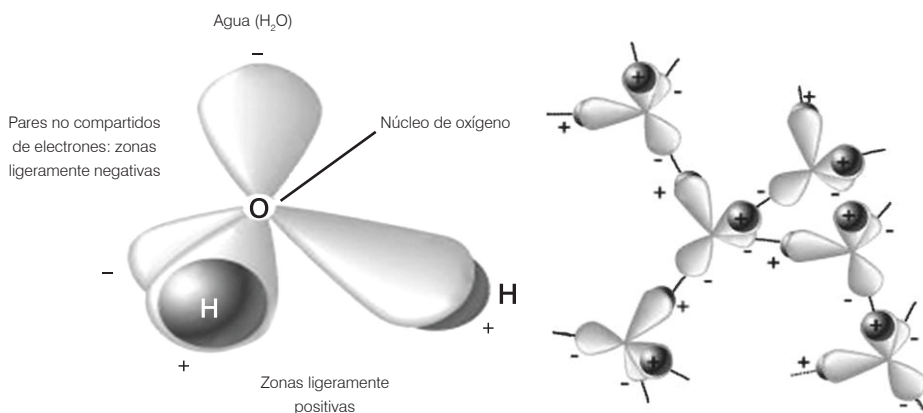
Figura 3. A la izquierda, la molécula de agua representada según el modelo atómico orbital que muestra las zonas de la molécula ligeramente positivas y ligeramente negativas. A la derecha, la formación de puentes de hidrógeno entre las moléculas de agua (Fuente: Curtis y Barnes, 2000).
