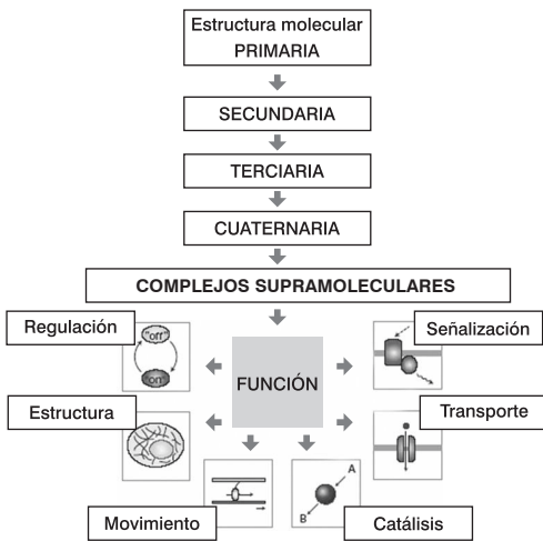
Figura 20. Resumen general de estructura y función de las proteínas (Fuente: Stryer, 2003).
