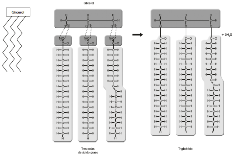
Figura 12. Estructura química de un triglicérido: a la izquierda, el esquema. A la derecha se observa la condensación de ácidos grasos con una molécula de glicerol para formar el triglicérido. Observa que al igual que los fosfolípidos, las colas de ácidos grasos no son siempre iguales, y pueden ser saturadas e insaturadas (Fuente: Starr-Taggart, 2004).
