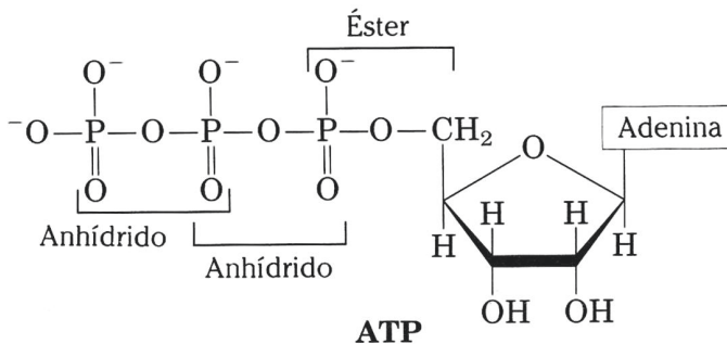
Figura 1. Estructura química del ATP, la moneda energética de las células. Los tres enlaces entre los fosfatos retienen gran cantidad de energía que se libera al romperse cada uno de estos.
