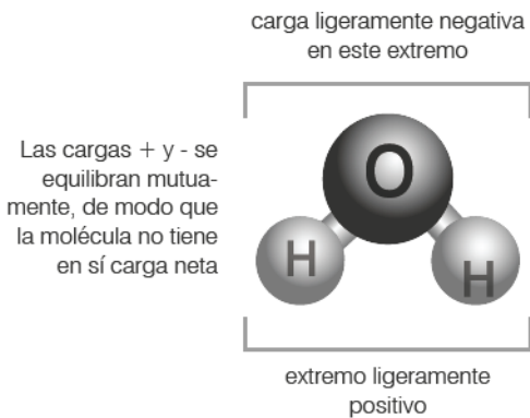
Figura 2. Estructura molecular del agua (Fuente: Starr-Taggart, 2004).
