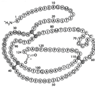
Figura 18. Estructura terciaria de una enzima, la ribonucleasa. Cada círculo representa un aminoácido. Se muestran pintados los puentes disulfuro que se forman entre aminoácidos alejados entre sí (Fuente: Stryer et ál. , 2003).
