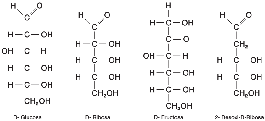
Figura 7. Monosacáridos de 5 y 6 átomos de carbono (Fuente: Stryer et al. , 2003).
