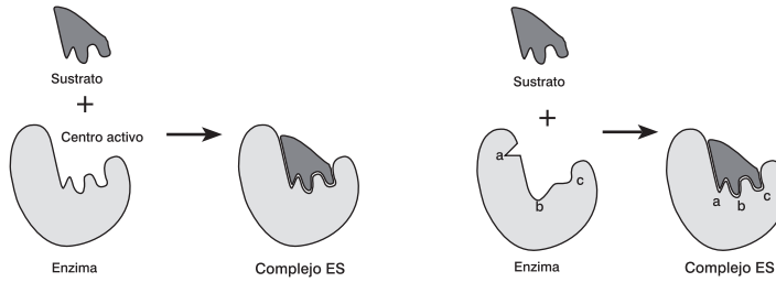
Figura 1. Modelos de interacción enzima-sustrato. A la izquierda, modelo de llave-cerradura. A la derecha, modelo de ajuste inducido (Fuente: Stryer, 2003).
