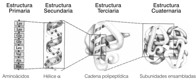
Figura 19. Los cuatro niveles de organización de las proteínas (Fuente: Stryer et al. 2003).
