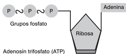
Figura 21. Estructura del adenosintrifosfato (ATP) (Fuente: Curtis y Barnes, 2000).
