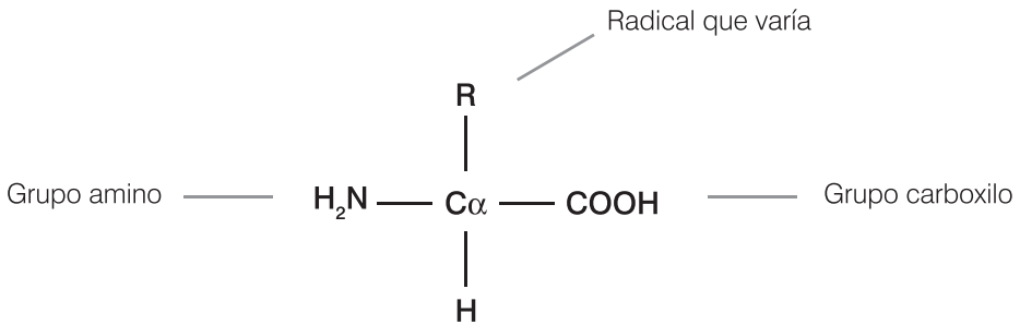
Figura 14. Estructura de un aminoácido.
