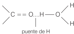
Figura 4. Formación de puentes de hidrógeno entre el agua y otros grupos químicos.
