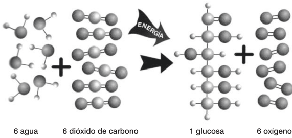
Figura 2. El resultado neto de la fotosíntesis es la obtención de moléculas de glucosa, siguiendo la reacción general que se esquematiza: 6 \text{H}_2\text{O} + 6 \text{CO}_2 = 1 \text{glucosa} + 6 \text{O}_2 (Fuente: Alajnti, 1997).
