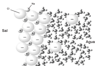
Figura 5. Acción disolvente del agua (Fuente: Curtis y Barnes, 2000).
