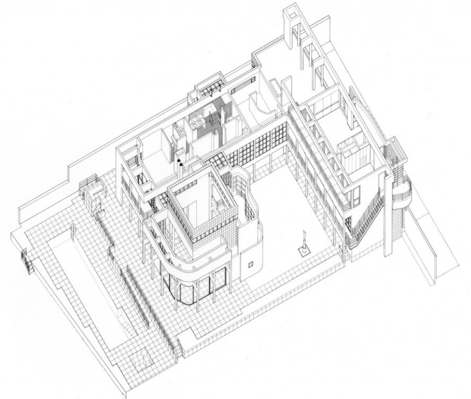
Fig. 3.3.7 AXONOMETRÍAS
