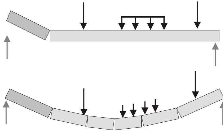
FLEXIÓN
