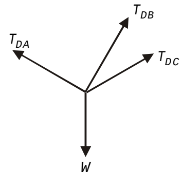
Diagrama de cuerpo libre
