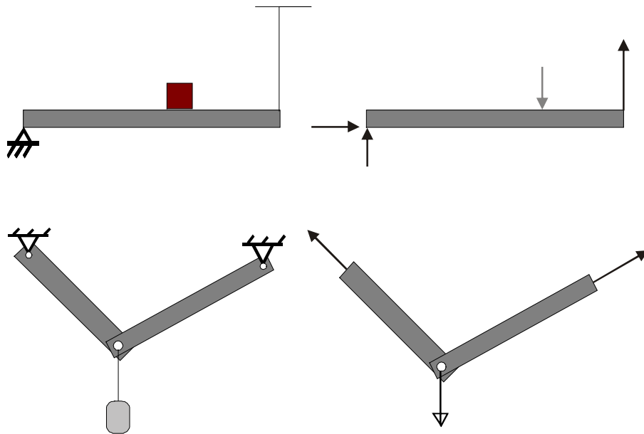
FUERZAS CONCENTRADAS
