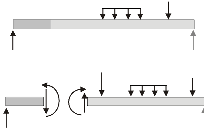
SENTIDOS POSITIVOS DE V Y M
