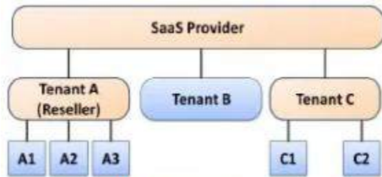
Fig 3 Tenant Tree
