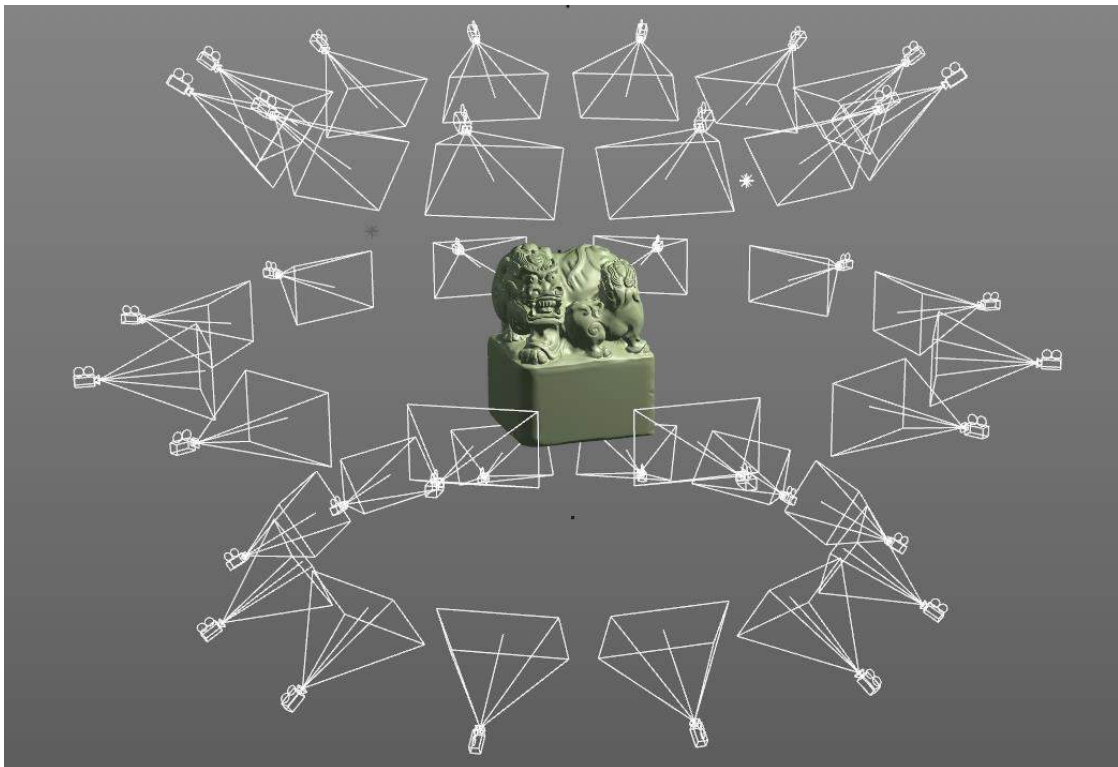
Figura 4-7. Ejemplo de disposición de cámaras para la realización de fotogrametría compleja.
