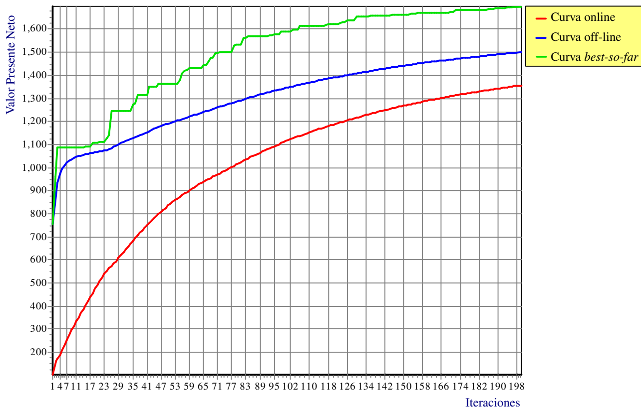
Figura 7.17: Ejemplo de curvas best-so-far , off-line y online .
