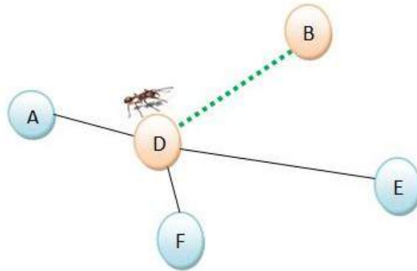
Figura 8.7: Muestra los nodos validos en base a la nueva posición de la hormiga.
