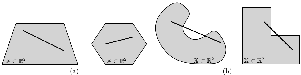
Figura 7.2: Espacios convexos y no convexos
