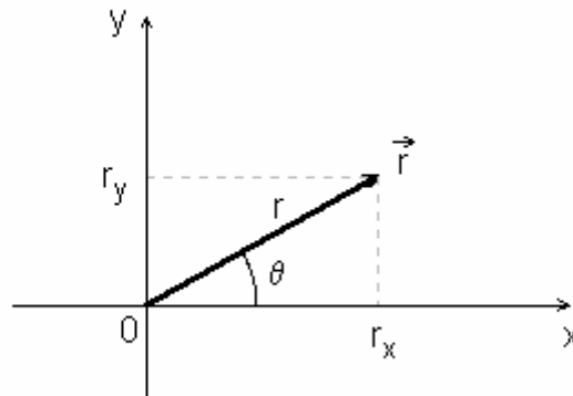
Figura 3 — Vetor posição.
