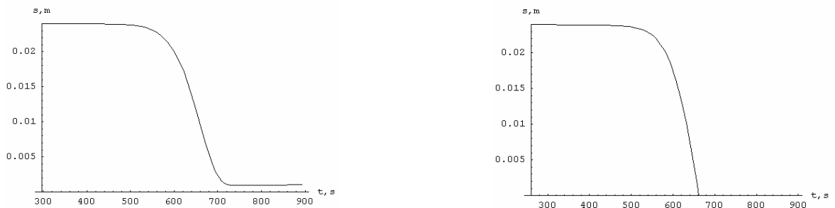
Figura 1 – Variação da espessura do material do sistema de proteção térmica em função do tempo de voo
