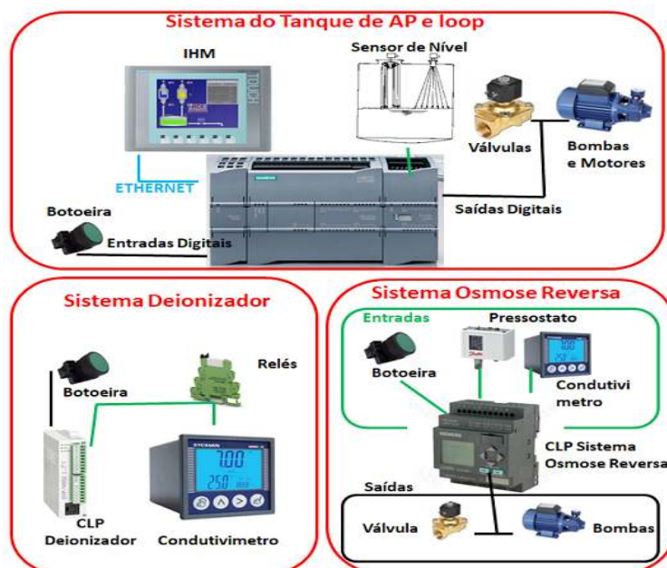
Figura 10. Arquitetura descentralizada da ETA antes da adequação.
