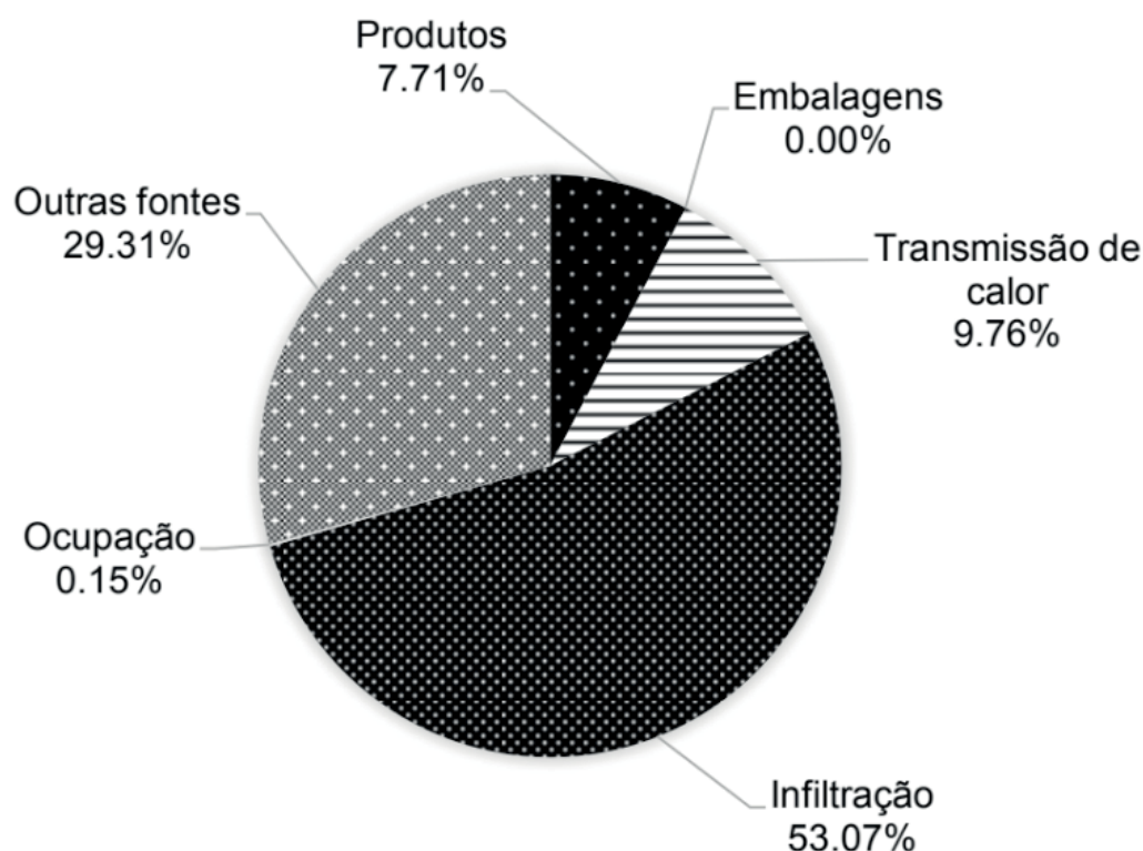
Figura 4. Distribuição das fontes de cargas térmica.
