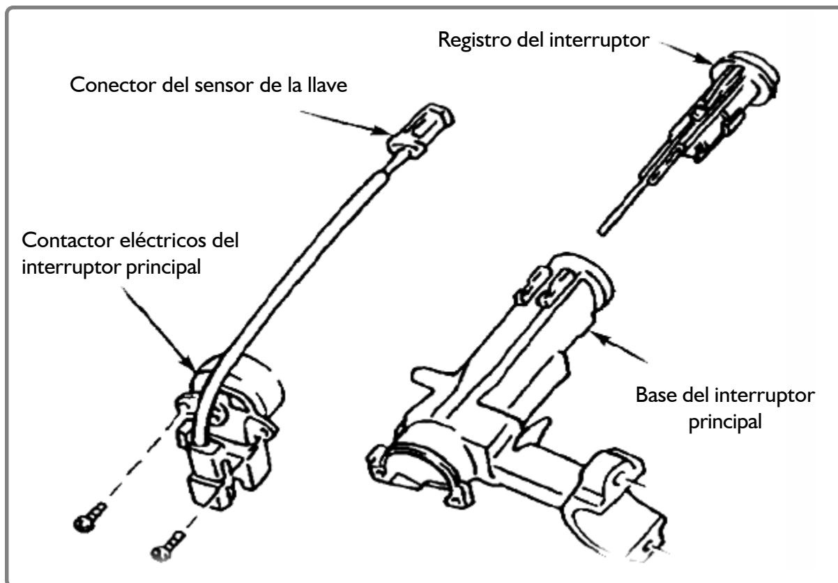
Figura 2-11 Conector del sensor de la llave
