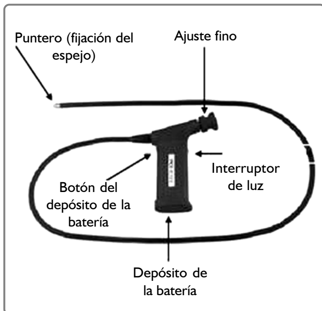
Figura 1-21 Equipo para videoscopia
