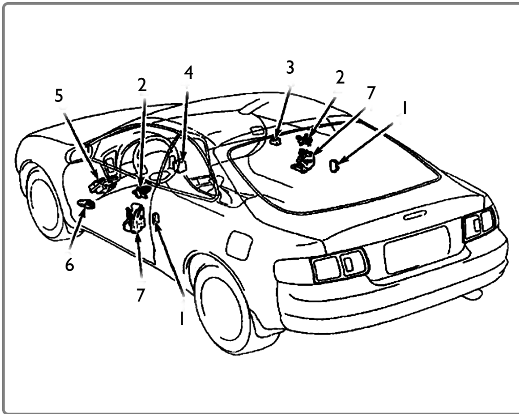
Figura 2-1 Componentes de la cerradura central
