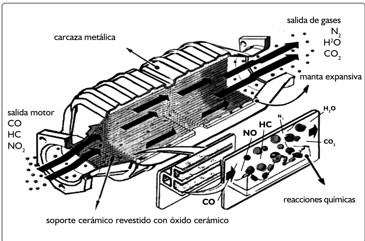
Figura 2-35 Convertidor catalítico
