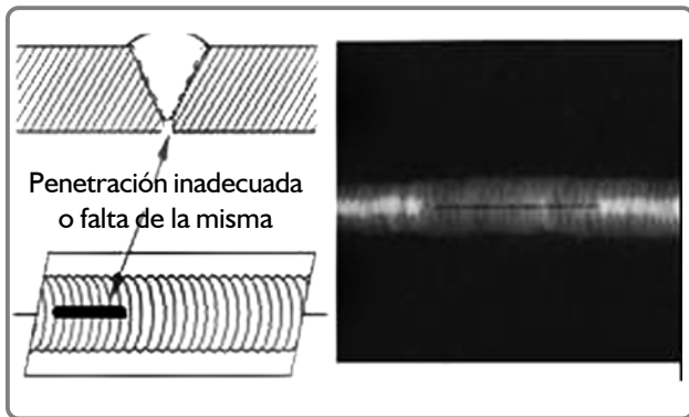
Figura 1-18 Falta de fusión detectada con radiografía
