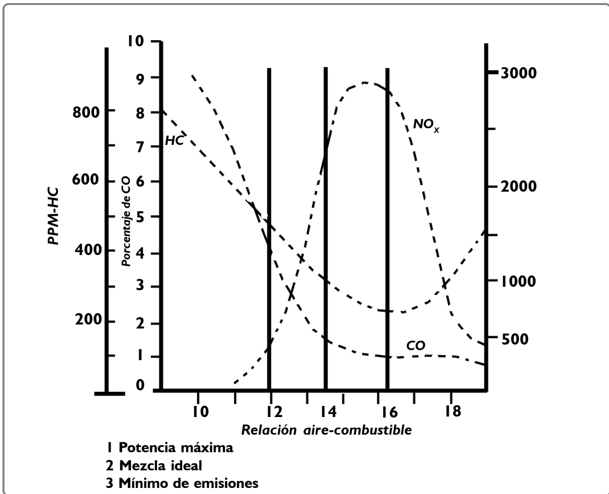
Figura 2-39 Gráfico de emisiones comparado en relación aire combustible
