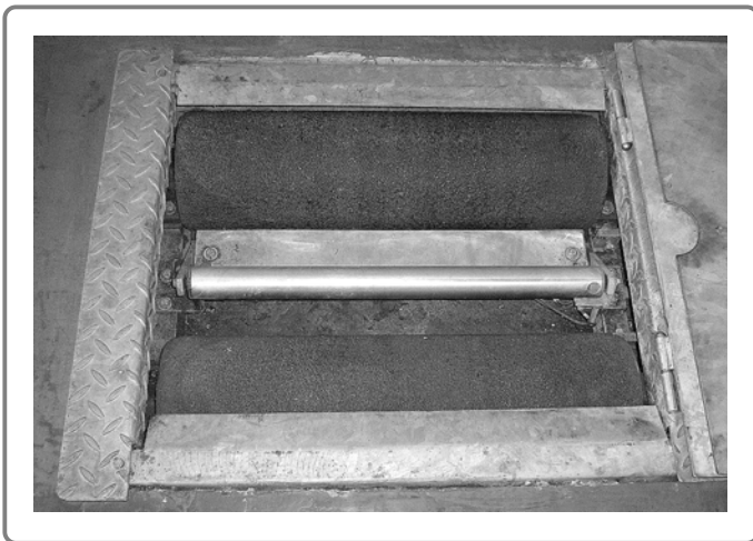
Figura 1-10 Rodillos y sensor del frenómetro
