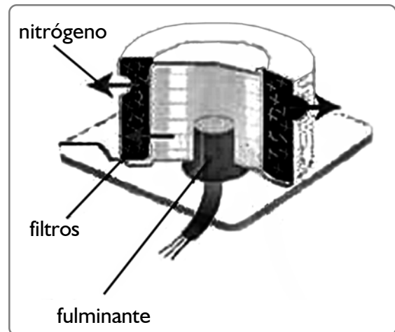
Figura 2-14 Componentes de la bolsa de aire
