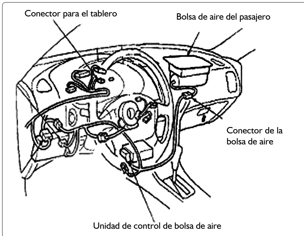
Figura 2-13 Componentes del sistema de bolsa de aire
