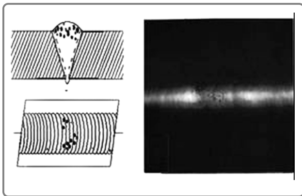
Figura 1-17 Porosidad detectada con radiografía
