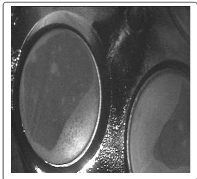
Figura I-15 Fotografía utilizando videoscopia en donde se muestra los depósitos de carbón en los asientos de las válvulas en una culata de cilindros de un motor a Diesel
