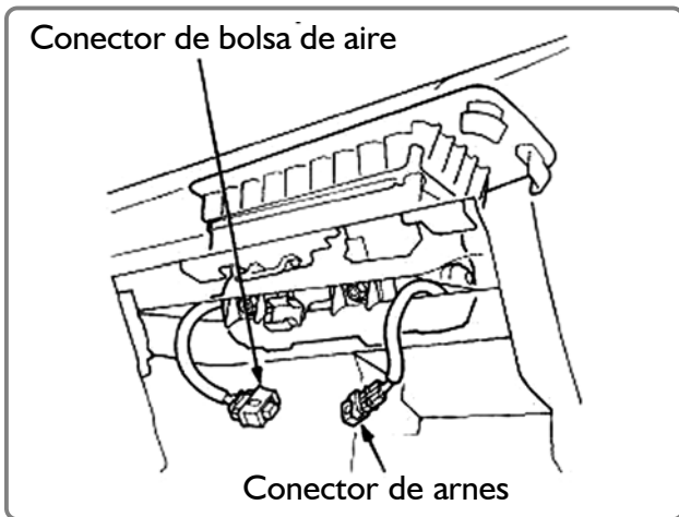
Figura 2-22 Conector de bolsa de aire
