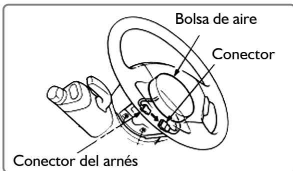
Figura 2-23 Bolsa de aire
