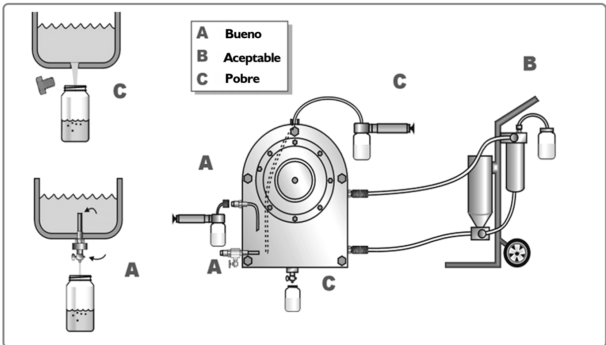
Figura 1-29 Extracción de muestra de aceite
