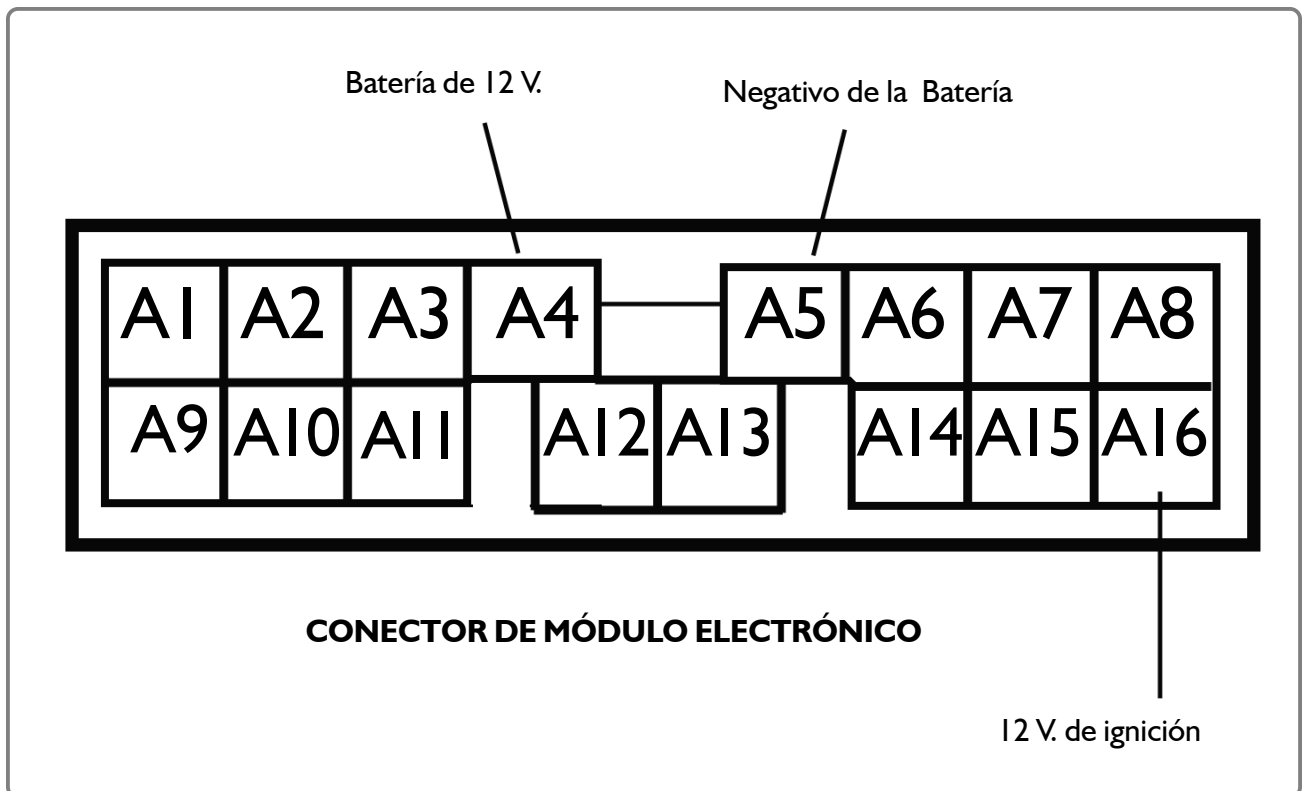
Figura 2-18 Conector de módulo electrónico
