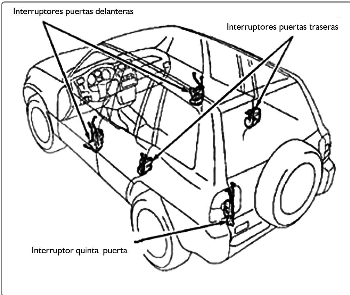
Figura 2-19 Interruptores del sistema de cerradura central
