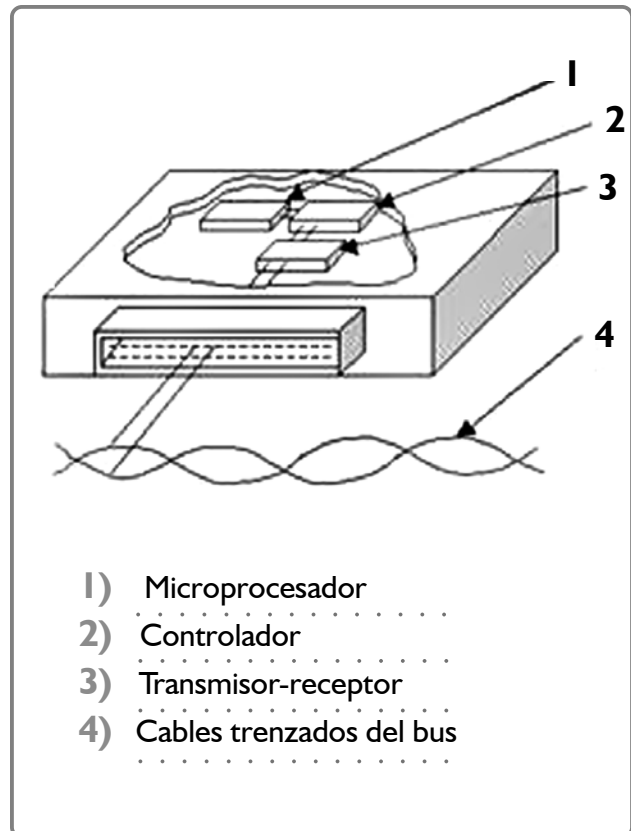
Figura 2-27 Transmisor y receptor
