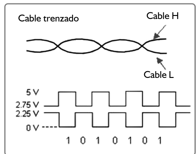
Figura 2-24 Forma de señal en la red can
