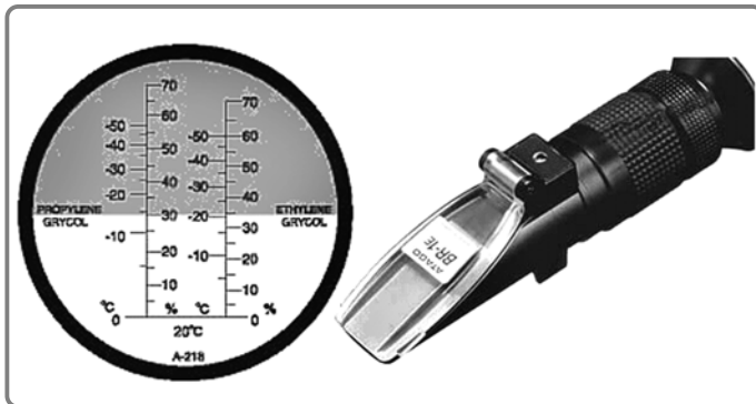
Figura 1-34 Refractómetro
