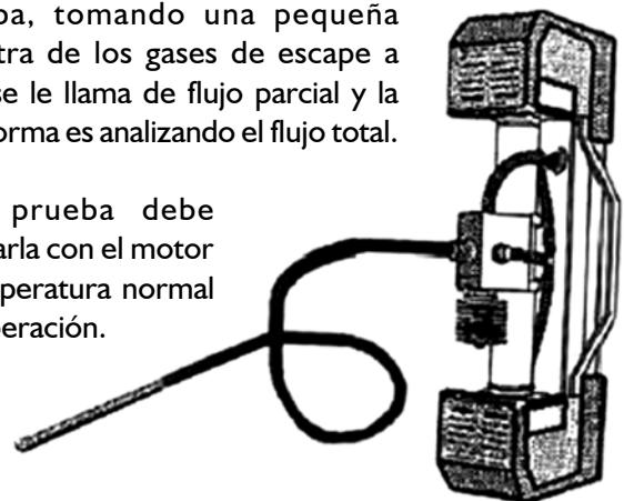
Figura 2-34 Medidor de opacidad de flujo parcial
