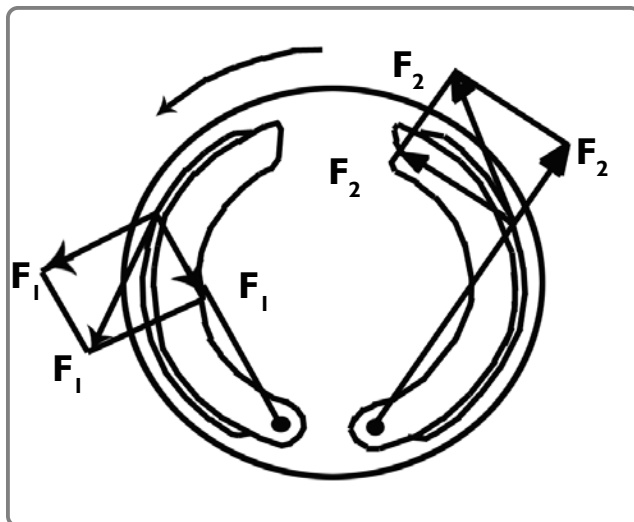
Figura 1-6 Distribución de fuerzas de frenado
