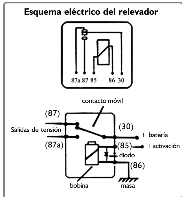
Figura 2-6 Esquema eléctrico del Relevador
