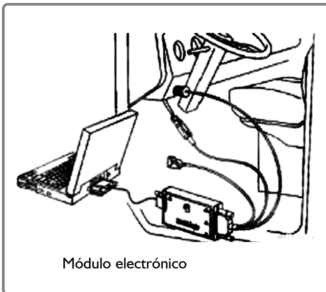
Figura 2-7 Módulo electrónico
