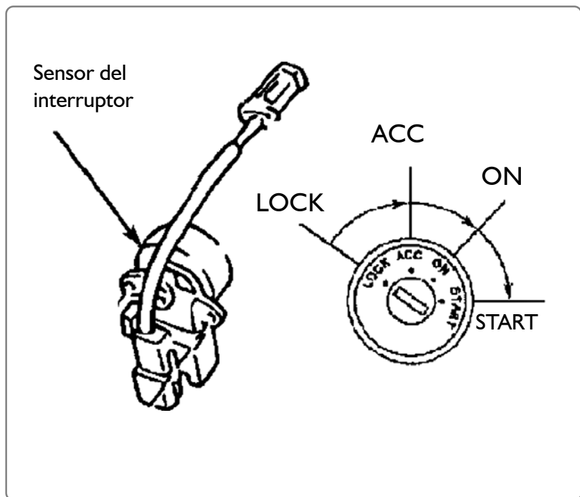
Figura 2-12 Interruptor del sistema anti robo
