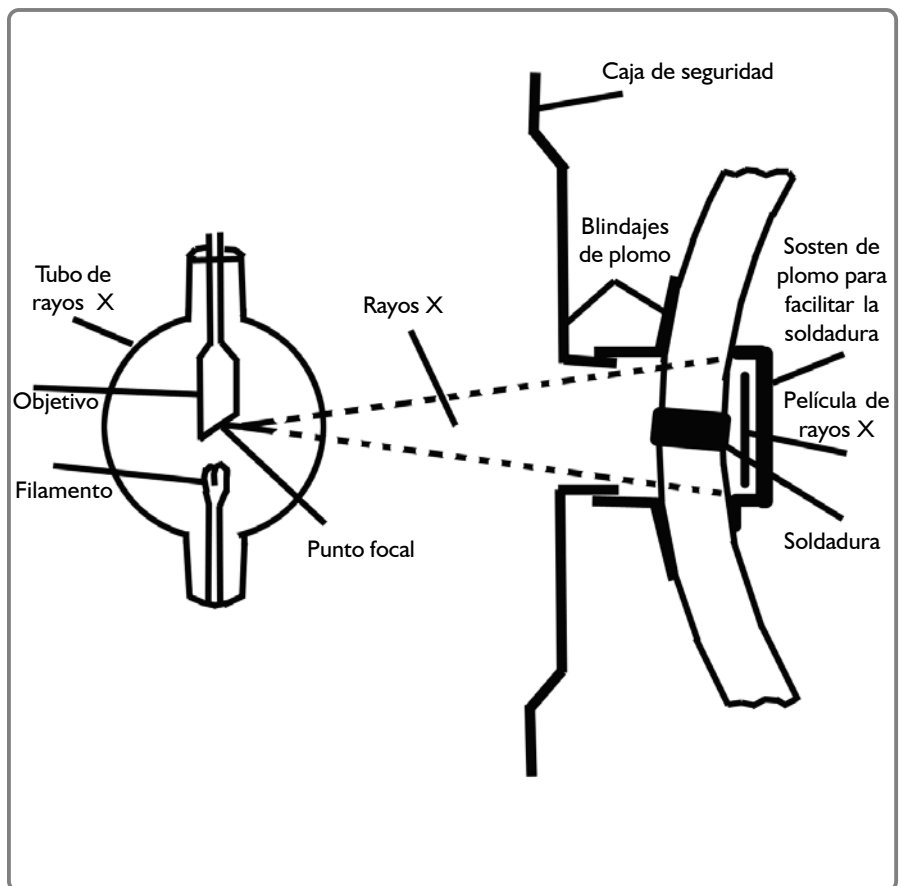
Figura I-20 Funcionamiento de radiografía por medio de rayos X
