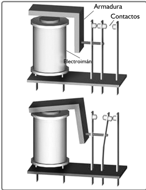
Figura 2-5 Relevadores utilizados en el sistema de cerradura central
