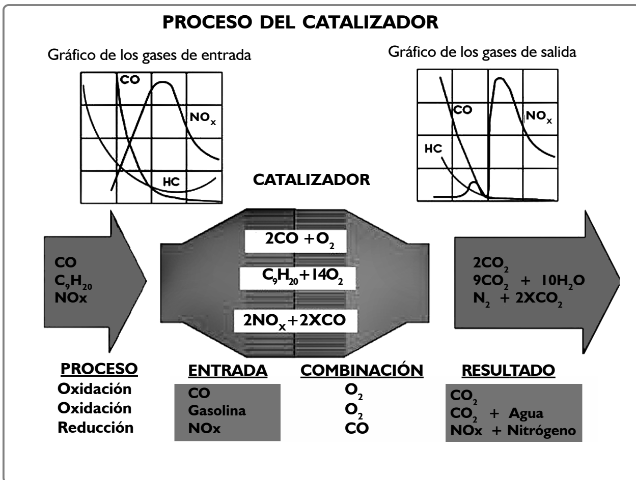
Figura 2-36 Proceso del catalizador
