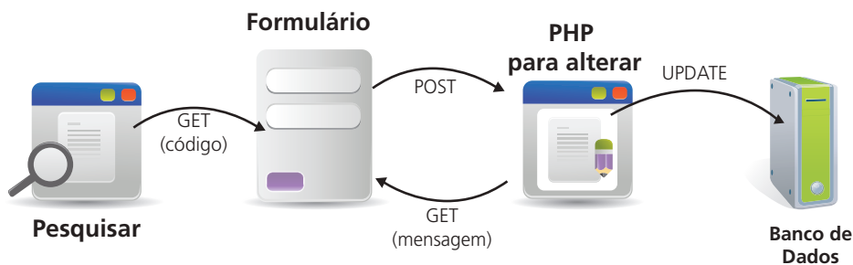
Figura 4.6: Diagrama de navegação das páginas para alterar dados
