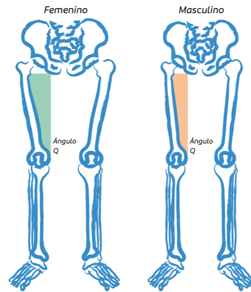
Figura 4 – Ensanchamiento de cadera
