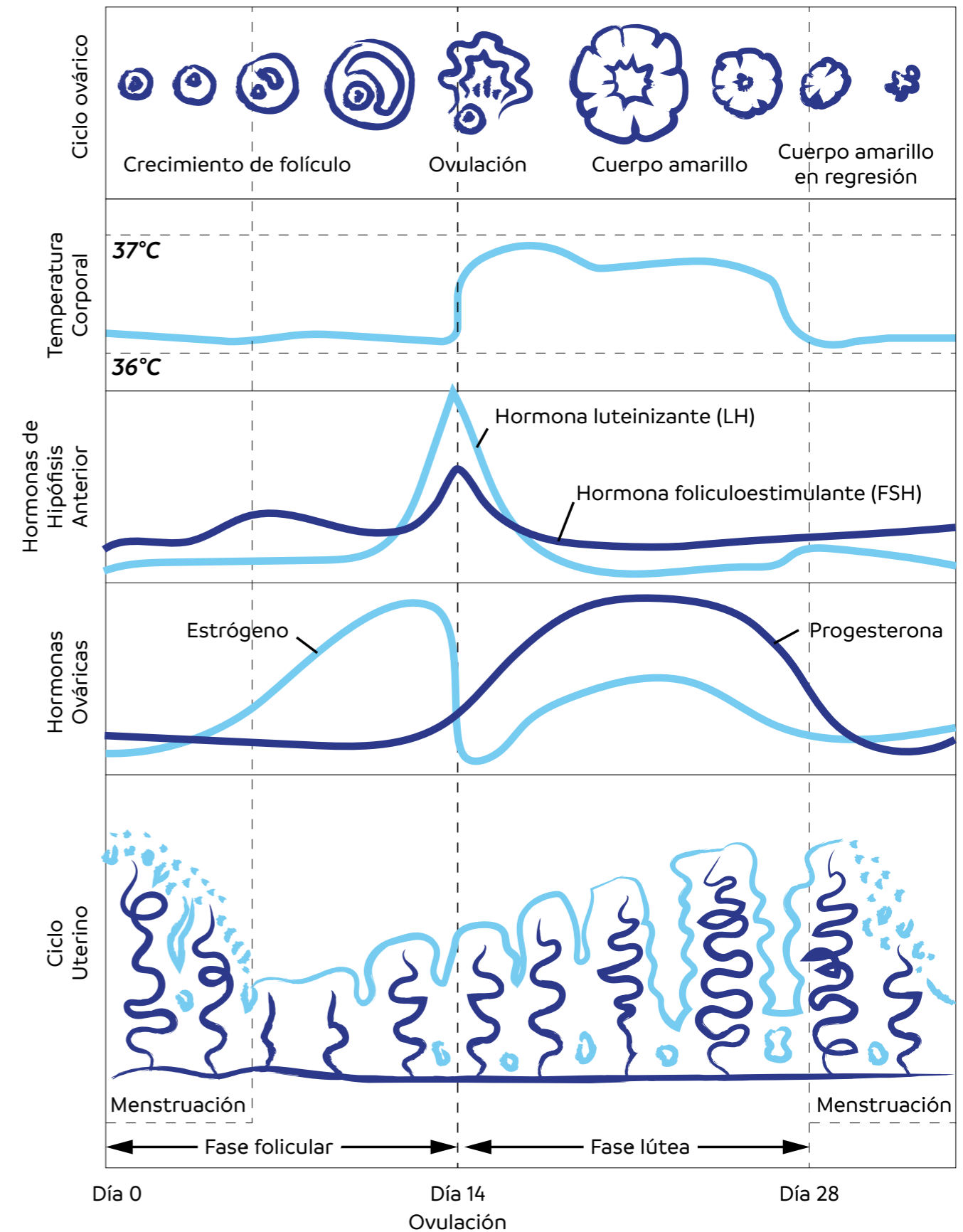
Figura 2 – Regulación del ciclo menstrual
