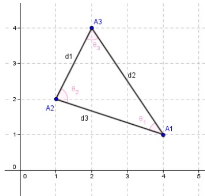
Figura 2.34: Representação geométrica do triângulo [A_1A_2A_3]
