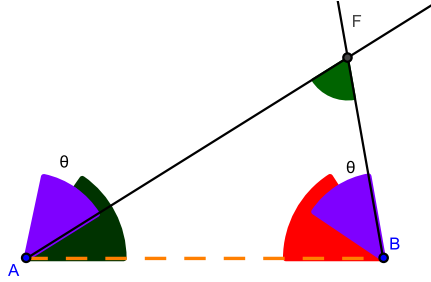
Figura 2.27: Triângulo AFB, do Polígono de Região R4.
