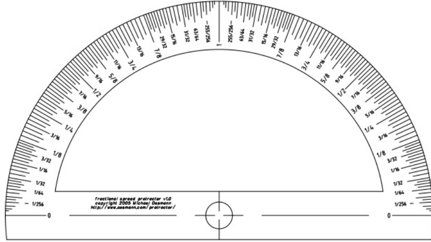
Figura 2.33: Transferidor da Trigonometria Racional
