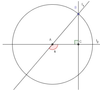
Figura 2.32: Separação de duas retas: afastamento
