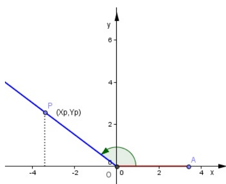
Figura 2.10: Ponto P no 2º Quadrante
