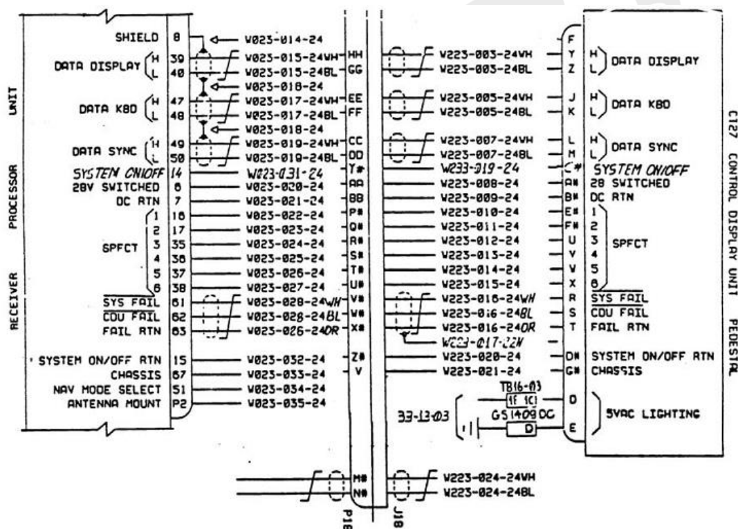
Figura 6- 10 Modificação do número na passagem por conector
