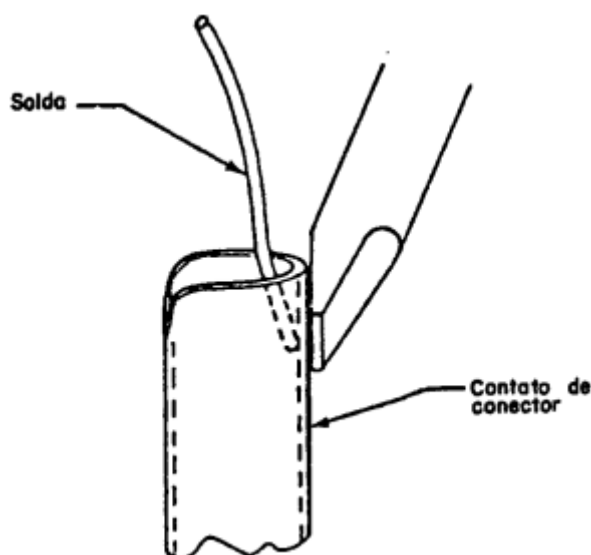
Figura 6-58 Aplicação de solda
