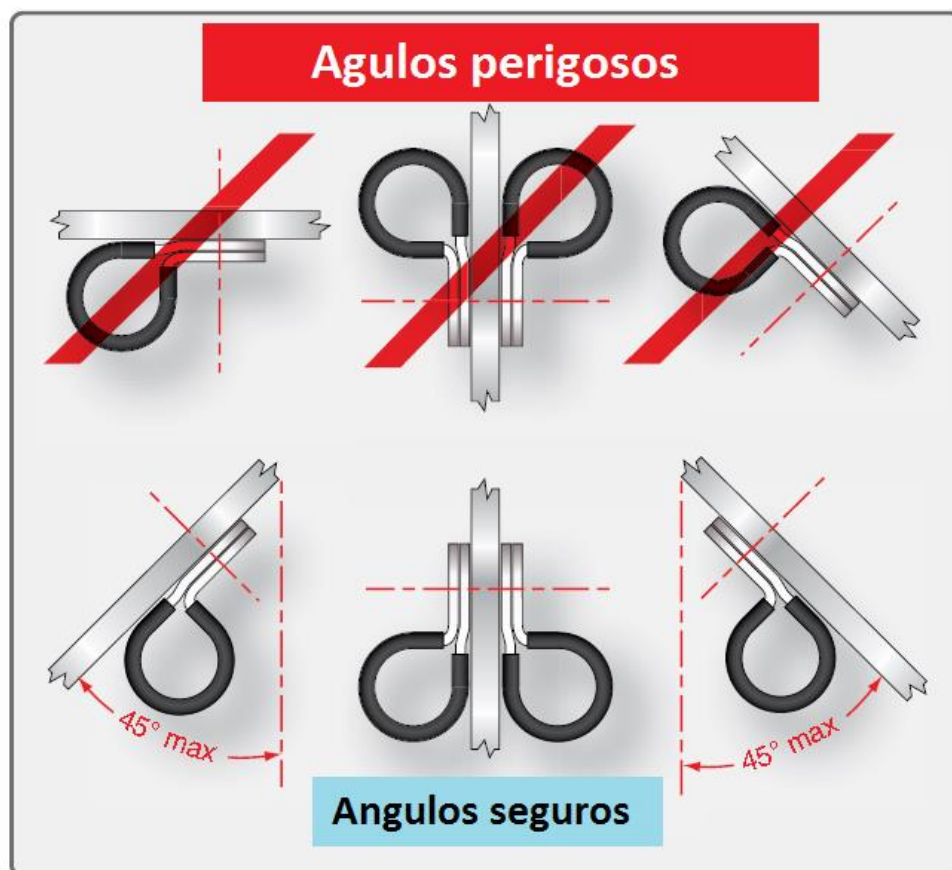
Figura 6-26 Ângulos de montagem adequados para braçadeiras de cabo
