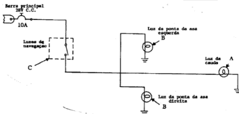
Figura 6-91 Circuito das luzes de posição sem pisca-pisca
