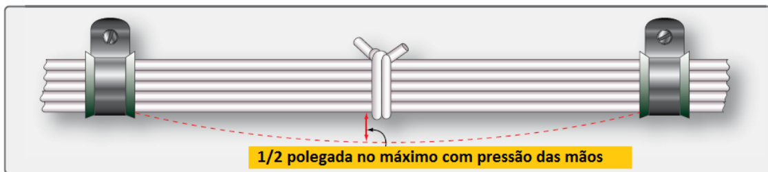
Figura 6-21 Frouxidão no chicote, entre os suportes
