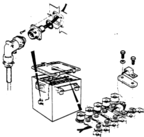
Figura 6-110 Bateria NI-CAD
