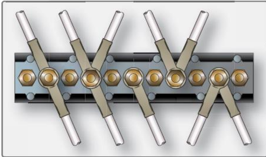
Figura 6-44 Conexão de terminais a blocos de terminais
