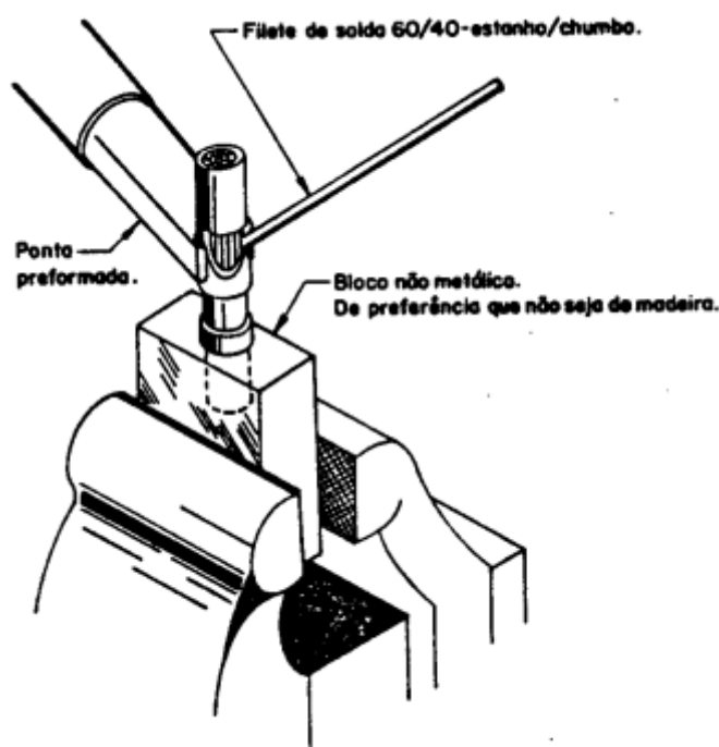
Figura 6-61 Procedimento de soldagem de grandes contatos
