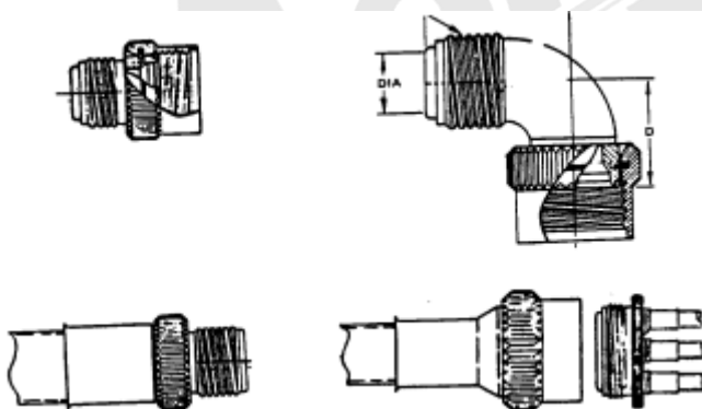
Figura 6-33 Diversos tipos de adaptadores
