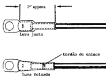
Figura 6-41 Luva isolante
