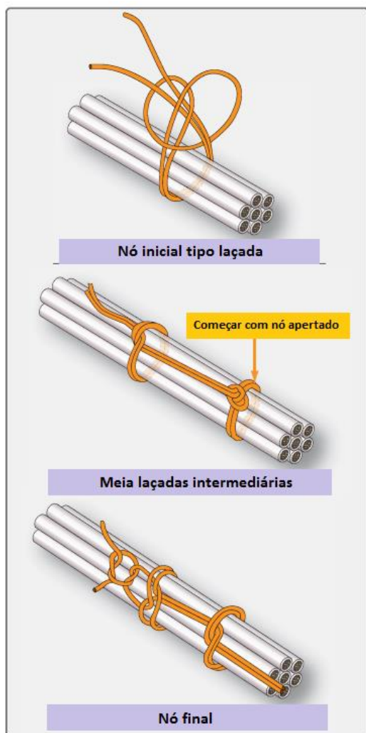
Figura 6-18 Amarração contínua iniciada com nó de laçada
