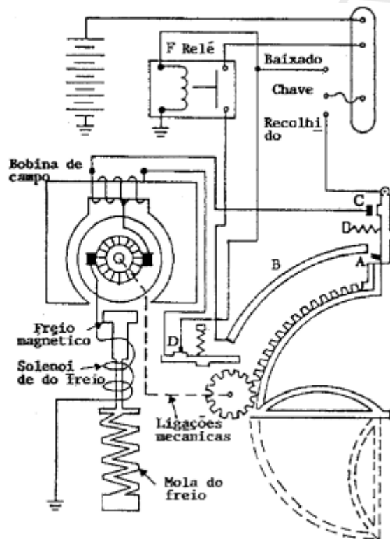
Fig. 6-96 Circuito e mecanismo da luz de pouso
