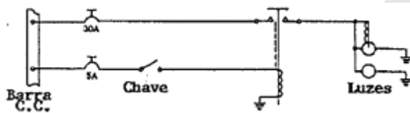
Figura 6-99 Circuito típico de luz de taxi
