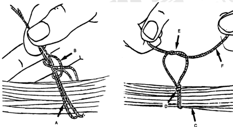
Figura 6-16 Amarração com nó de laçada
