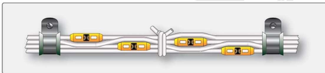
Figura 6-20 Emendas afastadas em um chicote
