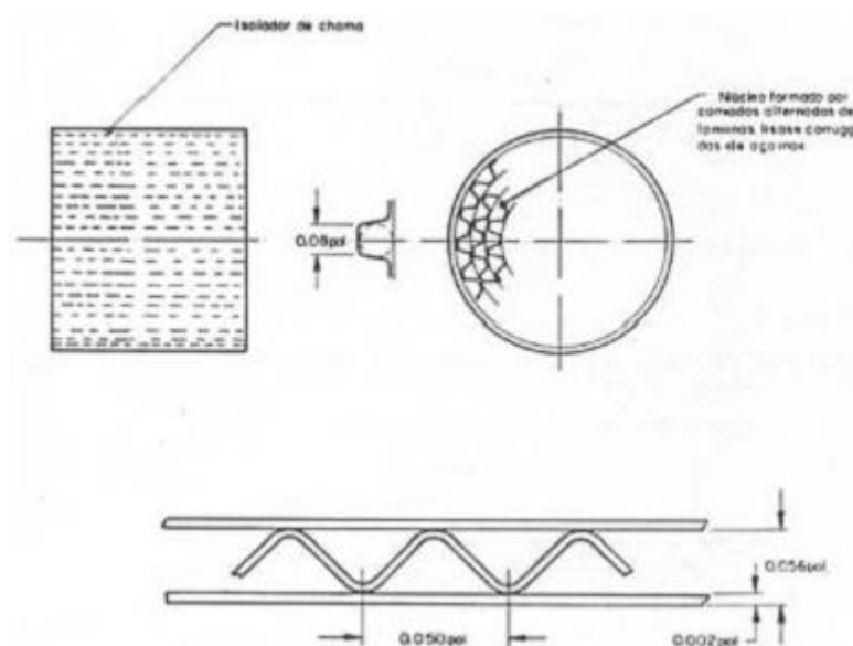
Figura 6-70 Típico isolador de chama
