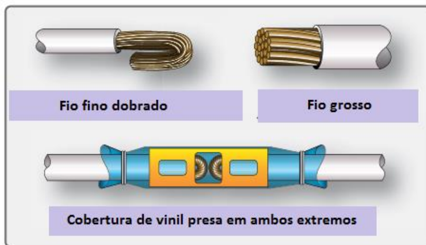
Figura 6-43 Redução da bitola do fio com uma emenda permanente
