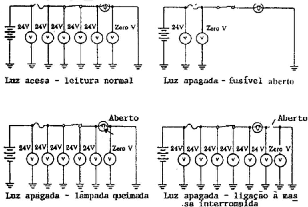
Figura. 6-102 Teste de continuidade com um voltímetro
