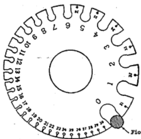
Figura 6- 3 Calibre para fio
