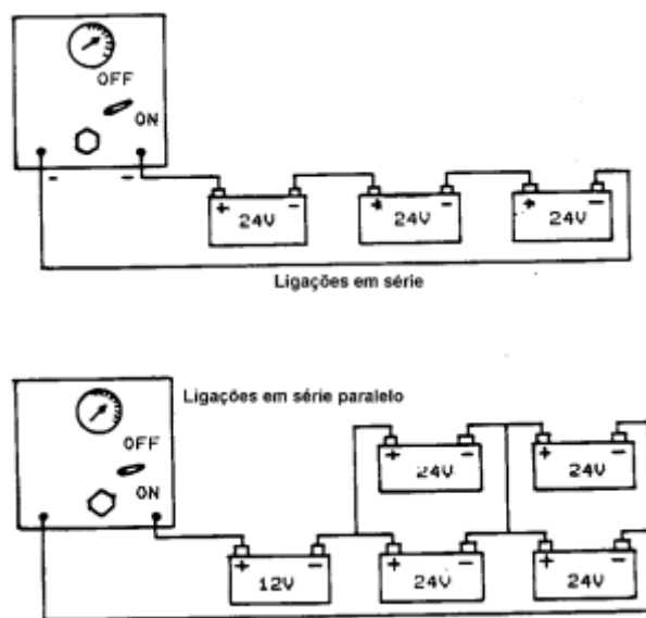
Figura 6-107 Ligações para carga de baterias
