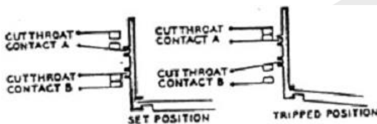
Figura 6-84 Contatos do disjuntor
