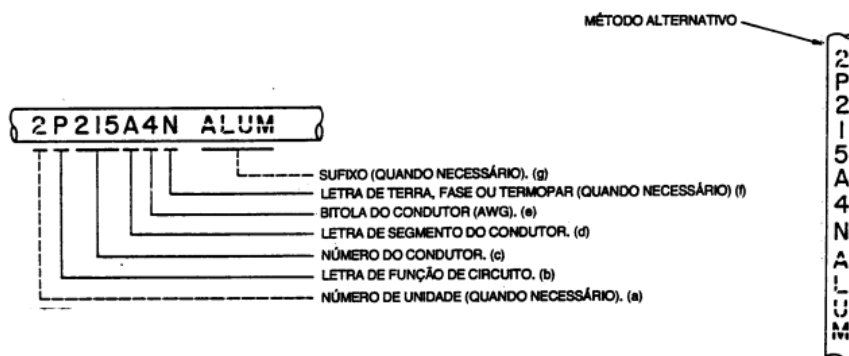
Figura 6-9 Identificação tipo "significante"
