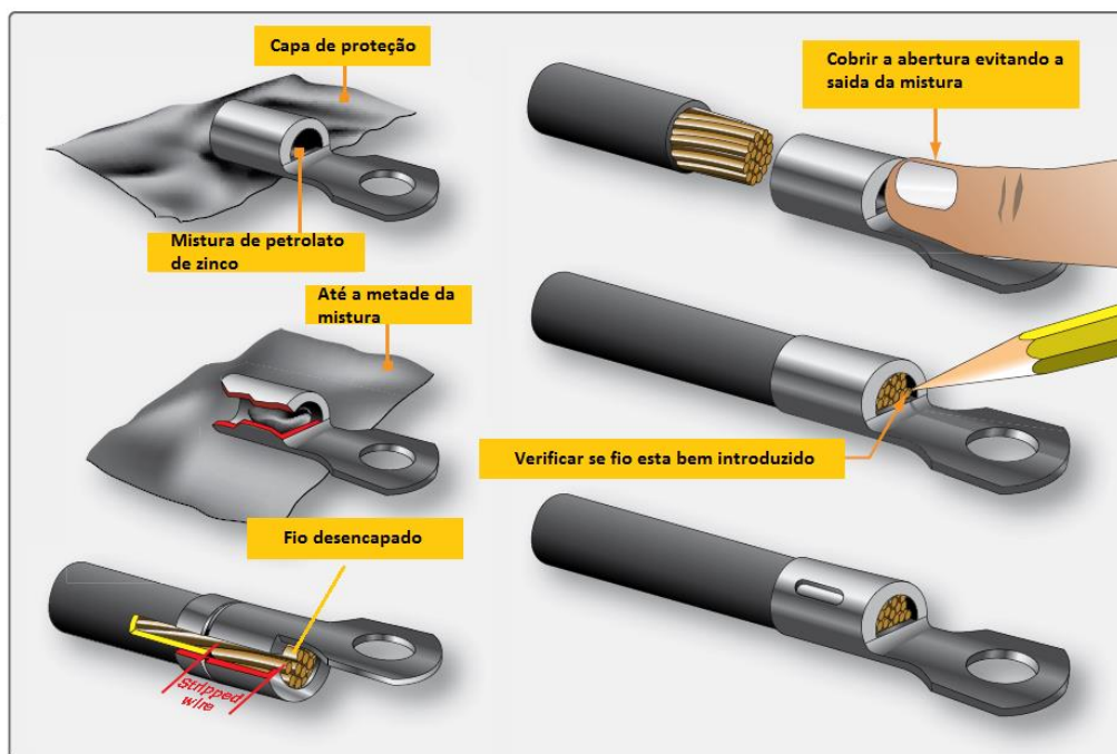
Figura 6-42 Introdução de fio de alumínio em terminal de alumínio
