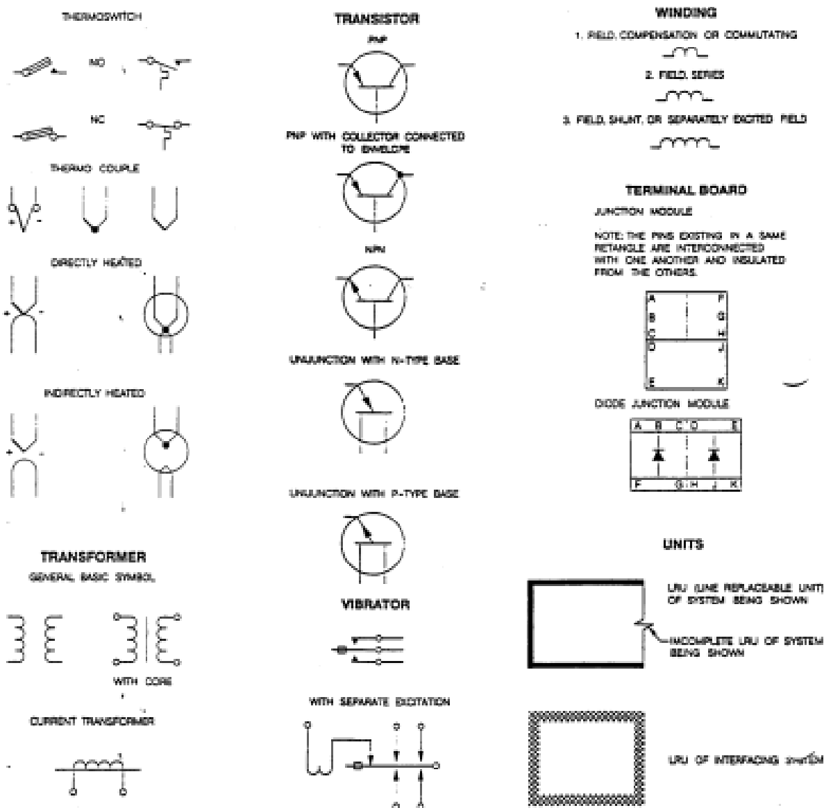
Figura 6-123 Símbolos elétricos X
