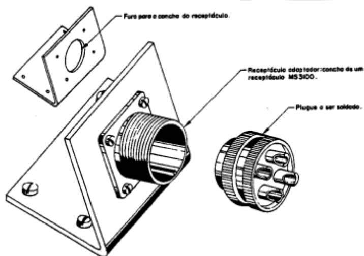
Figura 6-63 Suporte para soldagem de plugues de conectores
