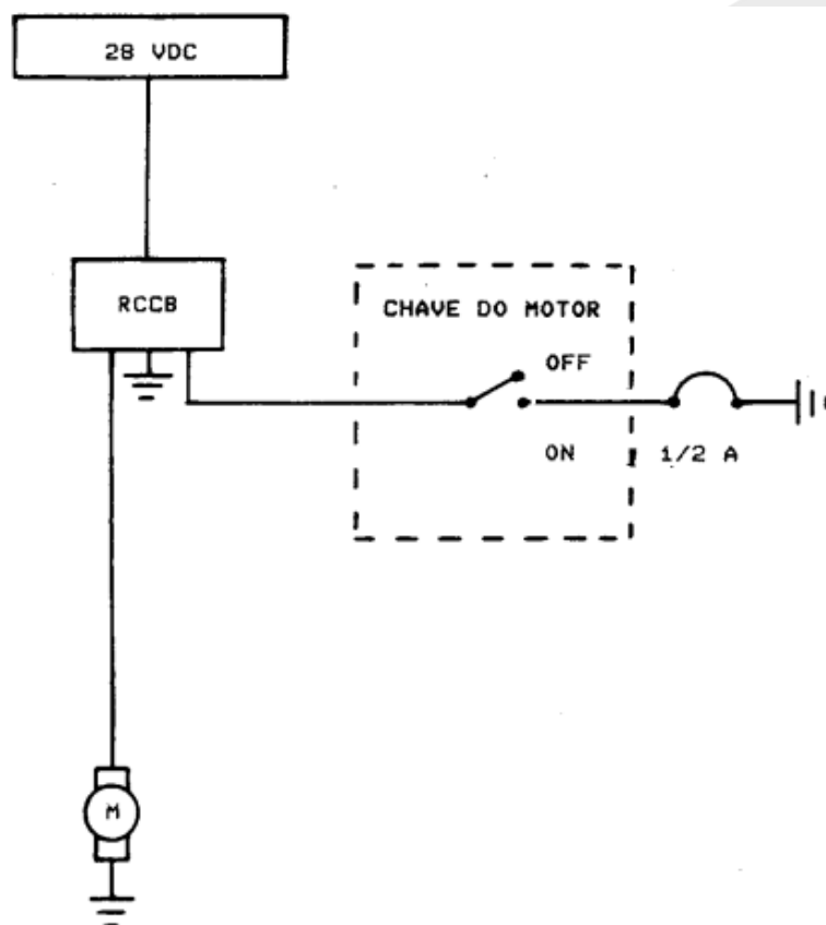
Figura 6-87 Diagrama simplificado usando o RCCB
