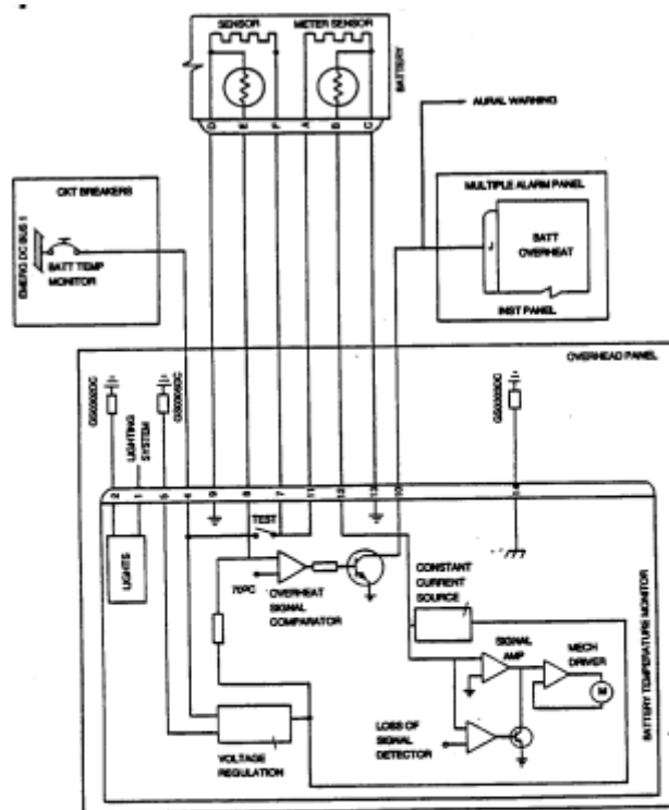
CIRCUITO TÍPICO DE MONITOR DE TEMPERATURA
