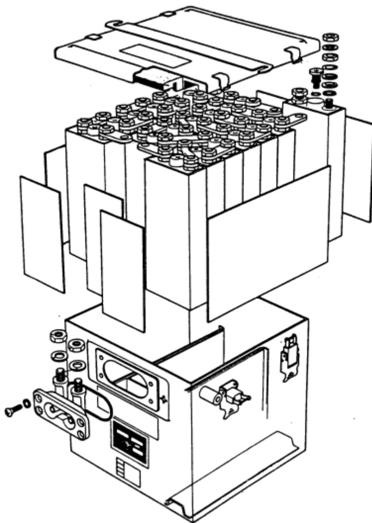
Figura 6 -112 Vista explodida da bateria Níquel-Cádmio
