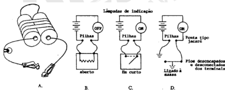
Figura 6-100 Teste com um medidor de continuidade
