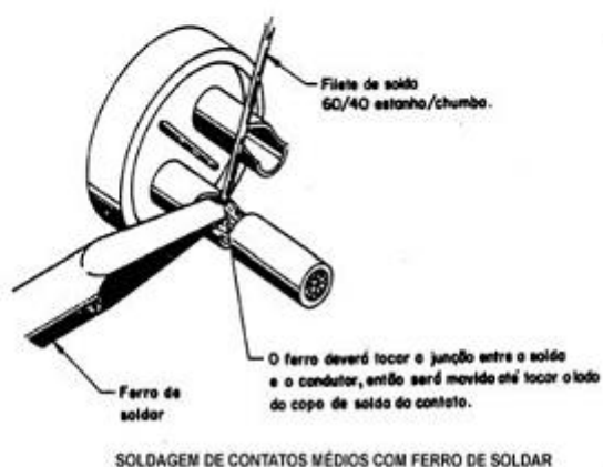
Figura 6-62 Soldagem de acordo com o tamanho dos contatos
