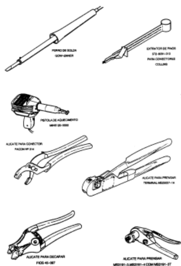
Figura 6-35 Diversas ferramentas para manutenção elétrica
