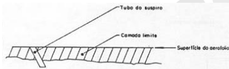
Figura 6-68 Saída do suspiro de combustível - Classe 2
