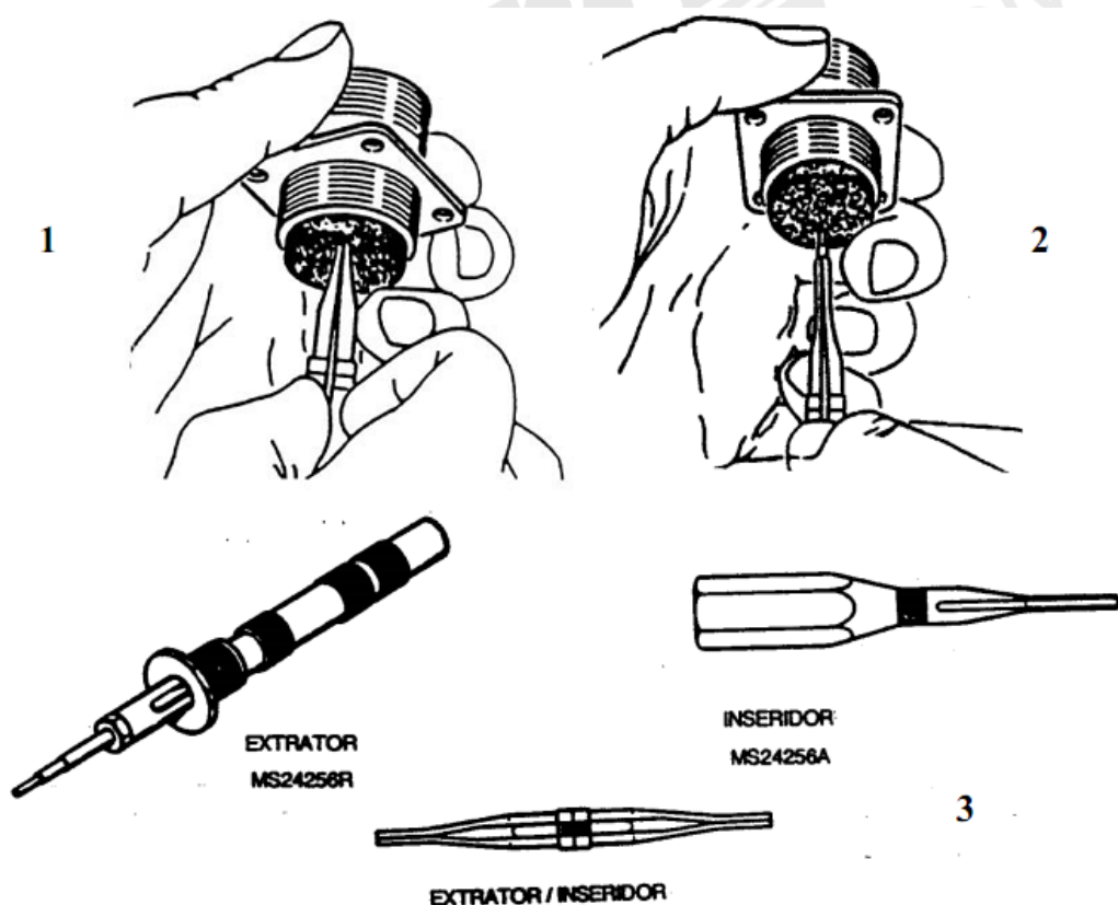
Figura 6-47 Remoção de pinos de contato
