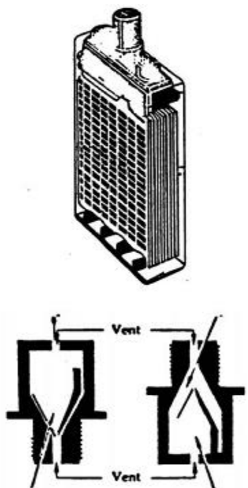
Figura 6-105 Grupo de placas e bujões de respiro
