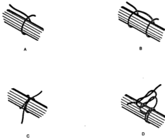
Figura 6-15 Amarração com nó simples
