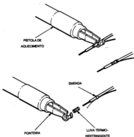
Figura 6-38 Ferramentas para instalação de terminais e emendas
