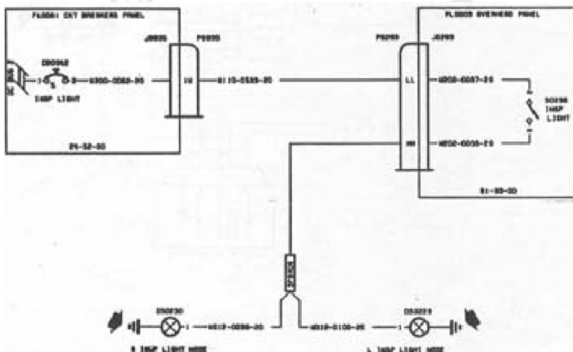
Figura 6 -77 Diagrama do circuito de aterramento por parafuso
