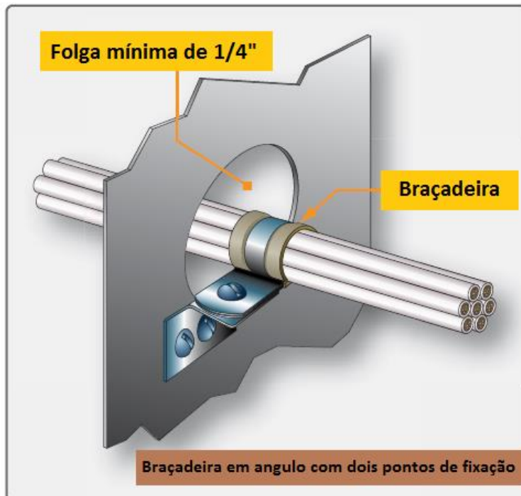
Figura 6-22 Braçadeira de cabo no orifício do anteparo
