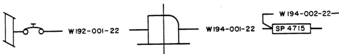
Figura 6-11 Modificação após "splices"
