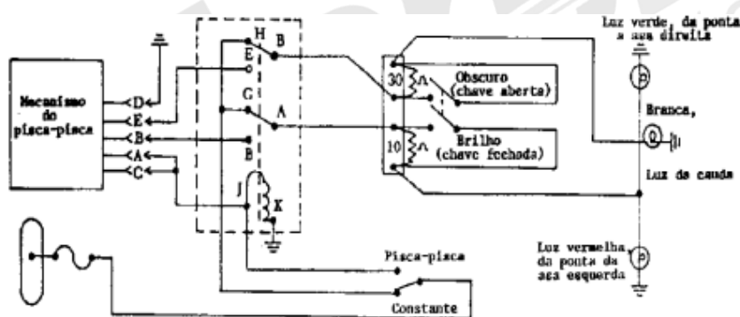
Figura 6-90 Circuito das luzes de posição
