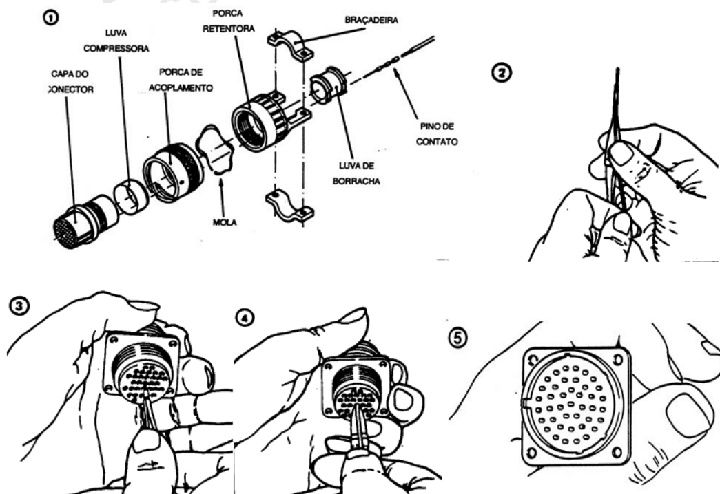
Figura 6-46 Instalação de pinos de contato prensados
