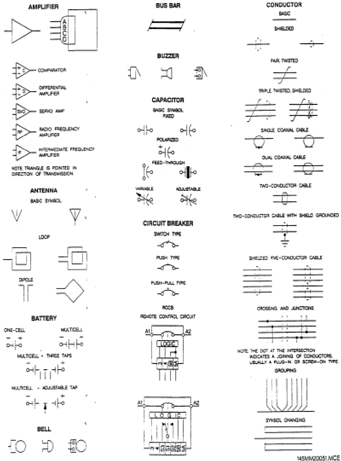
Figura 6-119 Símbolos elétricos VI
