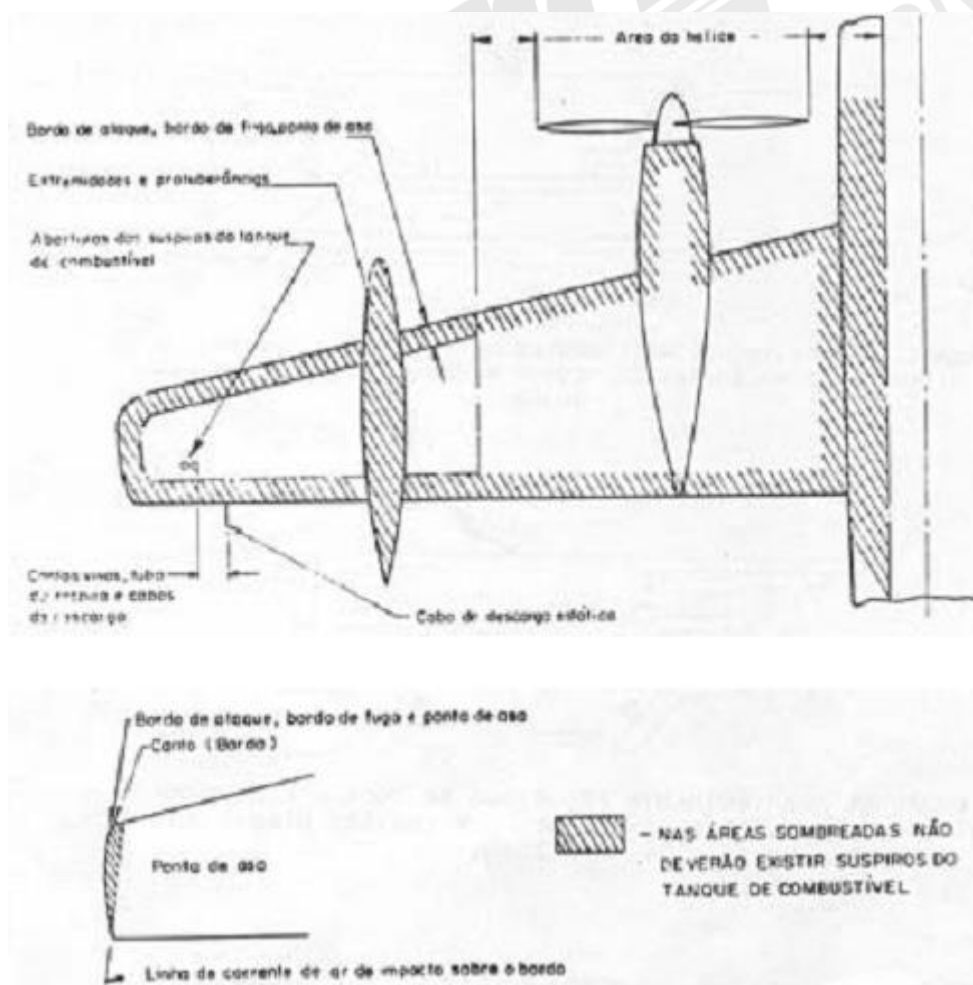
Figura 6-72 Zonas onde não deverão ser instalados suspiros de tanques de combustível.
