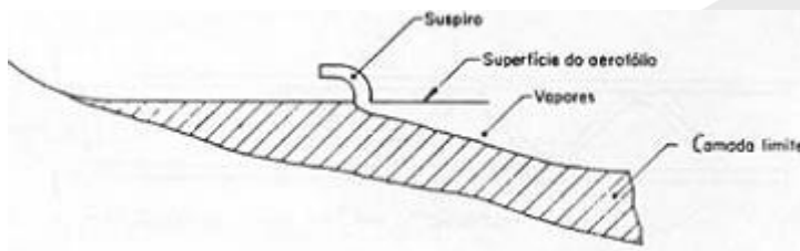
Figura 6-69 Saída do suspiro de combustível - Classe 3
