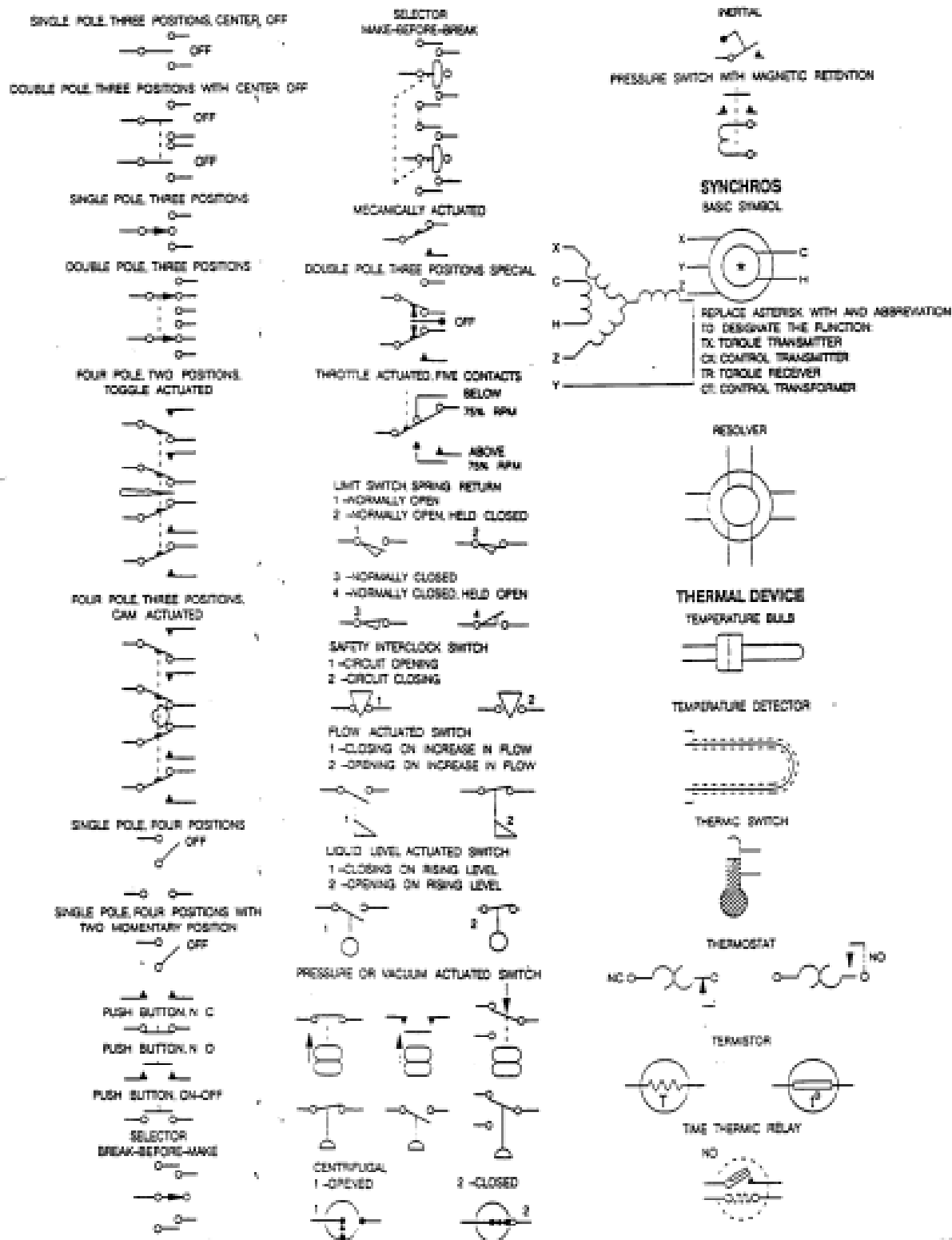
Figura 6-122 Símbolos elétricos IX
