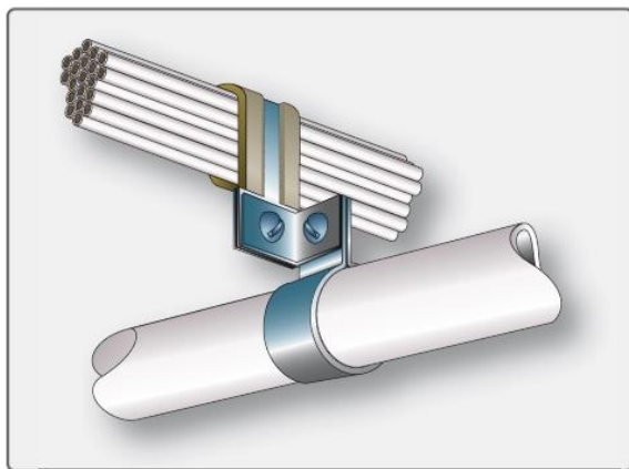
Figura 6-25 Separação entre a fiação e a tubulação
