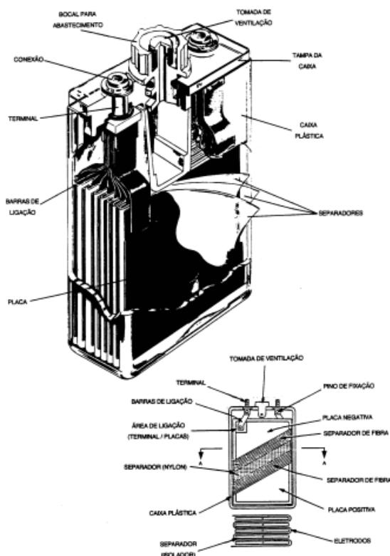
Figura 6-108 Elemento de bateria níquel-cádmio
