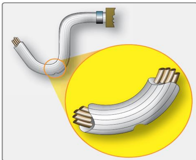
Figura 6-24 Orifício de dreno no ponto mais baixo da tubulação
