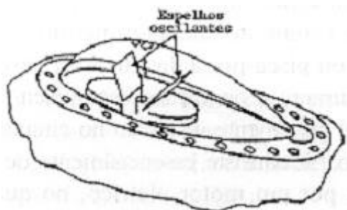
Figura 6-94 Luz de anticolisão
