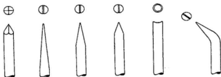
Figura 6-54 Formatos de pontas de ferro de soldar
