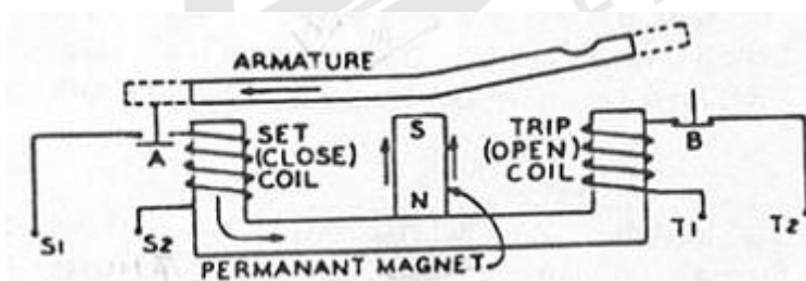
Figura 6-82 Representação simplificada do RCCB
