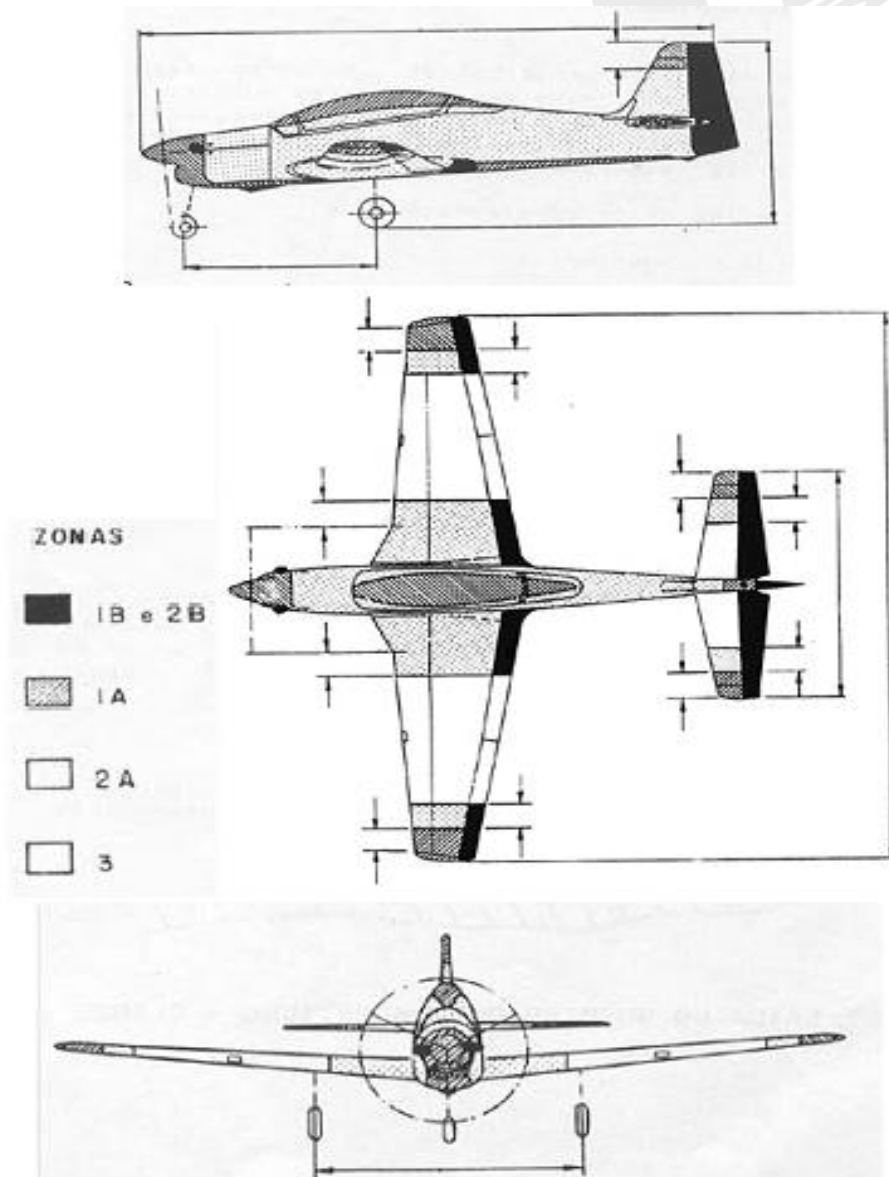
Figura 6-66 Designação típica das zonas sujeitas a descargas elétricas atmosféricas
