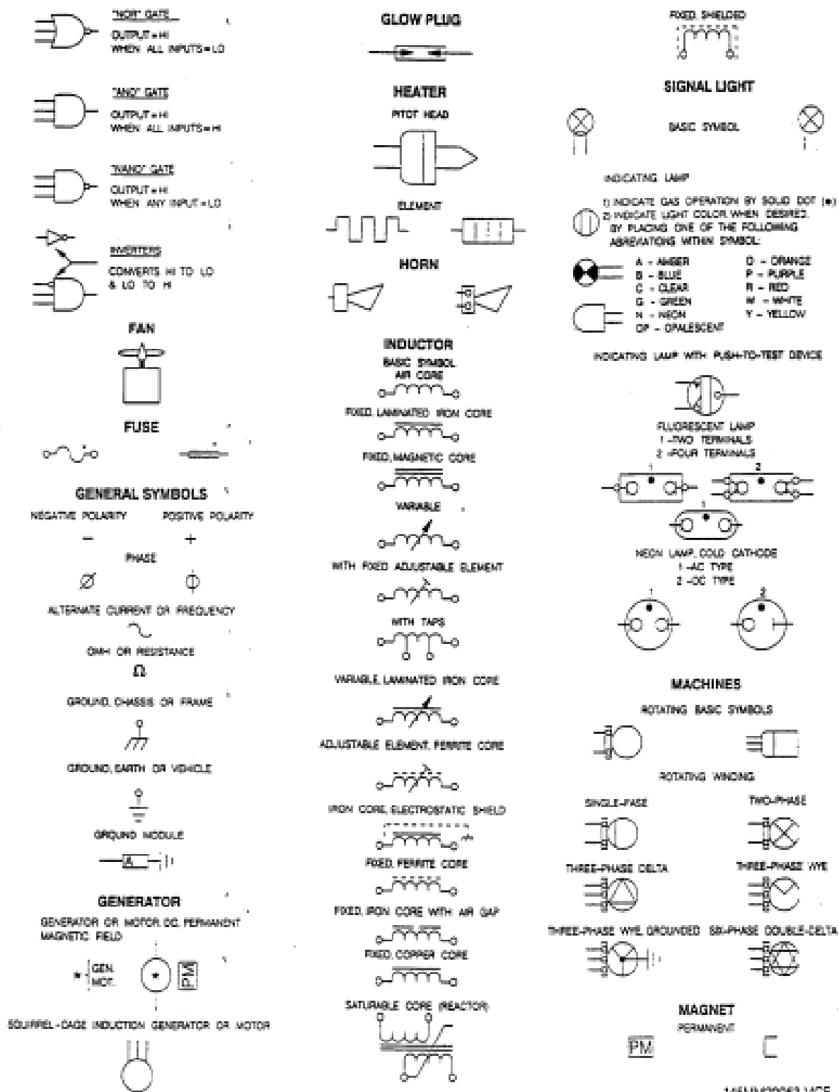
Figura 6-121 Símbolos elétricos VIII
