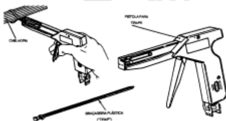
Figura 6-35 Diversas ferramentas para manutenção elétrica
