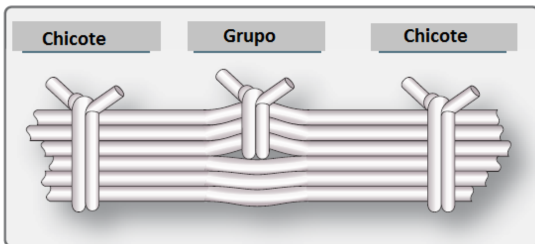
Figura 6-13 Amarrações de grupo de fios e chicotes
