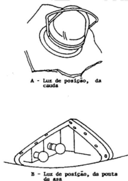
Figura 6-89 luzes de posição
