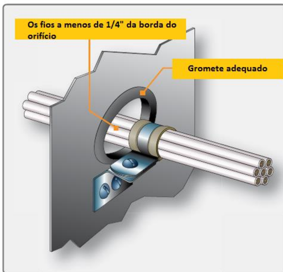
Figura 6-23 Braçadeira de cabo com gromete ilhós
