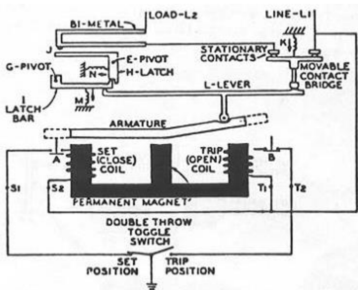
Figura 6-82 Representação simplificada do RCCB
