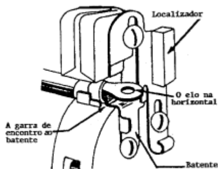
Figura 6-40 Colocação do terminal na ferramenta manual
