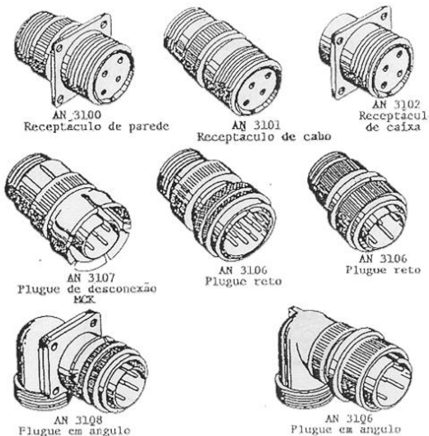
Figura 6 -29 Conectores AN
