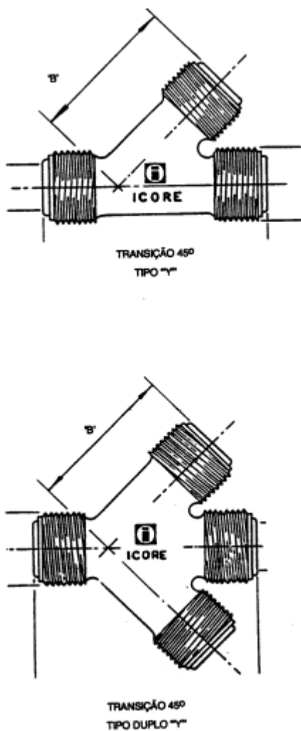
Figura 6-32 Derivações tipo "Y" e duplo "Y"
