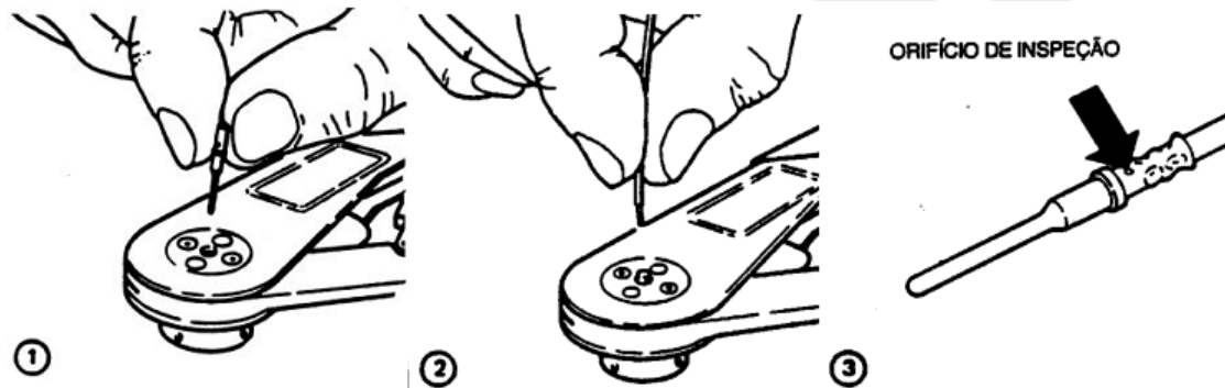
Figura 6-45 Prensagem de pinos de contato
