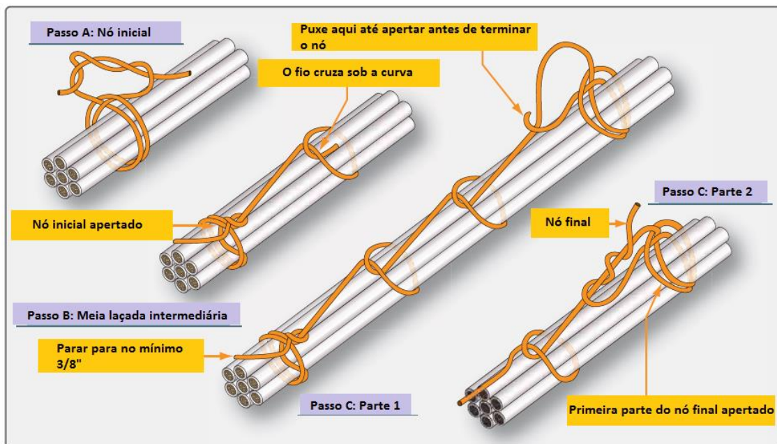
Figura 6-17 Amarração contínua iniciada com nó simples
