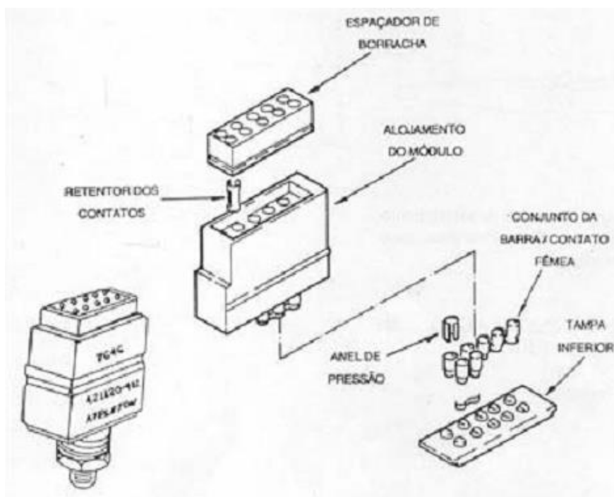
Figura 6-79 Módulo de aterramento
