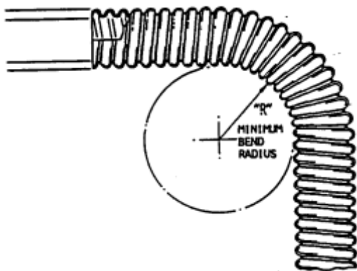
Figura 6-31 Conduíte transparente
