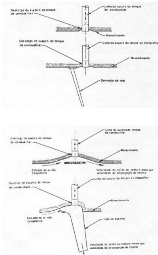
Figura 6-71 Proteção nas saídas dos suspiros de combustível
