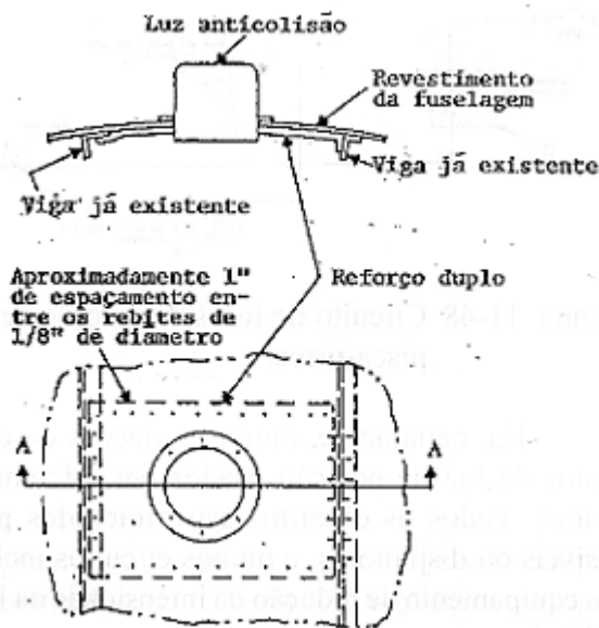
Figura 6-92 Instalação típica da luz de anticolisão num painel de revestimento não pressurizado.
