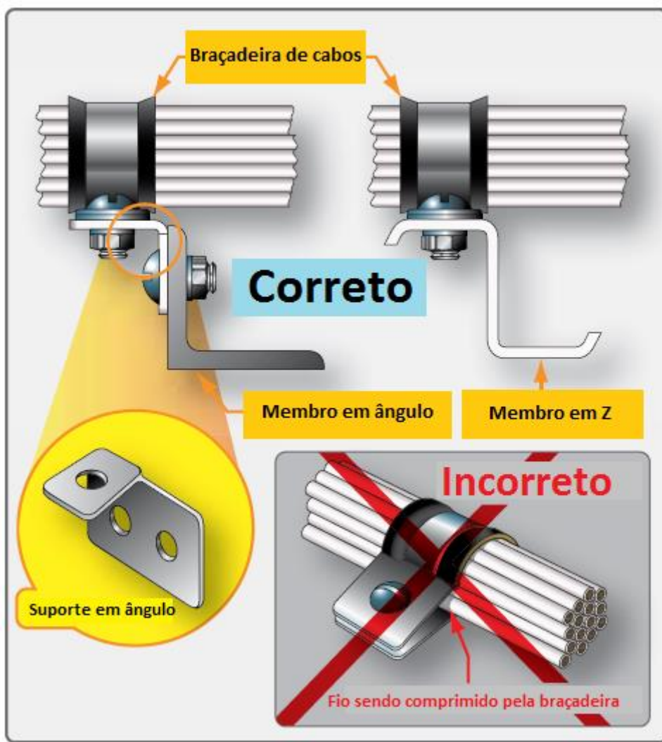
Figura 6-28 Montagem da braçadeira de cabo na estrutura
