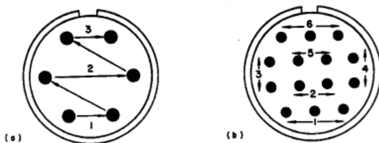
Figura 6-64 Sequência para a soldagem de pinos
