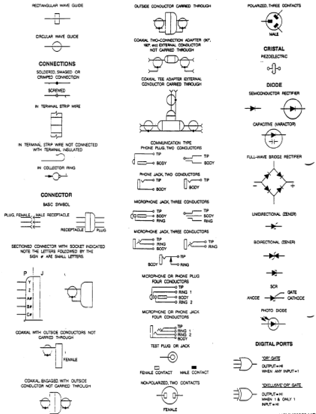
Figura 6-120 Símbolos elétricos VII
