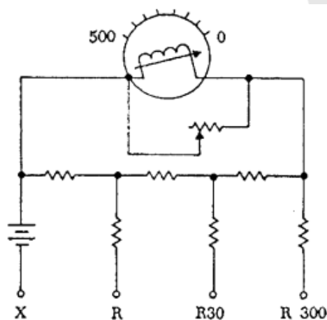
Figura 6-101 Circuito interno típico de um ohmímetro
