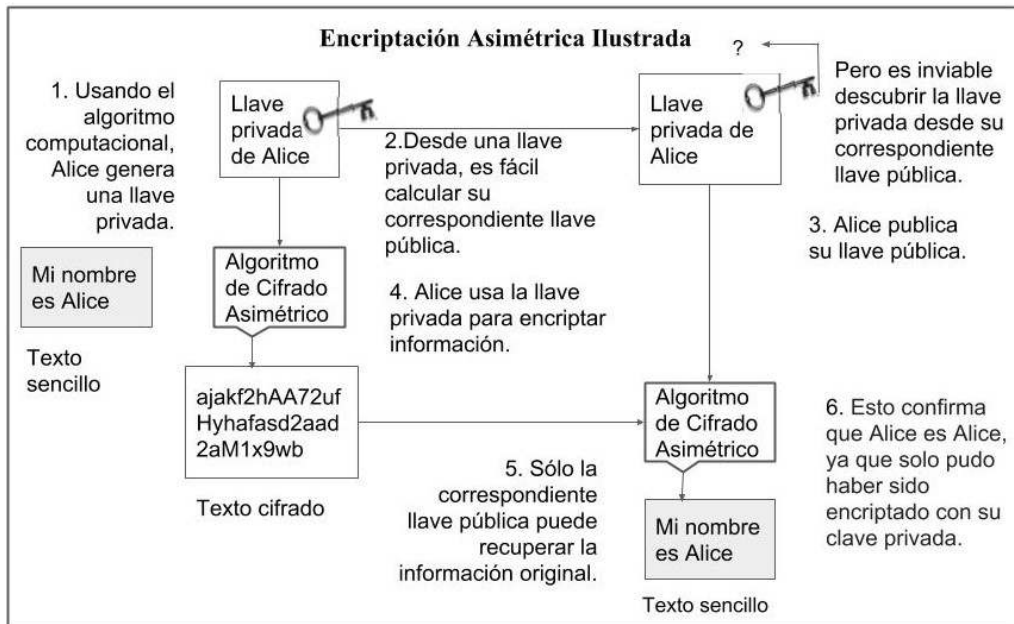
FIGURA 2: ENCRIPCIÓN ASIMÉTRICA ILUSTRADA
