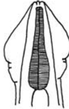
Toxocara cati ( T. mystax )
