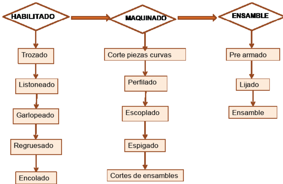
Gráfico 3 Operaciones de la carpintería en madera
