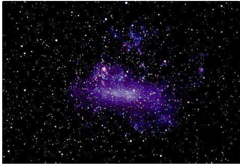
Figura 26.4: A Grande Nuvem de Magalhães, uma galáxia irregular.
