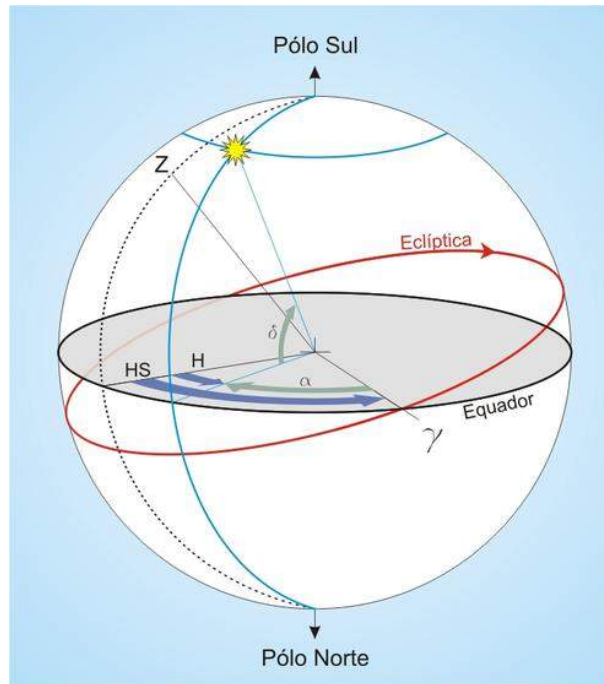
Figura 3.4: O ângulo horário ( H ) é o ângulo entre o meridiano local (linha pontilhada) e o meridiano do astro (linha azul), contado no sentido do movimento diurno. O ângulo horário do astro somado à sua ascensão reta ( \alpha ), define a hora sideral ( HS ).
