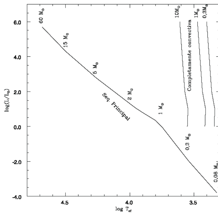
Figura 23.28: Sequência principal e zona completamente convectiva
