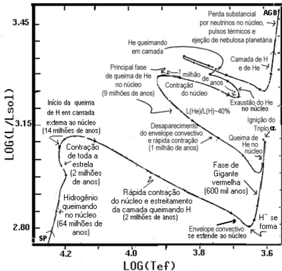
Figura 22.13: Diagrama HR teórico mostrando as diversas fases da evolução de uma estrela de 5 massas solares, a partir da sequência principal (SP), no extremo esquerdo inferior e, quanto tempo a estrela leva em cada fase, segundo os cálculos de Icko Iben Jr. (1931-).
