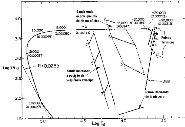
Figura 23.46: Diagrama HR teórico mostrando o caminho evolucionário de uma estrela de 0,6 M_{\odot} , a partir do Ramo Horizontal, calculado pelo americano Icko Iben Jr. e pelo italiano Alvio Renzini. O ramo horizontal é onde as estrelas queimam He no núcleo. As estrelas com massa até cerca de 6 M_{\odot} chegam ao ramo horizontal com um núcleo com, aproximadamente, 0,6 M_{\odot} . Posteriormente, perdem suas camadas superiores por perda de massa contínua, como vento solar e ejeção de nebulosa planetária. Os tempos indicados em cada ponto, positivos e negativos, são medidos em anos a partir de um ponto, no caminho, com T_{\text{ef}} = 35\,000 K.
