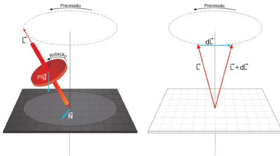
Figura 13.6: Em um pêlo, o peso ( m\vec{g} ) provoca um torque ( \vec{N} ) perpendicular ao momentum angular do pêlo ( \vec{L} ), o qual causa uma variação ( d\vec{L} ) no momentum angular, perpendicular a ( \vec{L} ), que altera sua direção sem alterar seu módulo.
