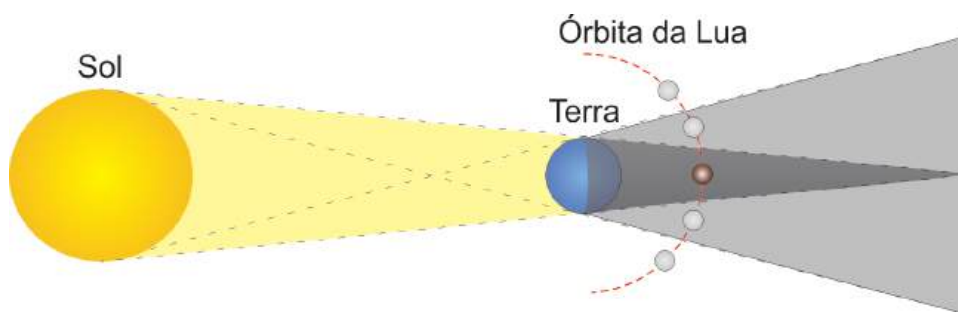
Figura 8.5: Diagrama de um eclipse lunar. A umbra da Terra, à distância em que é cruzada pela Lua, tem um diâmetro de aproximadamente 2,5 vezes o diâmetro da Lua.
