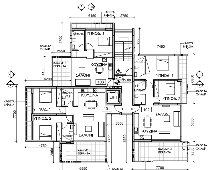
ΚΑΤΩΦΗ 1ΟΥ ΟΡΟΦΟΥ ΚΛΙΜΑΚΑ 1:200
