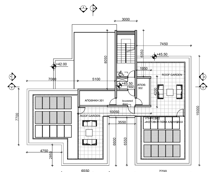
ΚΑΤΩΦΗ 4ΟΥ ΟΡΟΦΟΥ ΚΛΙΜΑΚΑ 1:200
