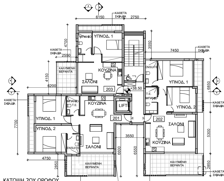
ΚΑΤΩΦΗ 2ΟΥ ΟΡΟΦΟΥ ΚΛΙΜΑΚΑ 1:200
