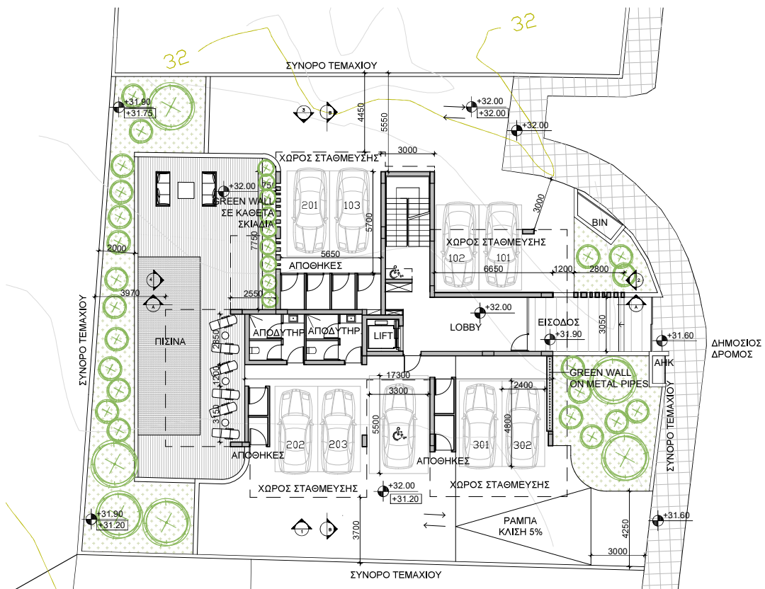
ΧΩΡΟΤΑΞΙΚΟ - ΚΑΤΟΨΗ ΙΣΟΓΕΙΟΥ (ΠΥΛΩΤΗ) ΚΛΙΜΑΚΑ 1:200
