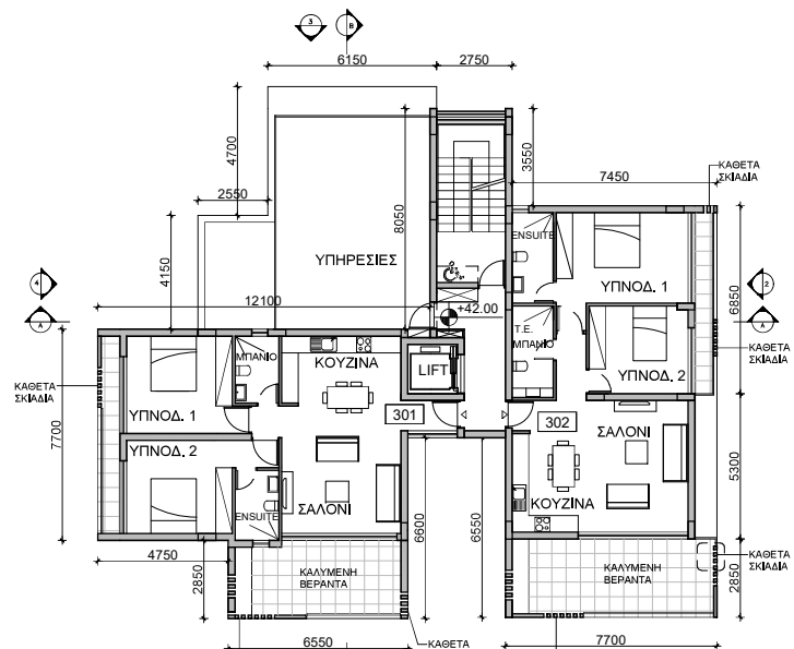
ΚΑΤΩΦΗ 3ΟΥ ΟΡΟΦΟΥ ΚΛΙΜΑΚΑ 1:200
