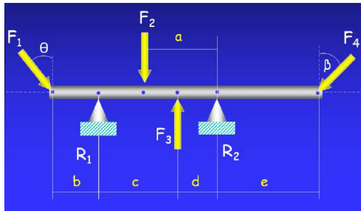
3.5.3 Esquema de fuerzas de problema
