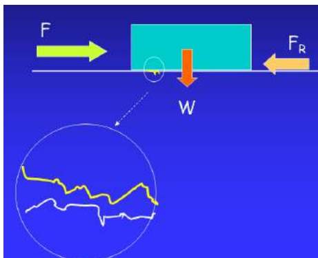
3.5.4 Roce estático
