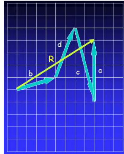
Figura 3.3.11 Resultante de la suma
