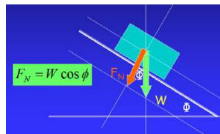
3.5.5 Roce estático inclinado
