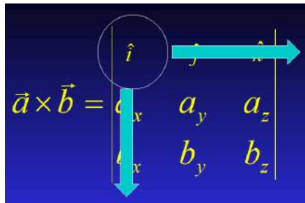
Figura 3.3.19 Nemotecnia del determinante
