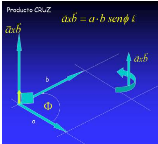
Figura 3.3.17 Producto cruz
