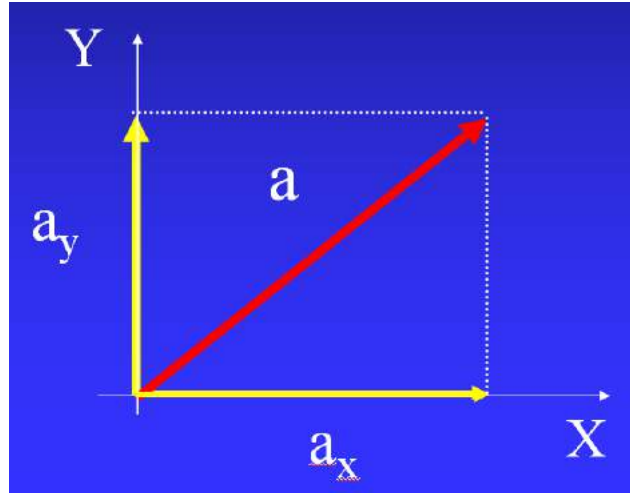
Figura 3.3.3 Gráfica cartesiana
