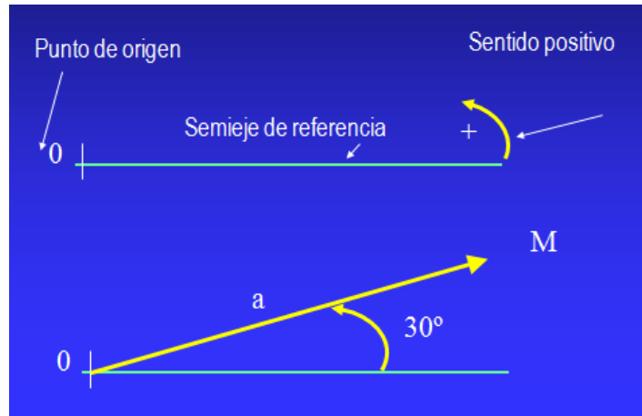
Figura 3.3.2 Gráfica polar
