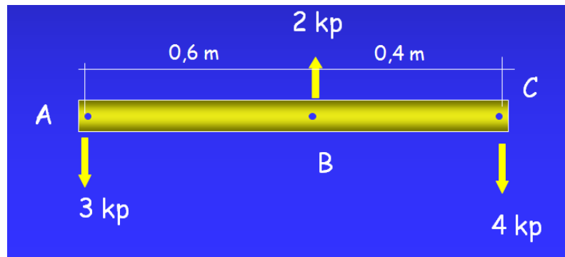
3.5.2 Esquema de fuerzas
