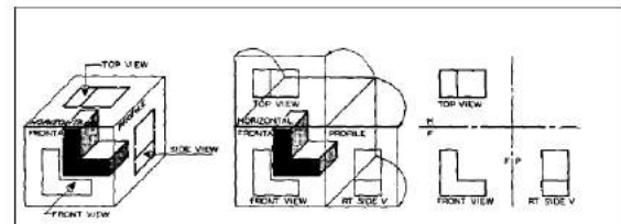
Figura 5.8 Ejemplo de proyecciones
