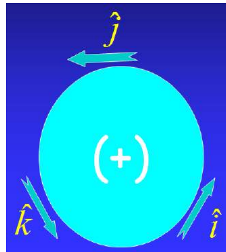
Figura 3.3.18 Nemotecnia del producto cruz
