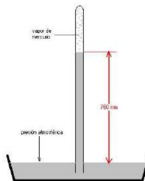
Figura 3.4 Presión atmosférica
