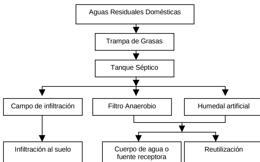
Figura 6.8.1 Tratamiento de las aguas residuales domésticas de baterías sanitarias y casinos
