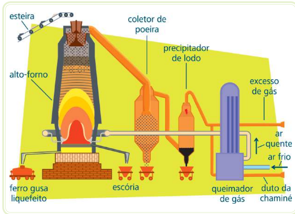
Figura 1.3: Alto forno Fonte: CTISM
