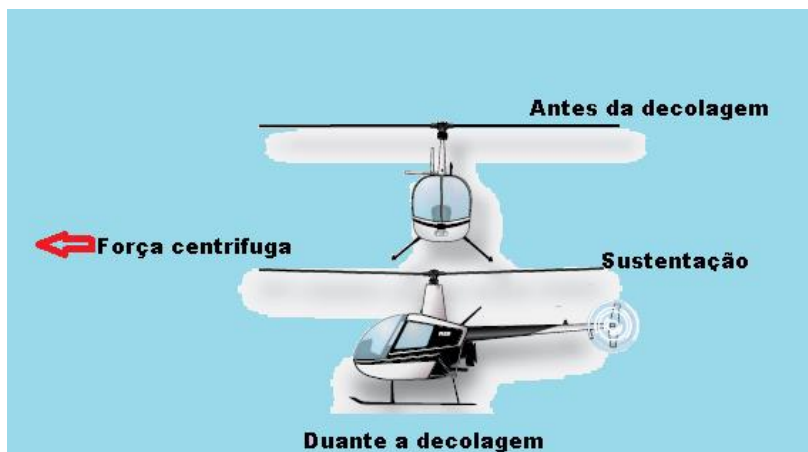
Figura 13-41 Cone nas pás.
