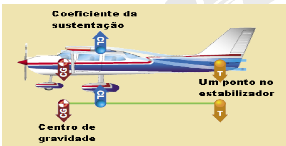
Figura 13-12 Sustentação na empenagem.
