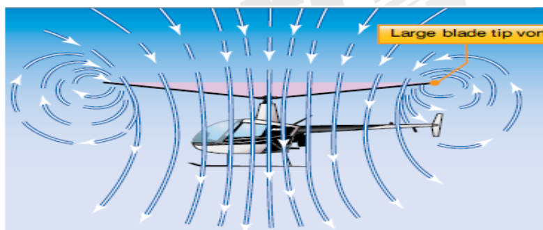
Figura 13-42 Efeito de solo.
