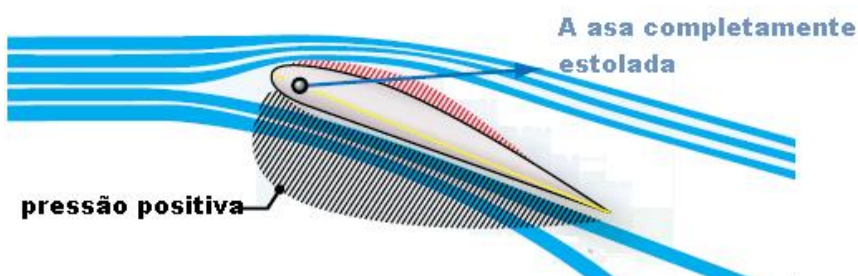
Figura 13-5 Efeito do aumento do ângulo de ataque.
