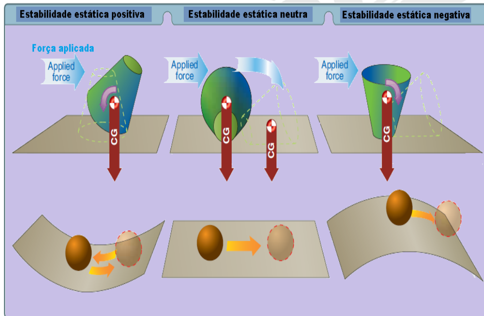
Fonte: FAA - Mechanic Training Handbook-Airframe Figura 13-11 – Estabilidade estática.
