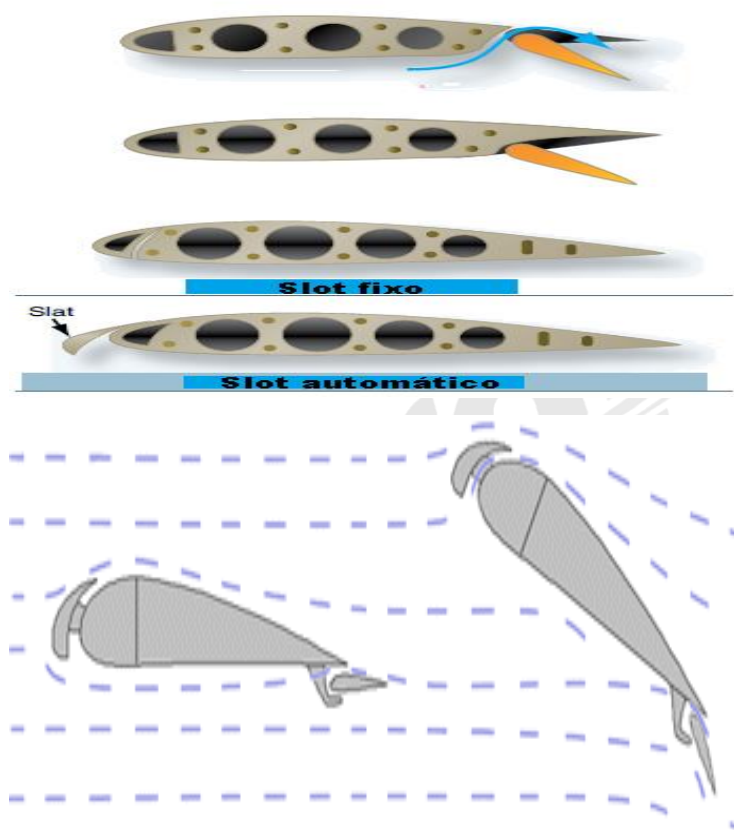
Figura 13-29 Dispositivos de hipersustentação.
