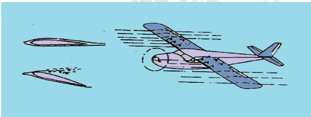
Figura 13-21 Spoileres fixos.
