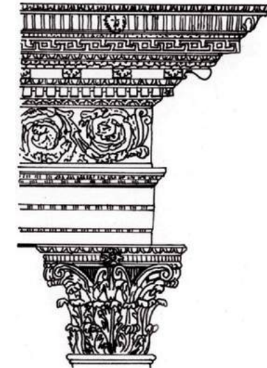
Coríntio (Nîmes, a Maison Carrée)
