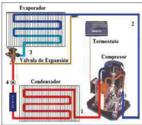
Fig. 1. Sistema de Refrigeración
