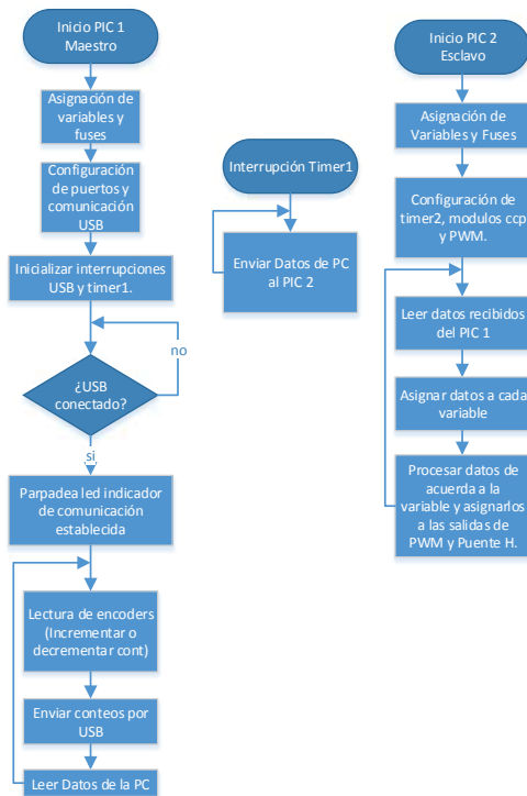
Fig. 3 Diagrama de flujo general que muestra los procesos principales del programa desarrollado.
