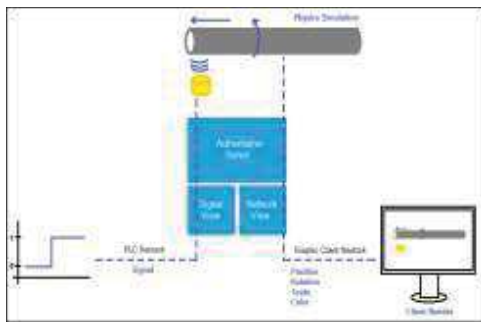
Fig. 2. Mecanismos independientes en el Sistema de mensajes para la red de PLC y los clientes gráficos.
