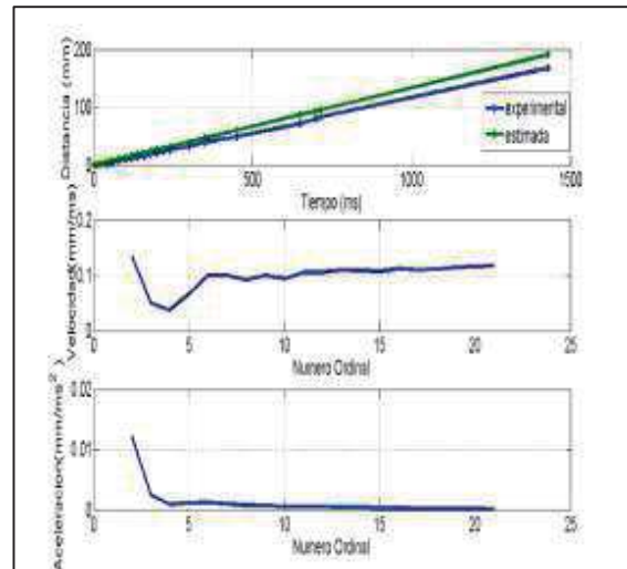
Figura 9. Grafica de posiciones, velocidades y aceleraciones.
