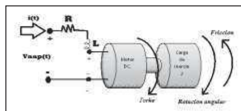
Fig. 3. Motor DC
