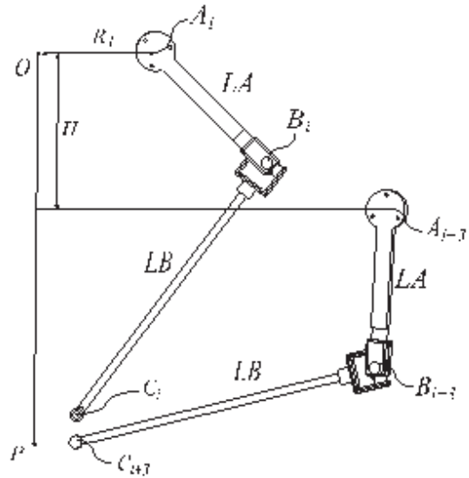
Fig. 2. Representación de la i e i+3 -ésima cadena cinemática del robot de paralelo de 6 GDL.
