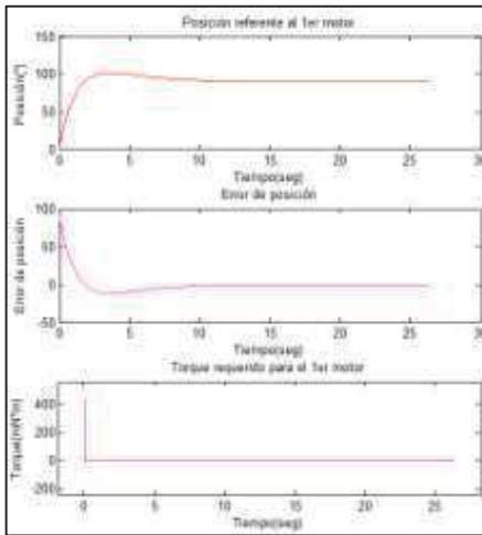
Fig. 7. Posición, error de posición y torque (base)
