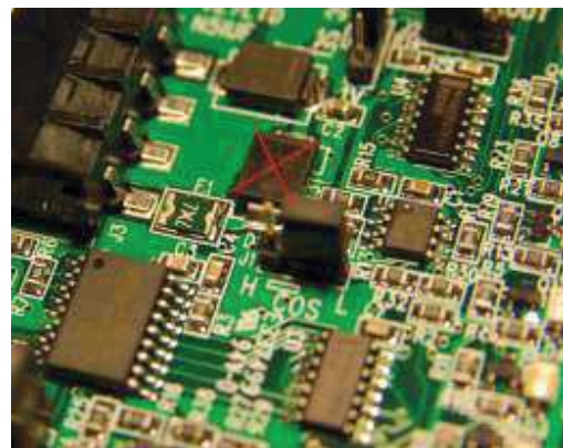
Figura 4. Remoción del diodo rectificador.
