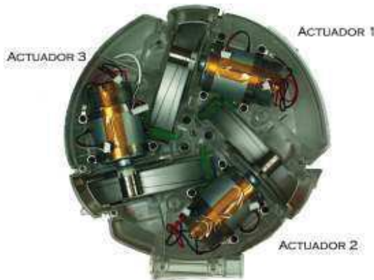
Fig. 2. Actuadores del Novint Falcon
