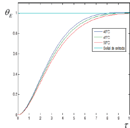
Fig. 8. Respuesta de la planta con retroalimentación unitaria.
