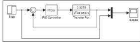
Fig. 9. Sistema del controlador PID y la planta
