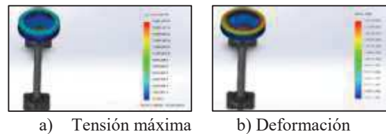
Figura 13. Estudio de tensión y deformación máxima del plato centrifugador.
