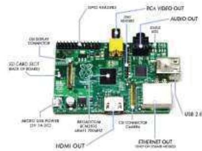
Fig. 8. Plataforma de cómputo Raspberry Pi
