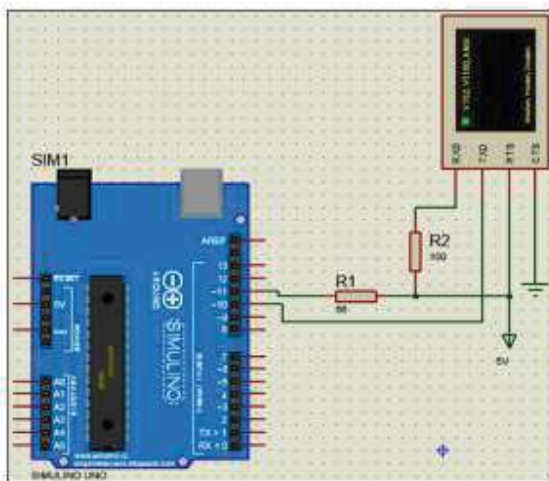
Fig. 7. Circuito de comunicación.
