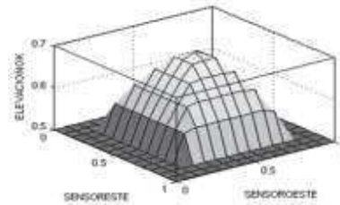
Fig. 10. Gráfico de salida de los sensores Este y Oeste con respecto a la salida Elevación OK
