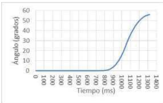
Fig. 11 Posicionamiento angular del Fémur con señal A.
