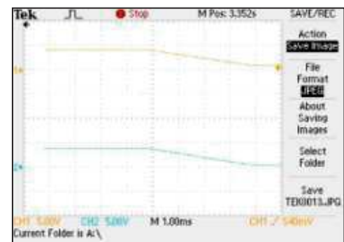
Figura 6. Transición de nivel alto a bajo al girar
