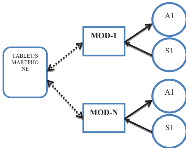
Fig. 4 Arquitectura implementada para el sistema de medición de energía eléctrica
