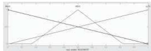
Fig. 6. Conjunto difuso de entrada Sensor-Este.
