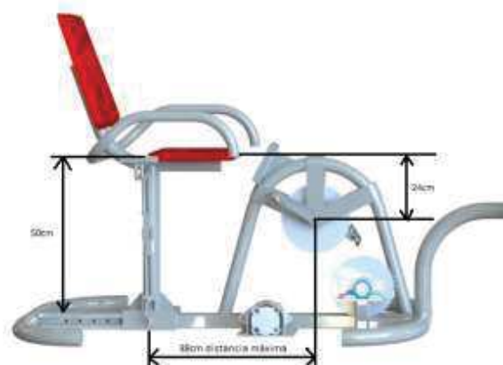
Fig. 2 Diseño funcional de la bicicleta horizontal
