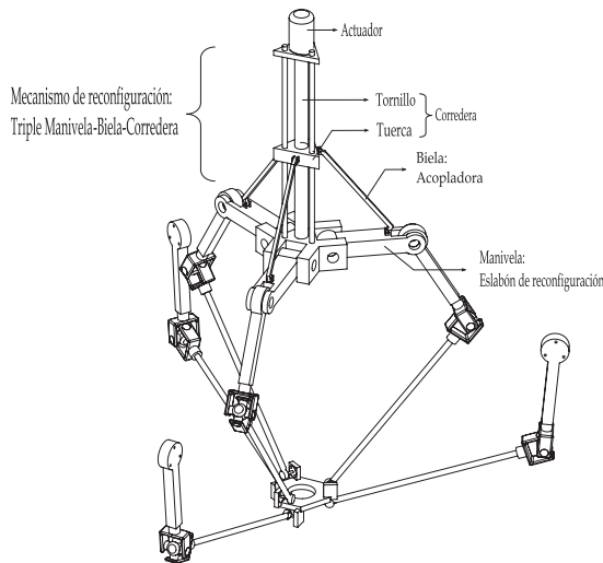
Fig. 6. Propuesta de diseño conceptual para el robot paralelo reconfigurable.
