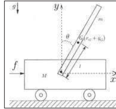
Fig. 1. Péndulo invertido sobre un carro.
