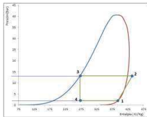
Fig. 3. Grafica Presión – Entalpía del HFC-134a
