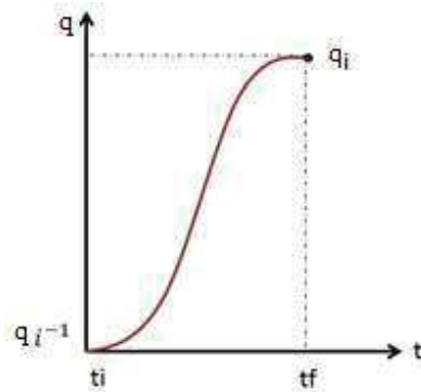
Fig. 3. Trayectoria con interpolación cúbica
