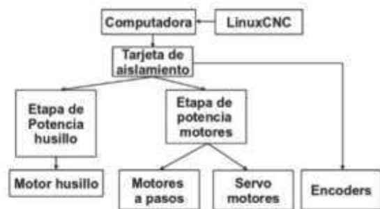
Fig. 6. Componentes requeridos para la implementación básica de LinuxCNC en una máquina herramienta.
