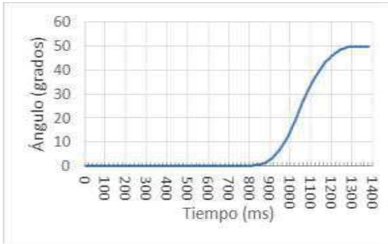
Fig. 9 Posicionamiento angular de la tibia con señal A.
