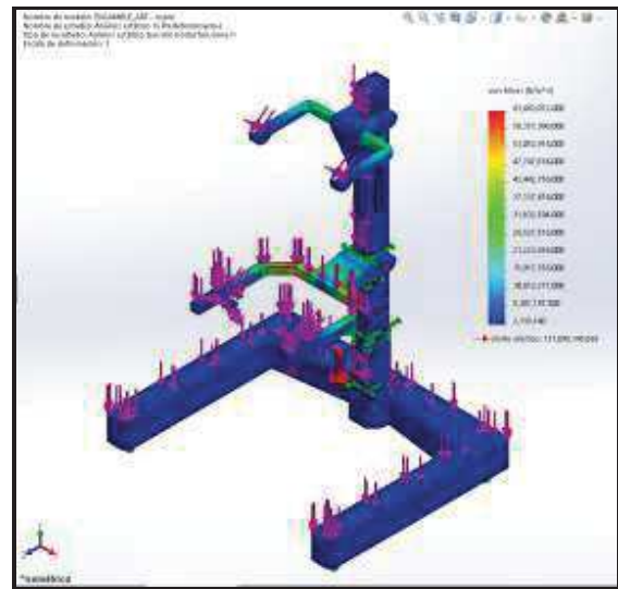
Figura 7: Análisis de deformación obtenido del soporte parcial de peso.
