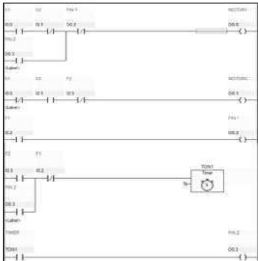
Fig. 3. Diagrama escalera.
