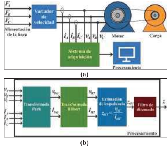
Fig. 1. a) Metodología para la medición de parámetros. b) Metodología para la estimación de impedancia.
