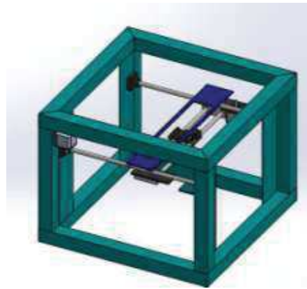
Fig. 5. Modelado en sólidos del robot cartesiano.
