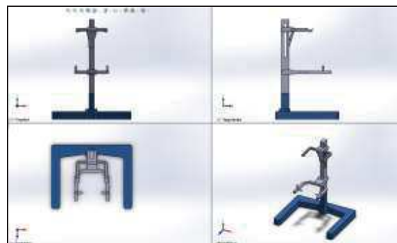
Figura 8: Diferentes vistas del Soporte Mecánico Parcial para Fisioterapia.
