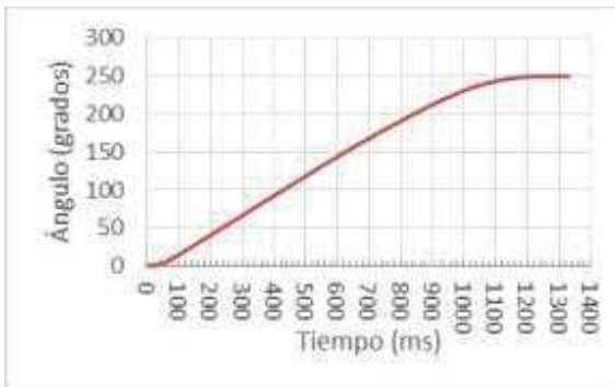
Fig. 10 Posicionamiento angular de la tibia con señal B.
