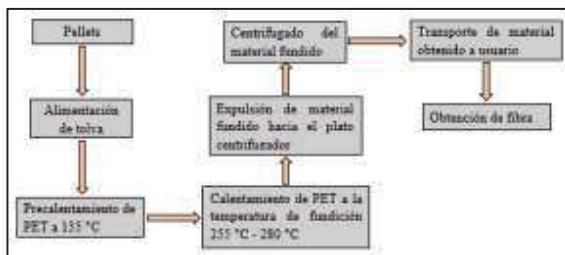
Figura 1. Cuadro de proceso realizado por la máquina.
