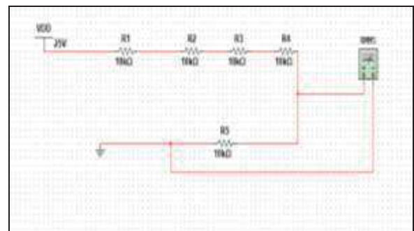
Fig. 2. Divisor de voltaje.
