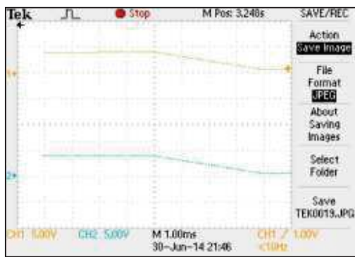
Figura 8. Transición de alto a Bajo lineal
