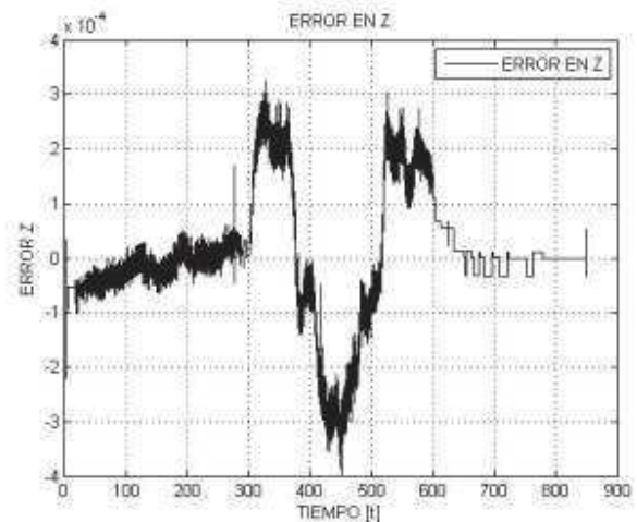
Fig. 11. Error en el eje Z.
