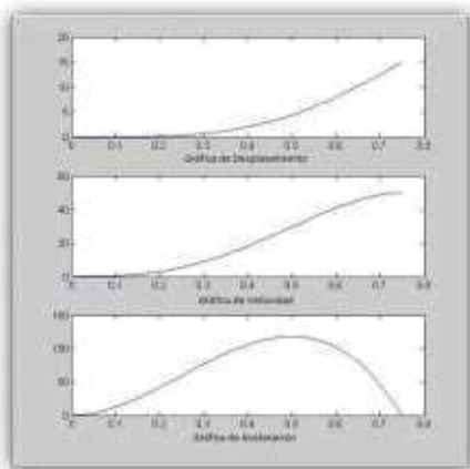
Fig. 4. Perfiles de trayectoria suavizados en MatLAB.
