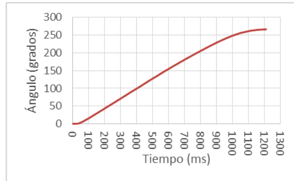
Fig. 12 Posicionamiento angular de Fémur con señal B.
