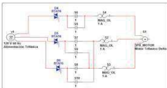
Fig. 10. Circuito de conexión del motor trifásico.
