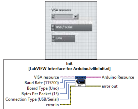
Fig.6. Interfaz gráfica en la que se muestra la comunicación con Arduino.
