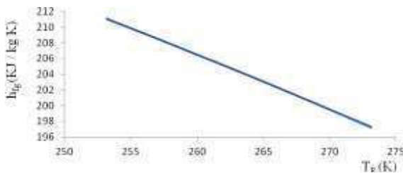
Fig.6. Regresión h_{fg}(T_R) = -0.6906 T_R + 386.01
