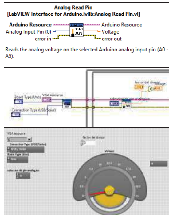
Fig.7 Componentes del lector de una entrada analógica.
