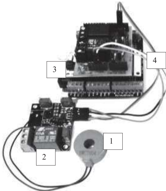
Fig. 6 Modulo inalámbrico con sensor de corriente y actuadores
