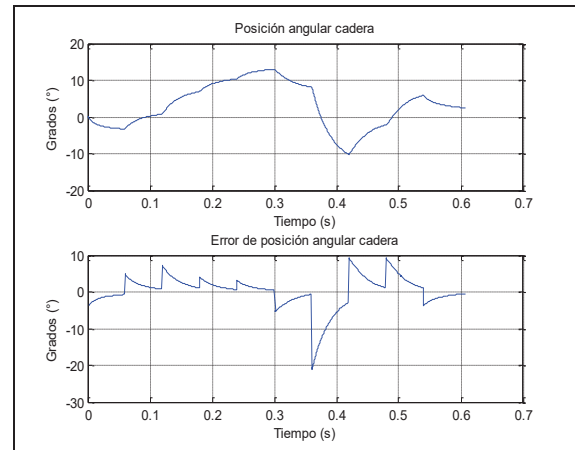
Fig. 11. Posición angular de salida y señal de error en el tobillo
