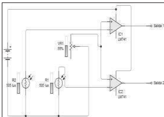
Fig. 4. Comparador analógico.
