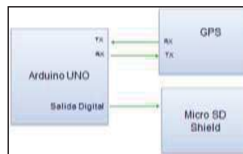
Fig. 8. Diagrama de bloques para el control de los sistemas GPS y Micro SD.
