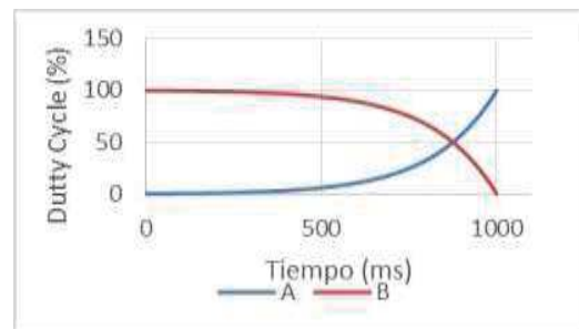
Fig. 8 Señales de aceleración aplicadas a cada motor en la articulación tibia-fémur.
