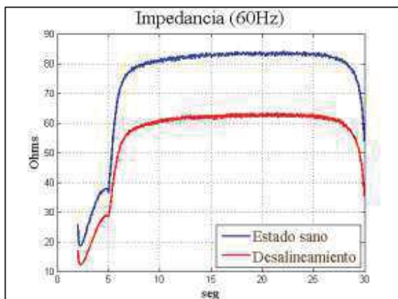
Fig. 7. Envolvente de impedancia de motor a 60Hz.
