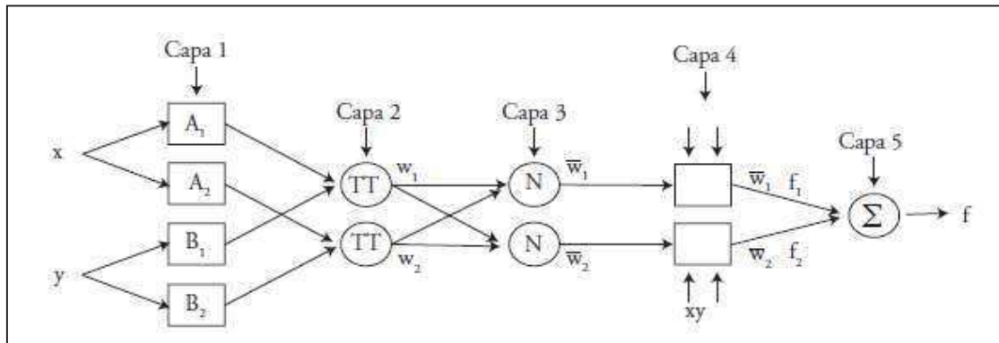
Fig. 2. Arquitectura ANFIS.
