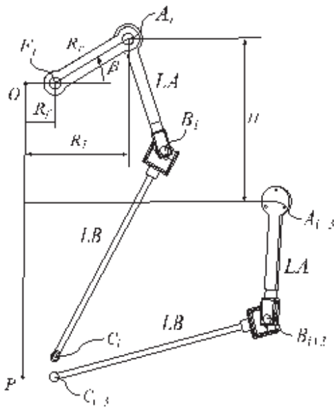
Fig. 3. Estrategia de reconfiguración basada en la variación simultánea de R_i y H .
