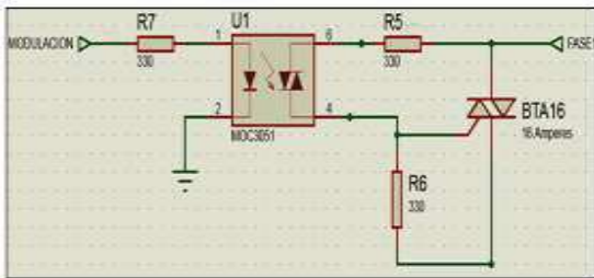
Fig. 9. Circuito de aislamiento entre el microcontrolador y la potencia.
