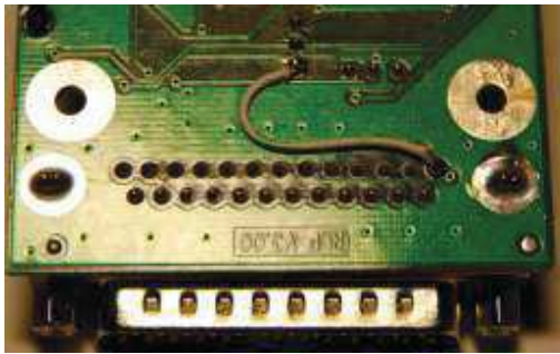
Figura 5. Puente para operación de la tarjeta IRLP a 3.3 Volts.
