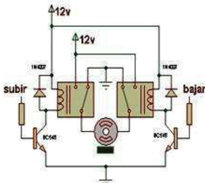
Fig. 5. Puente H.
