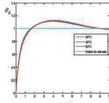
Fig. 10. Respuesta del controlador PID, con K_p=5 , K_i=2 y K_d=6.9
