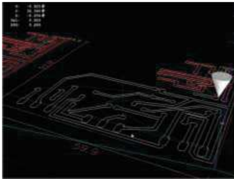
Fig. 7. Simulación de fresado de tarjetas en LinuxCNC
