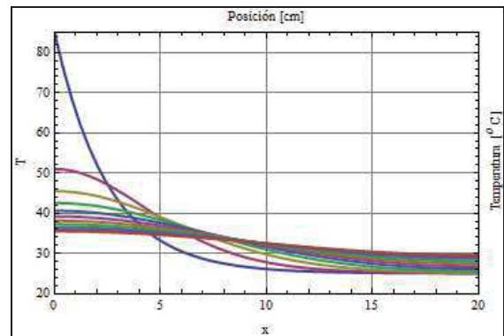
Fig. 3. Modelo de la Ecuación del Calor, Distribución de Temperatura vs. Posición para varios tiempos.
