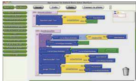
Fig. 7. Editor de bloques de App inventor.
