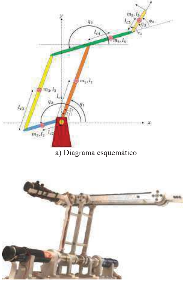
Figura 1. Manipulador Paralelo de 3 G.D.L.
