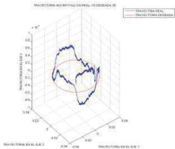
Fig. 5. Grafica de trayectorias en 3d
