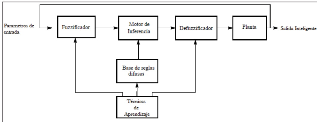
Fig. 1. Arquitectura de un controlador Neurodifuso.
