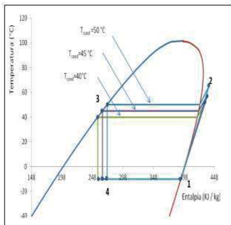
Fig.4. Grafica Temperatura – Entalpía, del HFC-134a.
