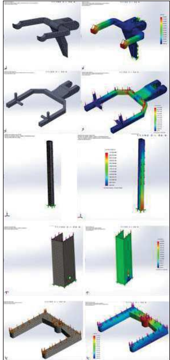
Figura 5: Mallado y análisis de deformación aplicado a cada una de las piezas que conforman el soporte parcial de peso.
