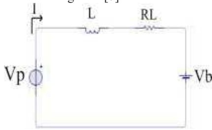
Fig. 1. Circuito de Carga de Batería con el Panel Solar.
