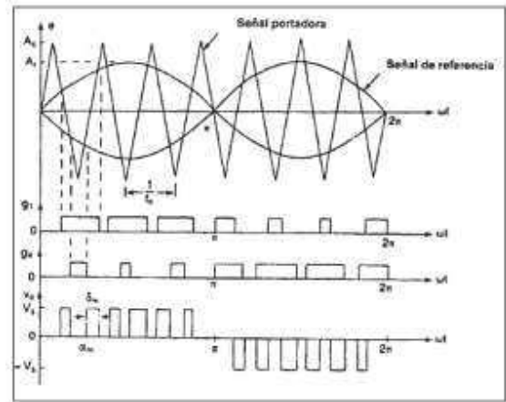
Fig. 8. Modulación de ancho de pulso sinusoidal.
