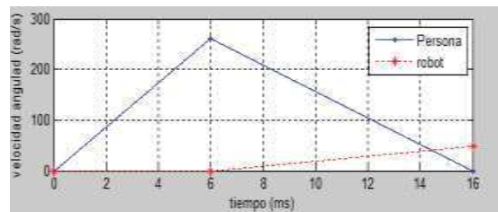
Figura 11 Gráfica de comparación velocidad 3.
