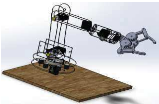
Fig.4. Ensamble mecánico del robot 5 GDL en Solidworks
