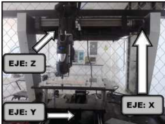
Fig. 3. Prototipo de robot cartesiano
