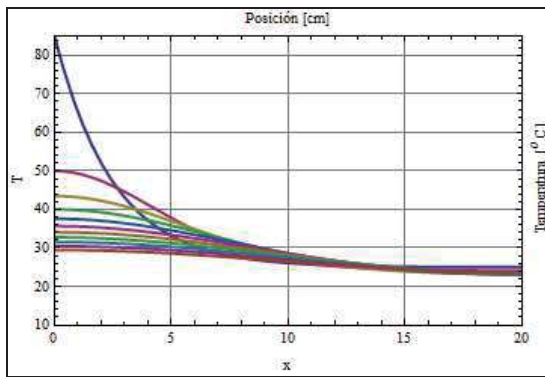
Fig. 8. Modelo de la Ecuación del Calor Modificado.
