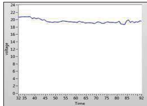
Fig.14. Gráfica de datos correspondientes a la tabla 1 que fueron obtenidos el 21 de mayo del 2014 mediante el sistema de adquisición desarrollado en LabVIEW.
