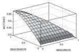
Fig. 9. Gráfico de salida de los sensores Este y Oeste con respecto a la salida Motor EO
