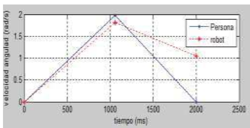
Figura 9 Comparación velocidad 1 (velocidad lenta).
