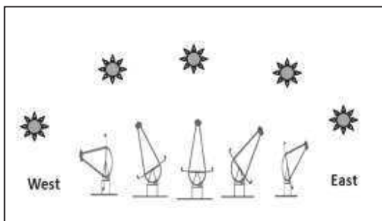
Fig. 1. Seguimiento solar.
