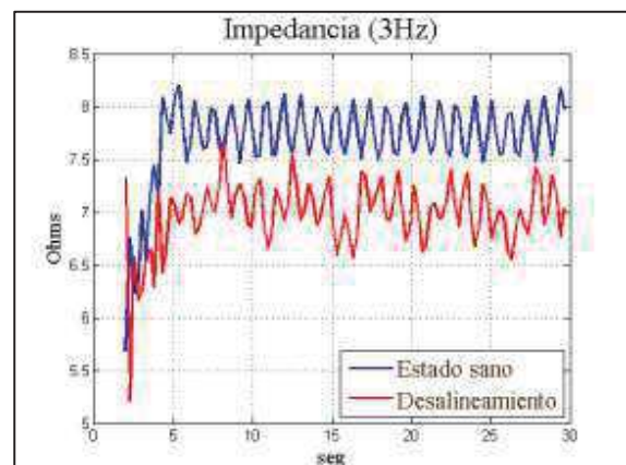
Fig. 5. Envolvente de impedancia de motor a 3Hz.
