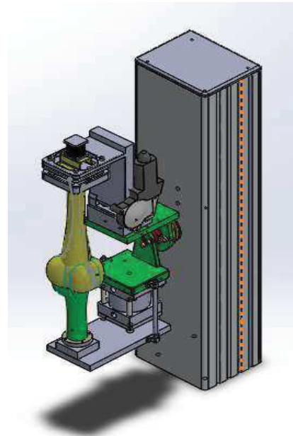
Fig. 1 Prototipo de rodilla para pruebas de meniscos sintéticos con movimientos complejos.
