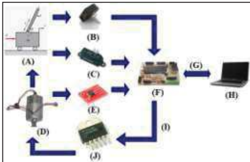
Fig. 2. Diagrama funcional del prototipo.
