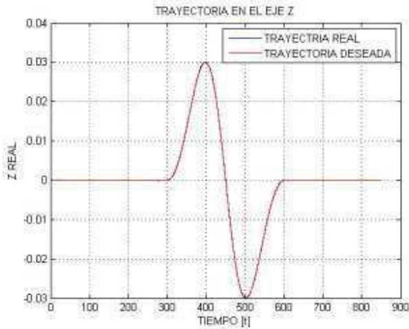
Fig. 8. Trayectoria en z real y deseada.
