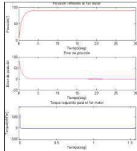
Fig. 4. Posición, error de posición y torque (base)
