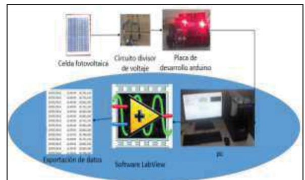
Fig.1. Diagrama a bloques del programa.
