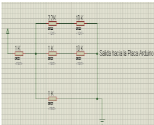
Fig. 3. Circuito de Acoplamiento de Señal
