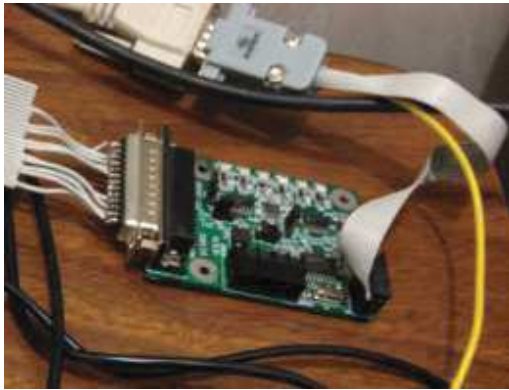
Figura 1. Nodo IRLP con interfaz para PC.
