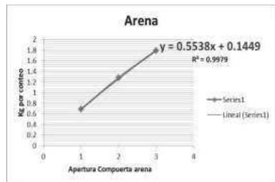
Figura 6. Gráfica kg de arena por apertura de compuerta
