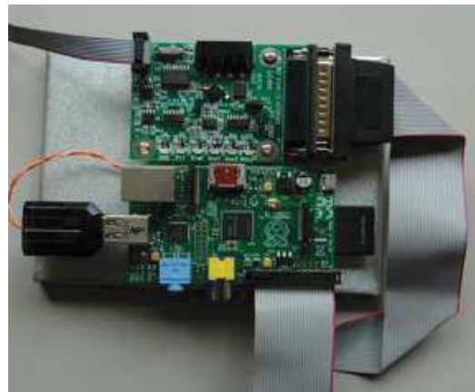
Figura 8. Nodo IRLP con microcomputadora Raspberry Pi.
