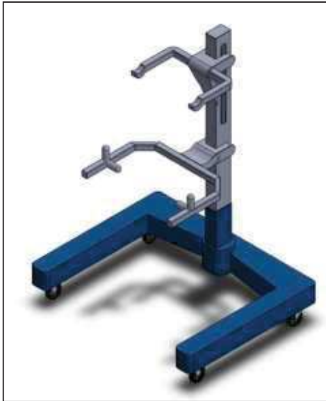
Figura 3: Diseño de la estructura mecánica del soporte parcial de peso.
