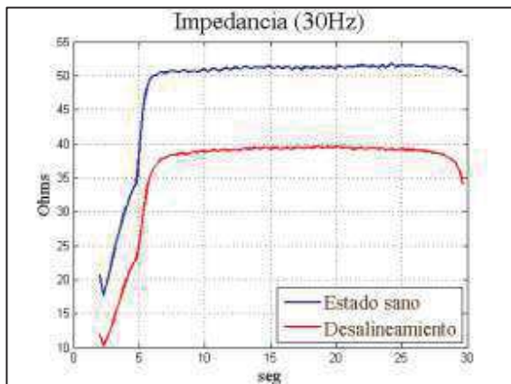
Fig. 6. Envolvente de impedancia de motor a 30Hz
