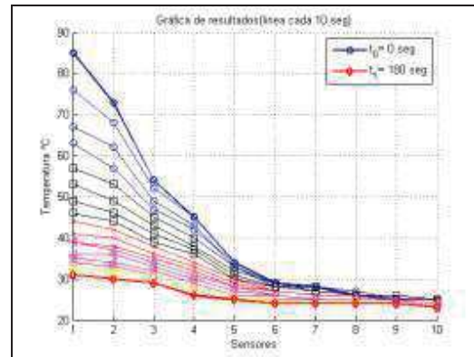
Fig. 7. Mediciones Experimentales para la Distribución del Calor.
