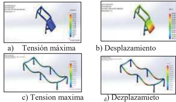
Figura 11. Estudio de tensiones y desplazamientos máximos en estructuras
