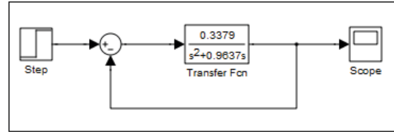
Fig. 7. Sistema con retroalimentación unitaria
