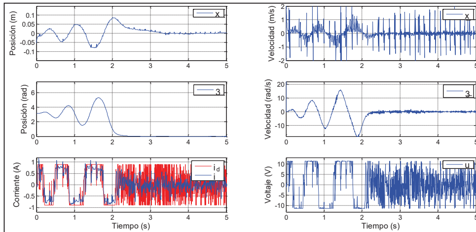
Fig. 4. Graficas de respuestas del PISC.
