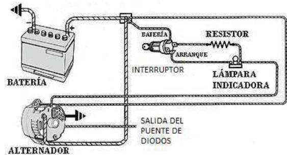
Fig. 4 Diagrama de Conexión
