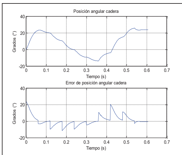
Fig. 9. Posición angular de salida y señal de error en la cadera
