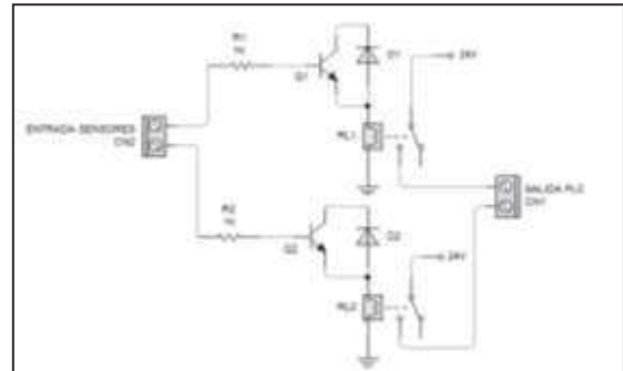
Fig. 5. Transducción de potencia.
