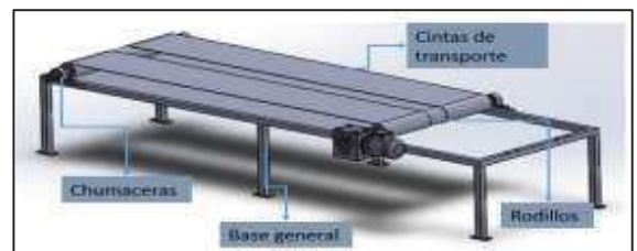
Figura 7. Propuesta del sistema de transporte
