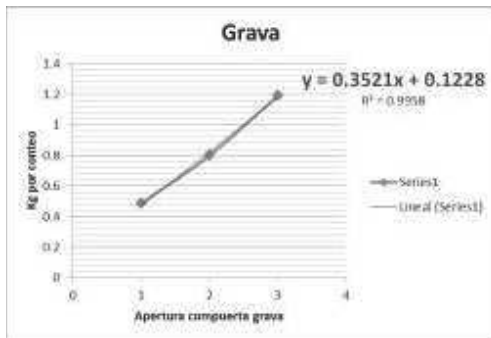
Figura 5. Gráfica de kg de grava por apertura de compuerta
