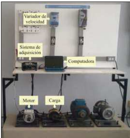
Fig. 2. Puesta del experimento.
