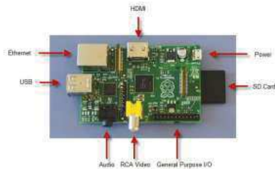
Figura 2. Placa base de la Raspberry Pi. Con flechas se indica la ubicación y nombre de los principales periféricos.
