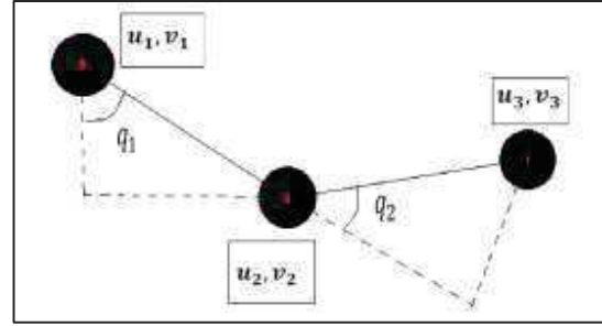
Fig. 4. Ilustración de los marcadores ubicados en el robot manipulador, donde los puntos en rojo determinan las coordenadas en píxeles determinados por el algoritmo.
