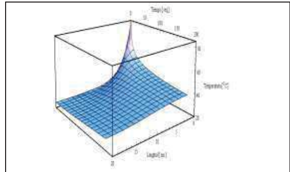
Fig. 2. Representación tridimensional de la evolución del calor en la barra.
