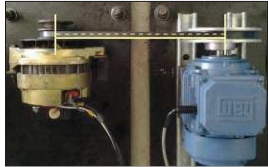
Fig. 3. Motor Alineado (estado sano).
