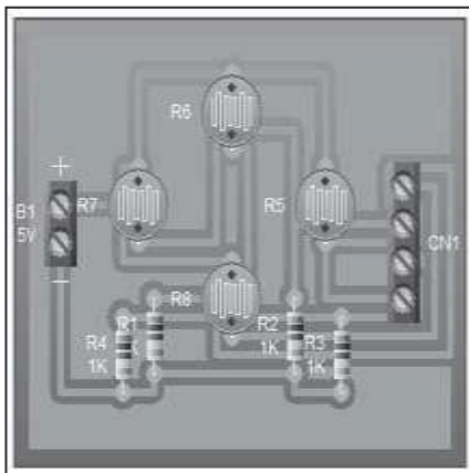
Fig. 4. Estructura física de los sensores.
