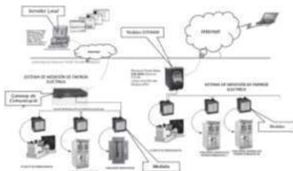
Fig. 2 Ejemplo de sistema de medición de la energía eléctrica
