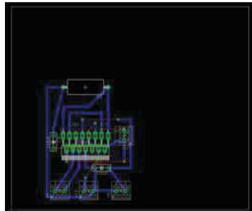
Fig. 5. Circuito dibujado en Eagle 6.4.0.
