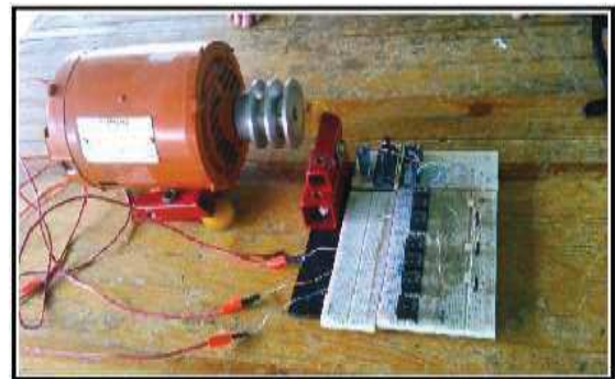
Fig. 11 Motor trifásico marca siemens con el sistema de freno.
