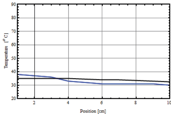
Fig. 10. Medición Temperatura Final.
