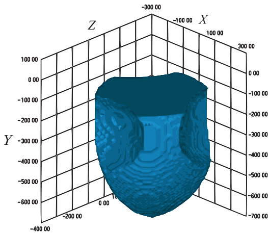
Fig. 5. Visualización 3D del espacio global de trabajo bajo la estrategia de reconfiguración basada en la variación simultánea de R_1 y H .
