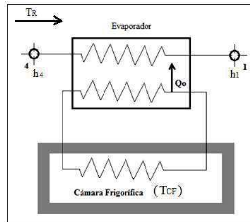
Fig.5. Diagrama esquemático del evaporador.
