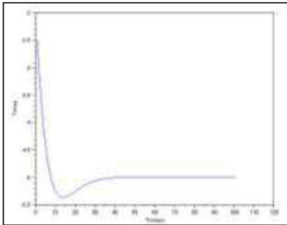
Fig. 2 PID sintonizado por ajuste de Zigler-Nichols
