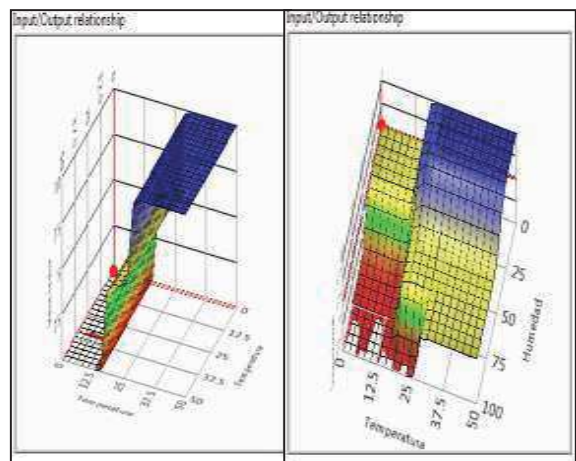
Fig. 4. Comportamiento del sistema para los actuadores del prototipo.
