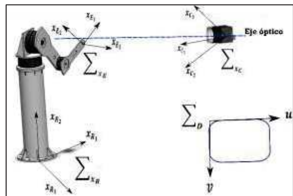
Fig. 1 Modelo de visión en configuración cámara fija
