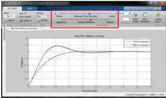
Fig. 6 Ventana de auto sintonía para el PID Controller.
