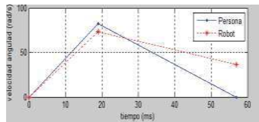
Figura 10 Comparación velocidad 2 (velocidad media).
