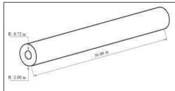
Figura 5. Dimensiones del cañón.
