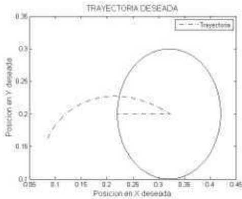
Figura 2. Trayectoria Deseada
