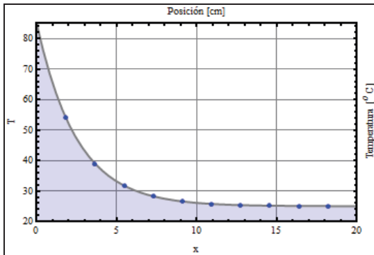
Fig. 1. Distribución de Temperatura Inicial para F_0(x) .
