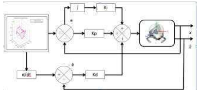
Fig. 3. Diagrama de bloques del controlador.
