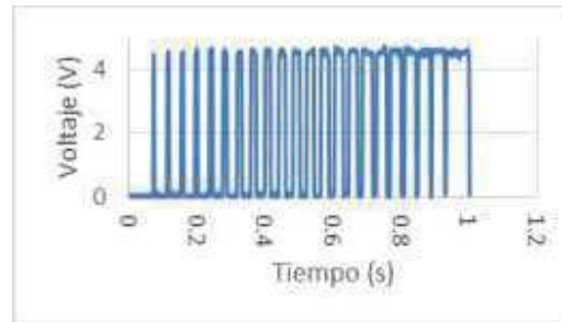
Fig. 7 Variación de ancho de pulso respecto a una función no lineal tipo exponencial.
