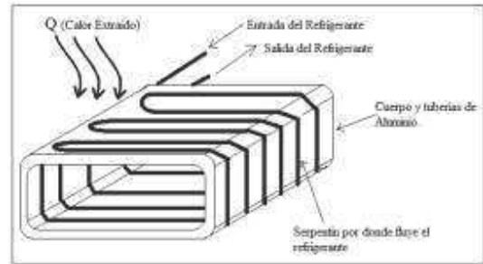
Fig. 2. Intercambiador de calor tipo evaporativo
