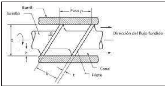
Figura 4. Geometría del tornillo
