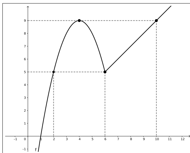
Figura 11.21: Gráfico da função f
