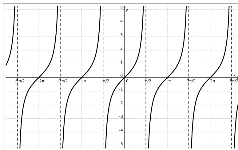
Figura 13.3: Gráfico da função f(x) = \tan(x)
