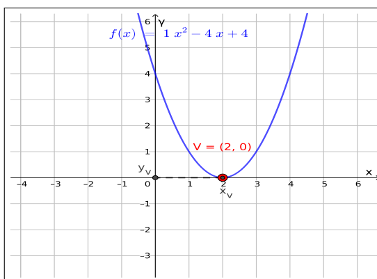
Figura 11.6: Gráfico da função f(x) = x^2 - 4x + 4
