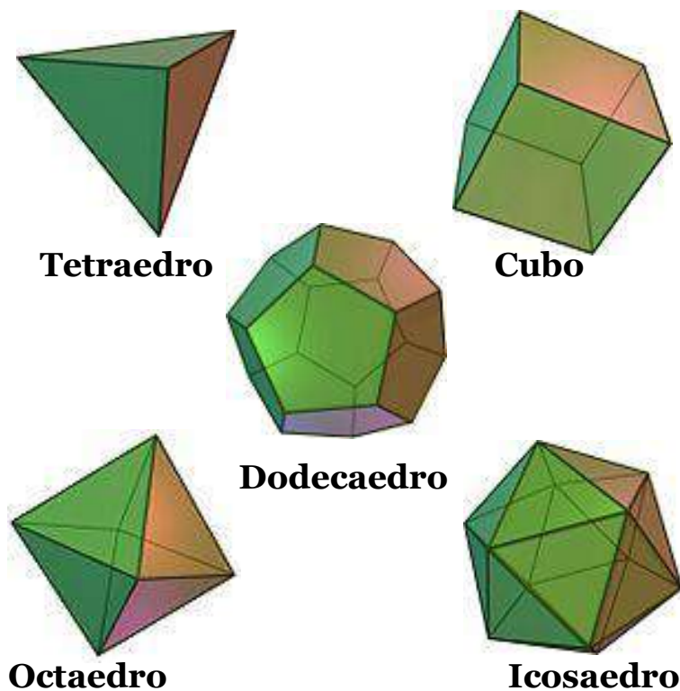
Figura 10. Poliedros regulares.
