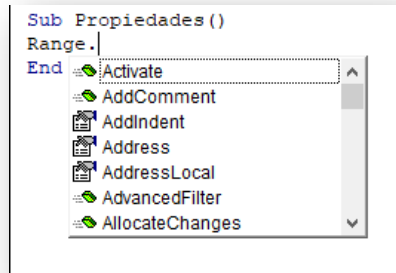
Figura 4.16. Si bien se muestran en la misma lista las propiedades y métodos de un objeto, éstos se distinguen entre sí por sus iconos correspondientes.
