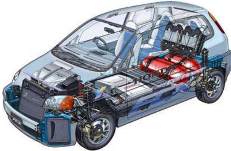
Disposición interna de un vehículo Honda a hidrógeno
