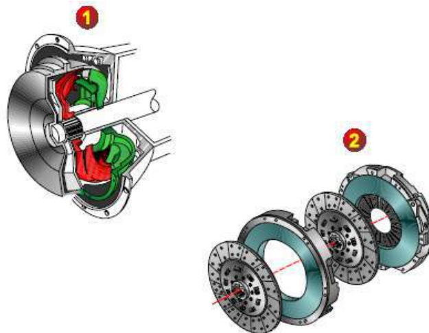
(1) Embrague hidráulico
