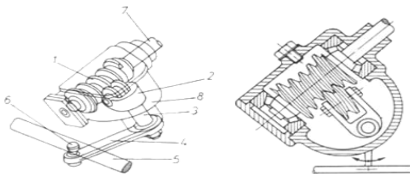
Sinfin globoidal y rodillo
