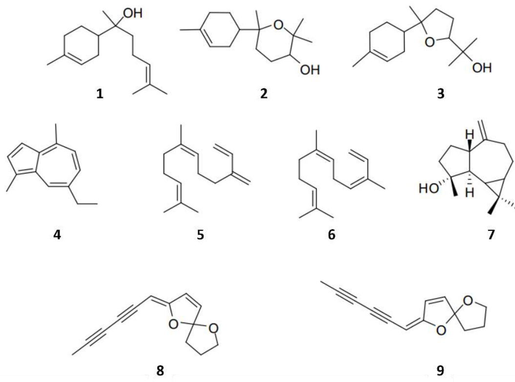
Figura 3. Principais constituintes da camomila. \alpha -bisabolol (1); \alpha -bisabolol A (2); \alpha -bisabolol B (3); Camazuleno (4); Farnesenos \alpha (5) e \beta (6); Epatulenol (7) e Espiroéteres Z (8) e E (9) (Adaptado de Oliveira, 2012).
