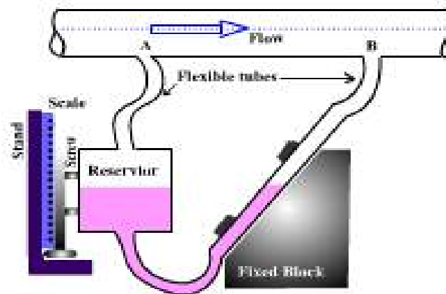
Fig. L-8.6: Micro manometer
