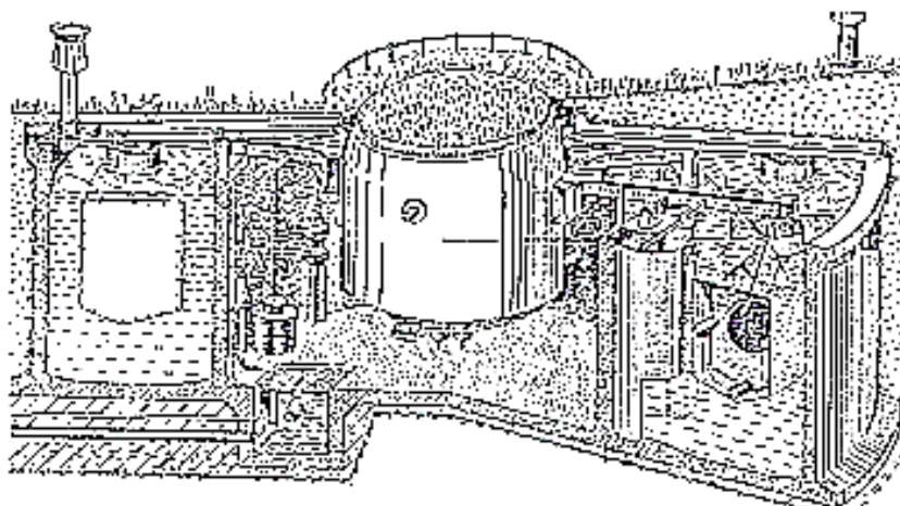
Fig. 5.5 - Lisímetro
