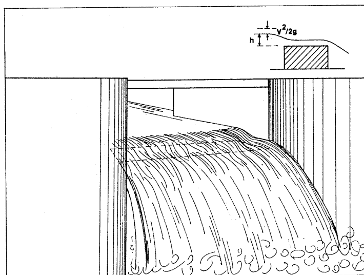
b) SOLEIRA ESPESSA
