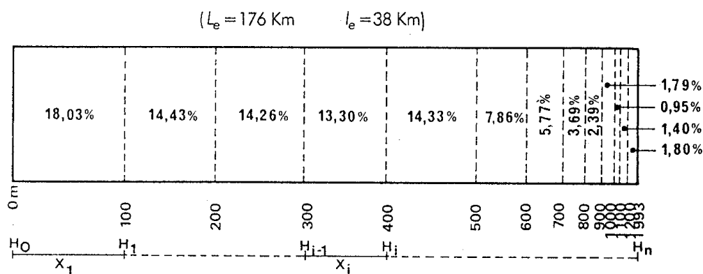
Fig. 2.7 Rectângulo equivalente da bacia do Mondego (Lencastre, 1984)
