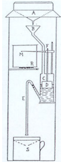
Fig. 3.6 - Udógrafo de bóia e sifão
