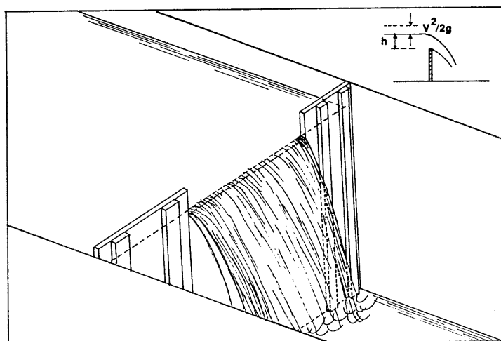
a) SOLEIRA DELGADA
