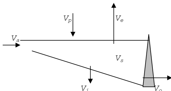
Fig. 5.4 - Esquematisação das variáveis intervenientes no balanço de uma albufeira
