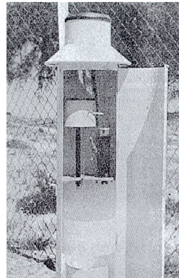
Fig. 3.6 - Udógrafo de bóia e sifão
