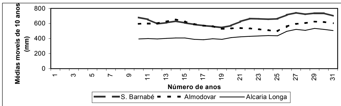
Fig. 3.18 - Média móveis
