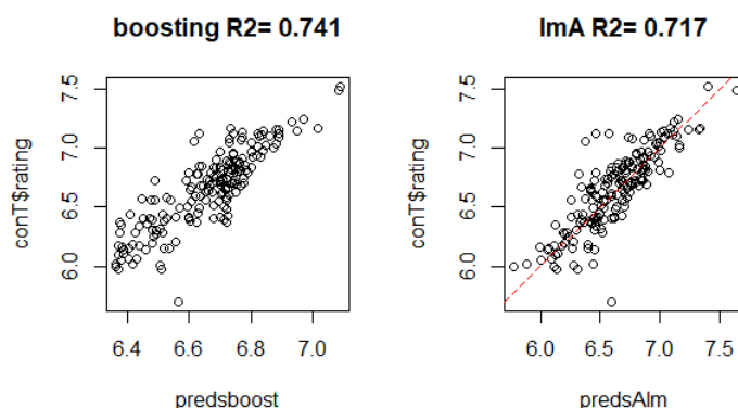
Figura 4.6: Comparación entre boosting y regresión.
