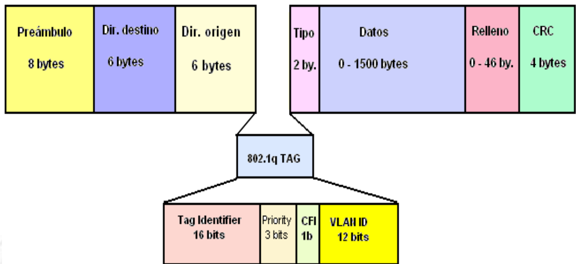
Imagen 4 (Formato de una trama 802.1q)
