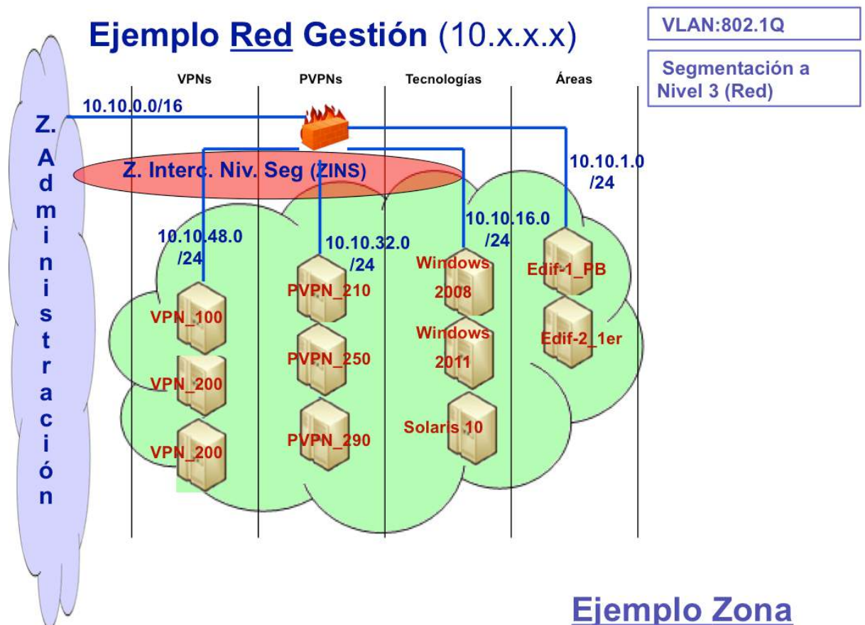
Imagen ejemplo de una red segmentada y de VLANs
