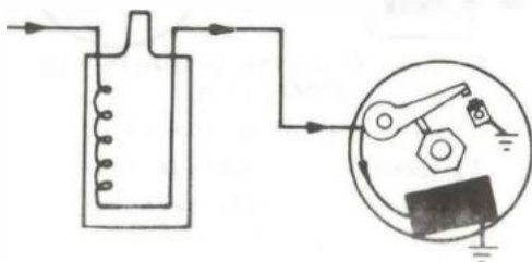
Fig. 27 Circuito primario con condensador.
