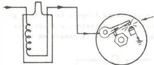
Fig. 25 Circuito primario sin condensador.
