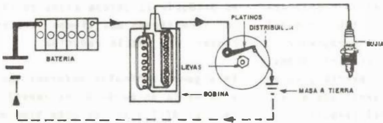
Fig. 22 Circuito Primario
