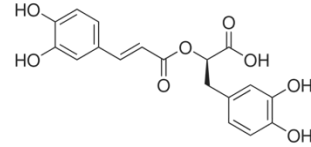
Figura 12 – Ácido Rosmarínico
