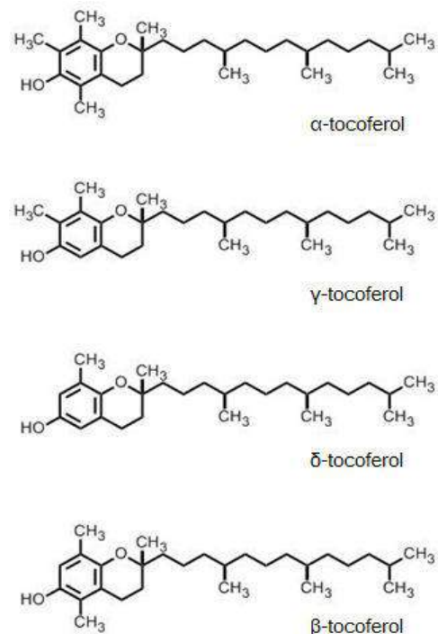
Figura 27 – Tocoferóis (Bender, 2009).
