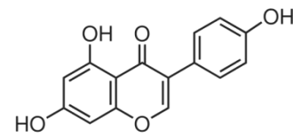
Figura 25 - Genisteína
