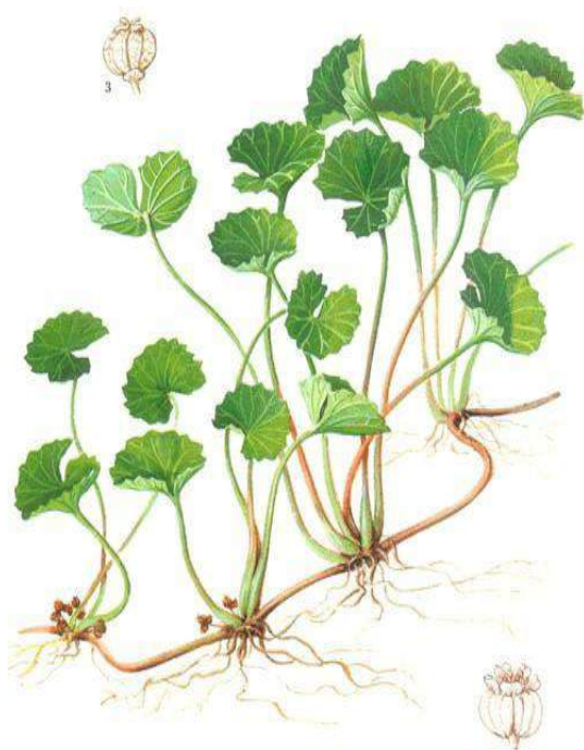
Figura 43 – C. asiatica
