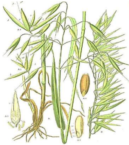
Figura 40 – A. sativa
