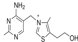
Figura 30 – Tiamina
