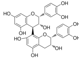
Figura 14 – Procianidina B-2
