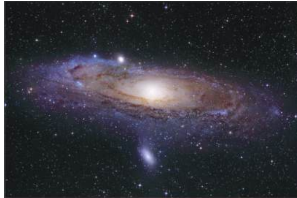
Figura 5.18. Galáxia vizinha de Andrômeda. Crédito: Robert Gender
