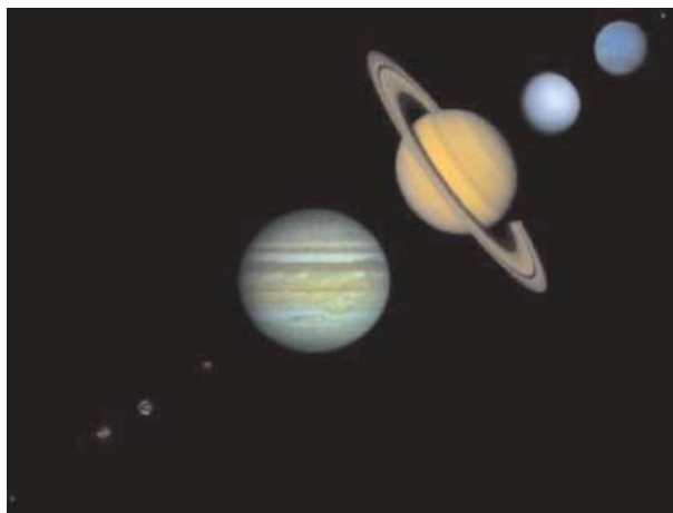
Figura 6.4. Sistema Solar: planetas na escala de tamanho
