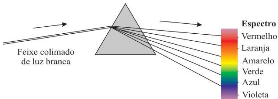
Figura 5.1. Espectroscópio com prisma
