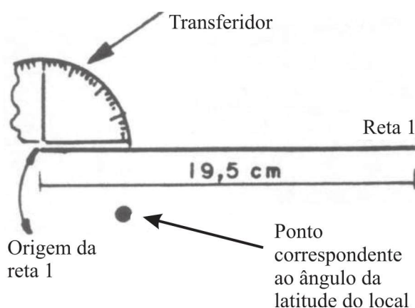
Figura 3.19. Determinação do ângulo correspondente à latitude local
