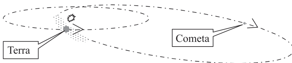
Figura 5.9 (fora de escala). A Terra e um cometa orbitam ao redor do Sol. Do cometa desprendem-se fragmentos quando ele se aproxima do Sol. Enxames de fragmentos podem ficar vagando nas proximidades da órbita percorrida pelo cometa. A Figura mostra o instante em que a Terra cruza um desses enxames
