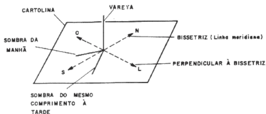
Figura 3.16. Determinação dos pontos cardeais
