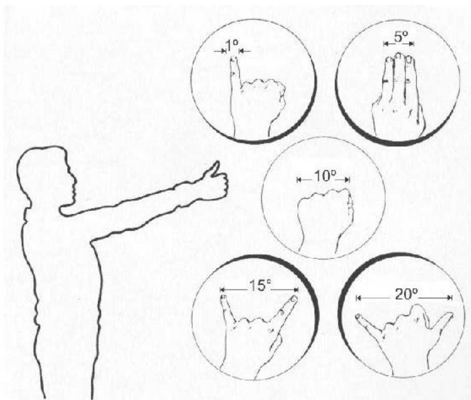
Figura 1.14. Método simples para medição de ângulos no céu
