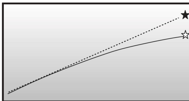
Figura 1.9. As camadas mais densas da atmosfera, nas quais o encurvamento dos raios de luz é mais pronunciado, ficam mais perto do solo. A estrela branca está na posição verdadeira. Mas o observador tem a impressão de que ela se encontra mais elevada, na posição da estrela preta. Para o observador a estrela parece estar na direção da tangente (linha tracejada) à trajetória da luz no local de observação
