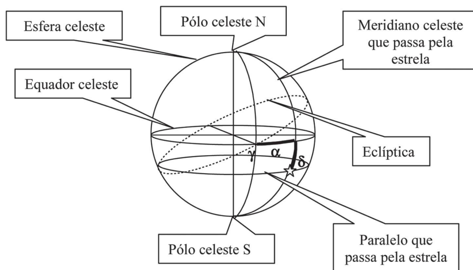
Figura 2.9. Sistema equatorial de coordenadas celestes. O plano fundamental é o equador. Com base nele define-se os pólos celestes. A posição de uma estrela é especificada pela declinação \delta e ascensão reta \alpha . A trajetória do Sol na esfera celeste é a eclíptica aqui representada apenas para definir a localização do ponto vernal \gamma
