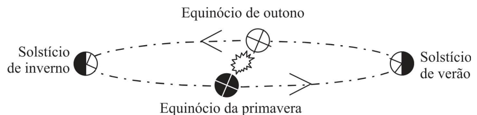
Figura 5.11 (fora de escala). A eclíptica, plano da órbita da Terra ao redor do Sol, fica mais elevada no céu para um observador do hemisfério sul às 06:00 h, no equinócio de outono
