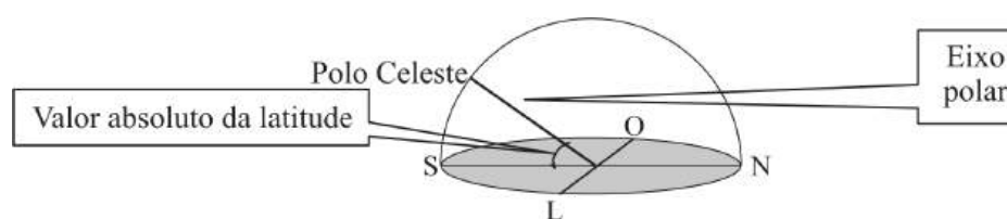
Figura 2.13. É mostrada a direção do pólo celeste sul
