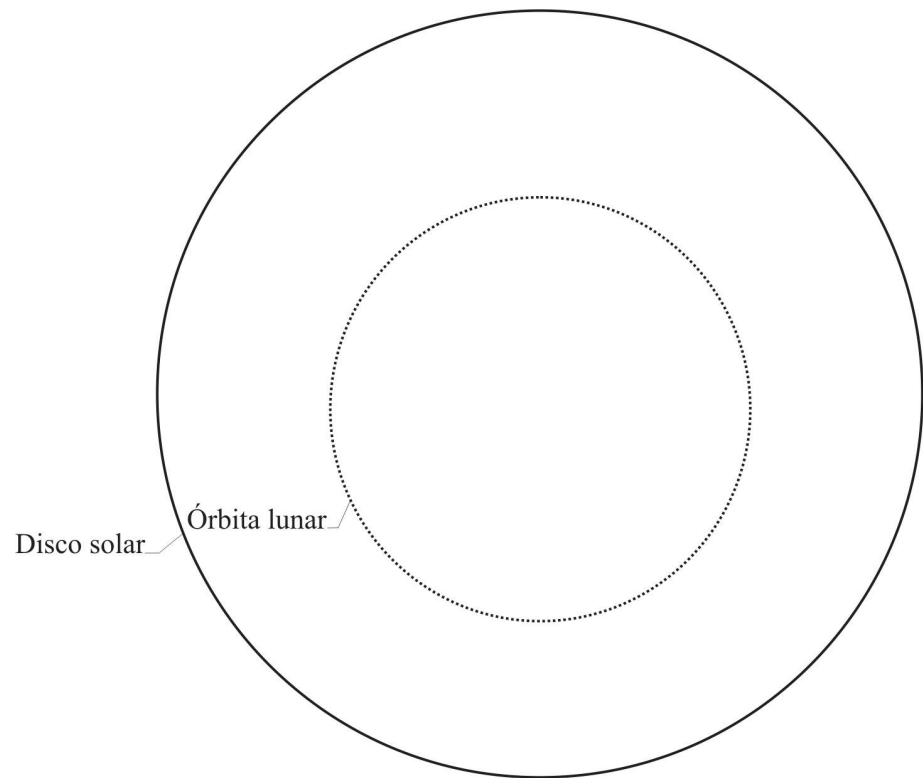
Figura 4.30. Esquema de como fica a atividade proposta com a inserção da órbita lunar dentro do disco solar
