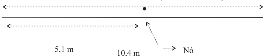
Figura 4.18. Esquema da posição do nó sobre o barbante usado para a construção da elipse do cometa Halley.
