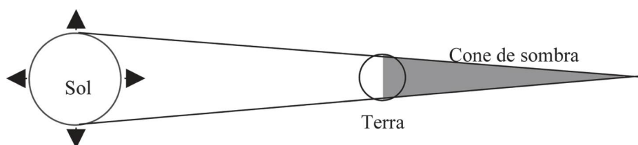
Figura 1.6 (fora de escala). A incidência dos raios solares ocorre só no hemisfério voltado para o Sol, ou diurno. O hemisfério oposto, ou noturno, se encontra no cone de sombra. Esse cone se forma porque a Terra é opaca e os raios solares se propagam em linha reta. Do interior desse cone não se pode observar o Sol
